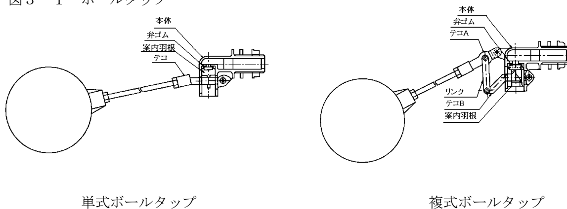
図3-1 ボールタップ
