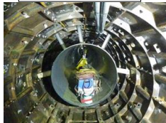
シールド内部（二次覆工）
