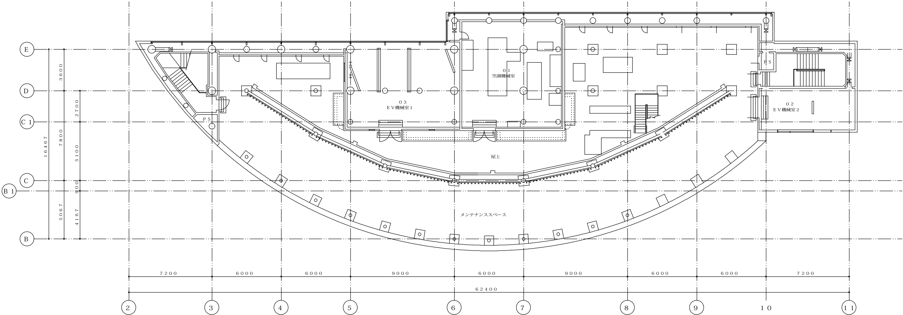
塔屋階平面図
