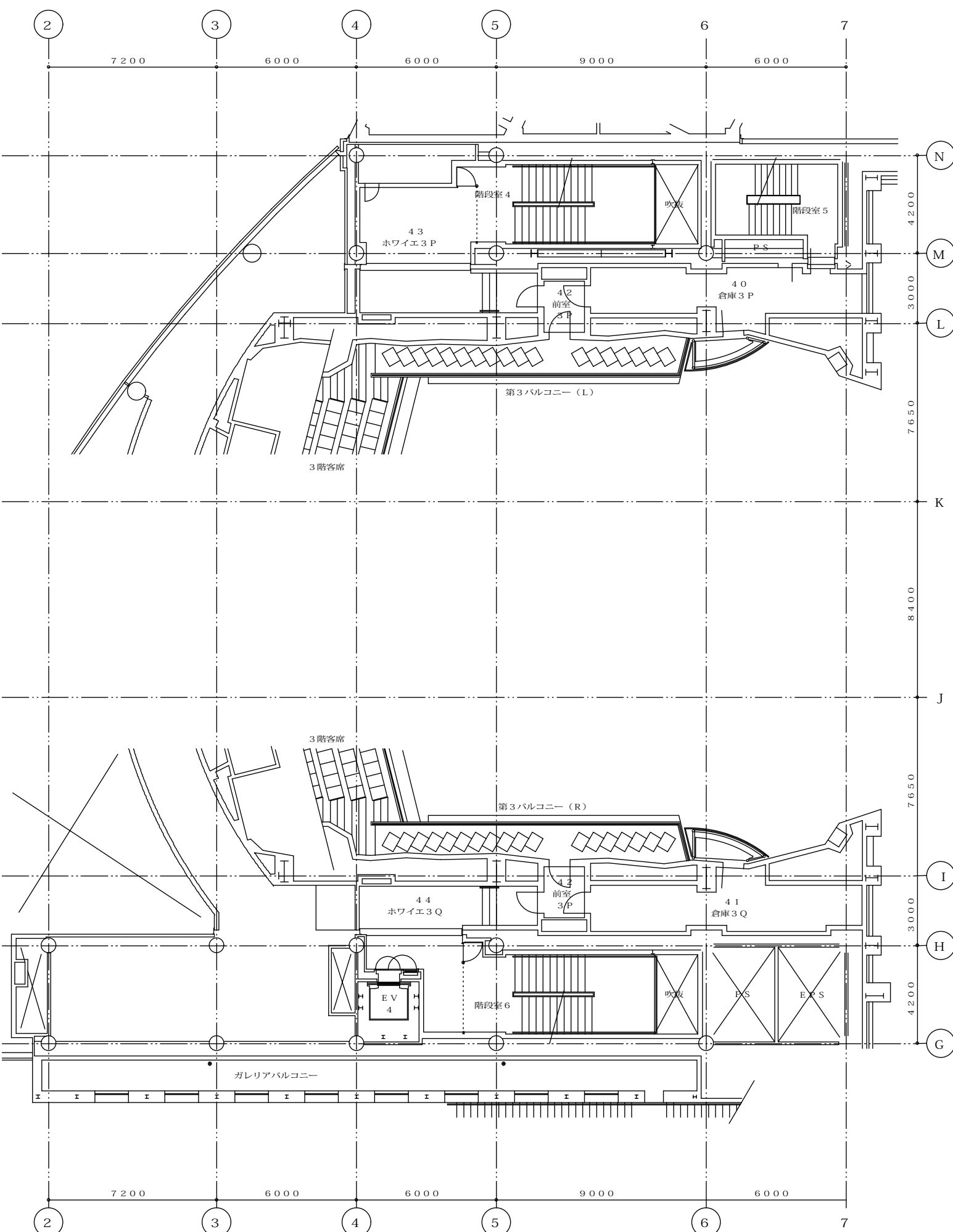
第3バルコニー平面図 1: 200
