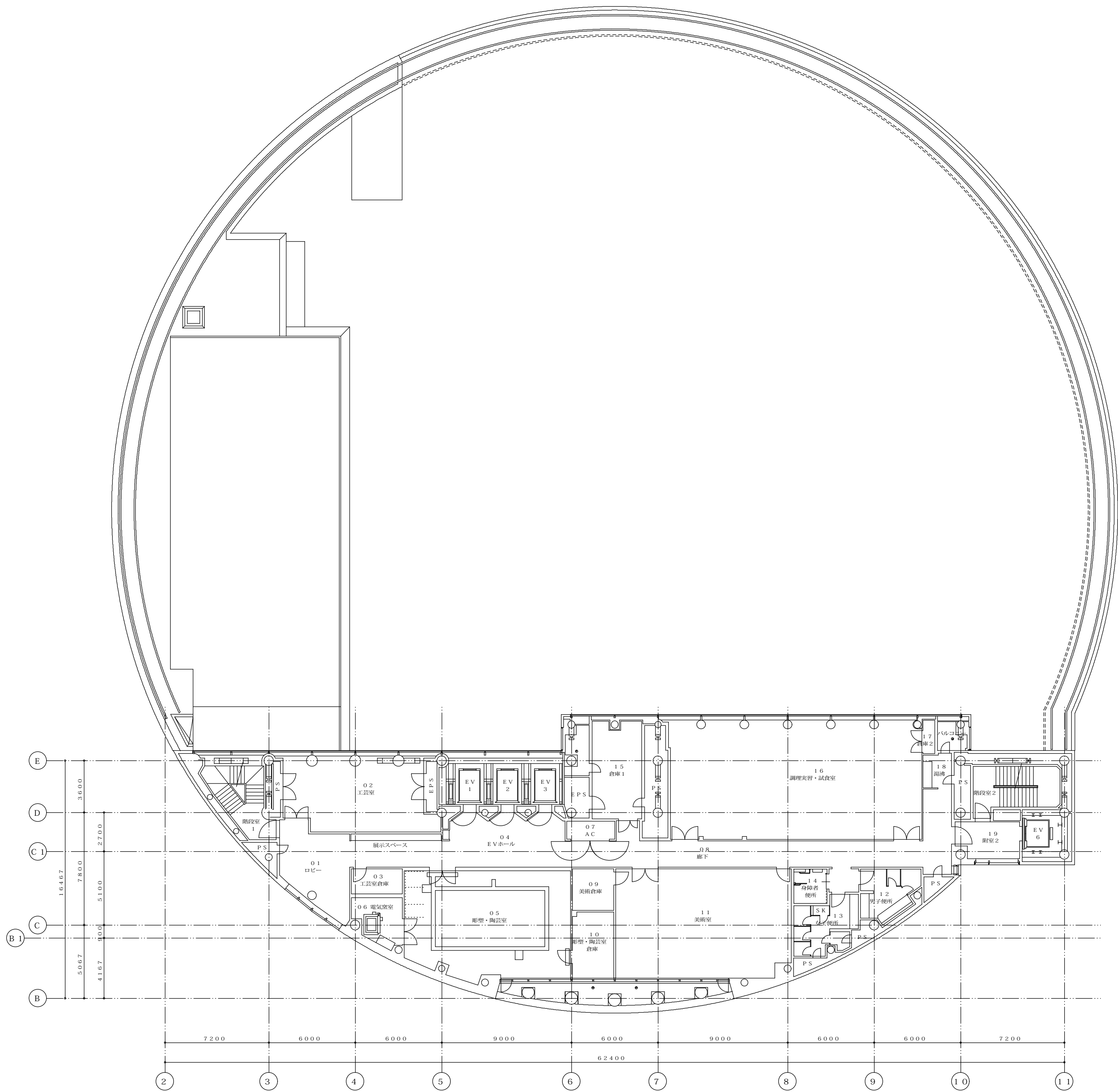
10階平面図
