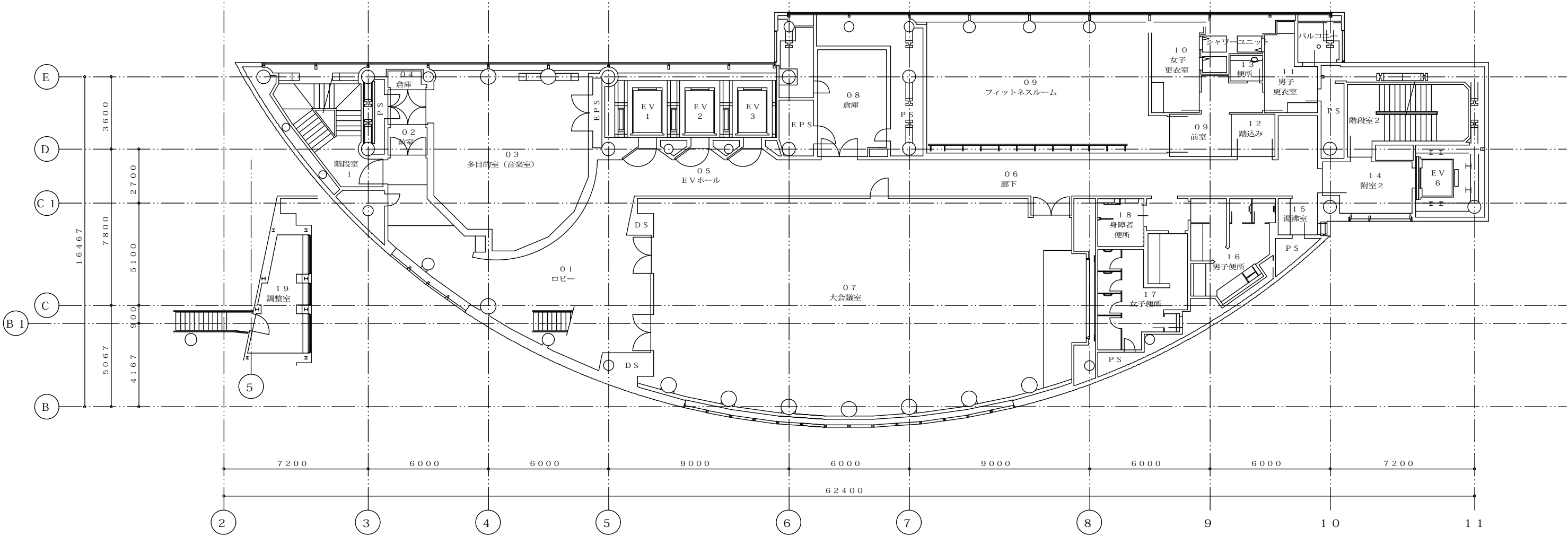
11階平面図
