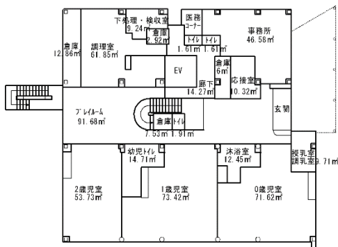
1階平面図
