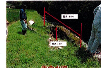
重倉水路 護岸復旧修繕
