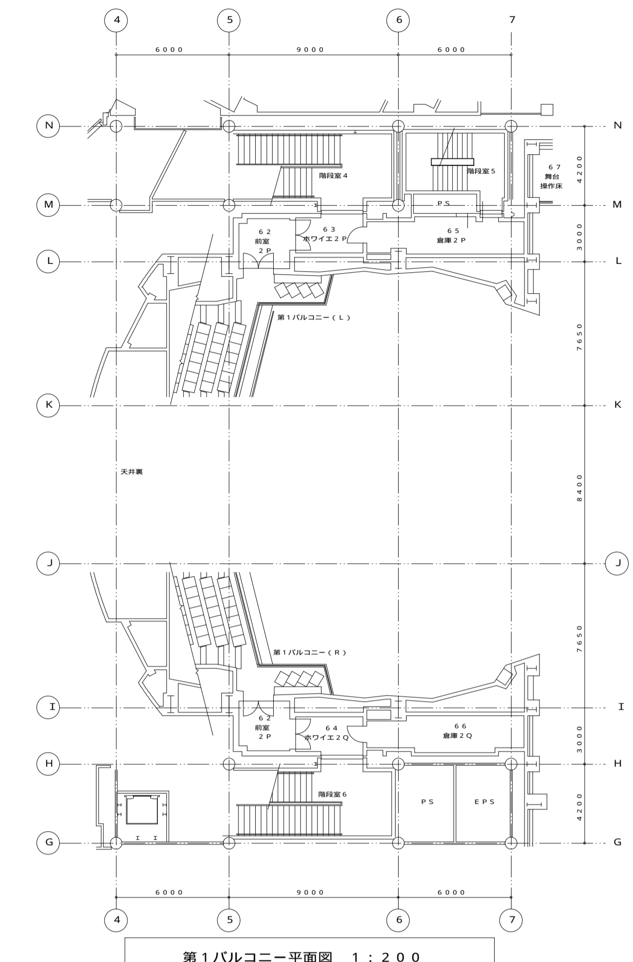
第1バルコニー平面図 1 : 200
