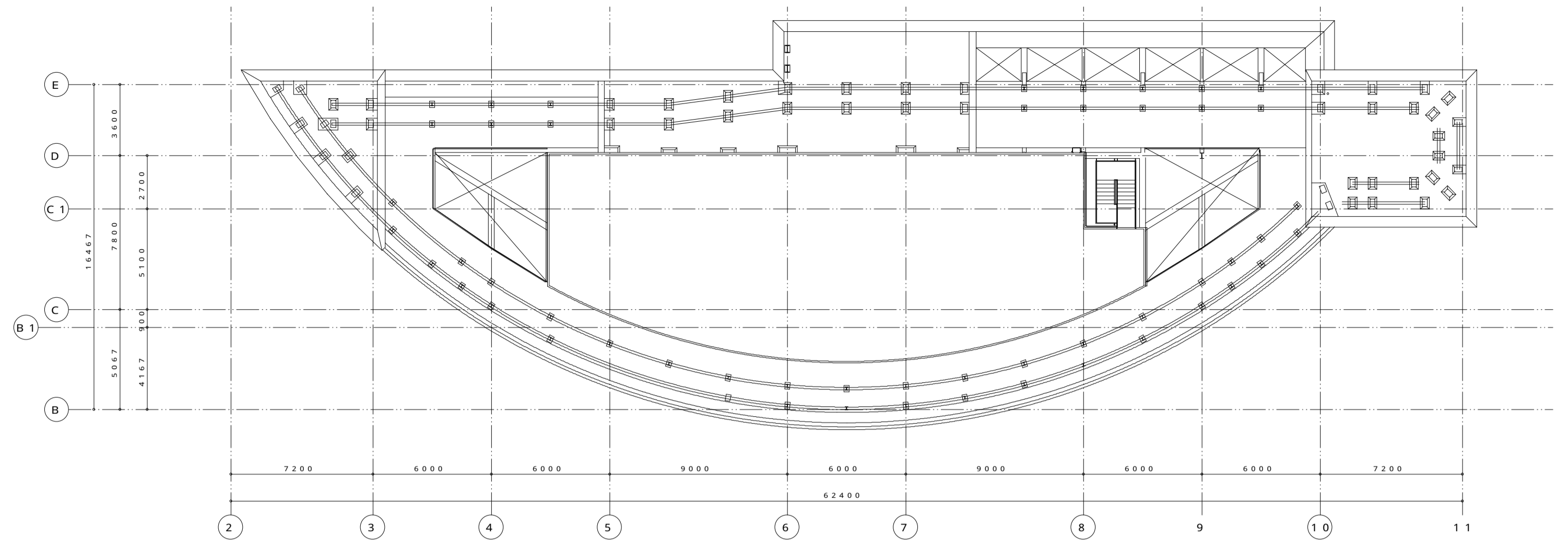
屋根伏図
