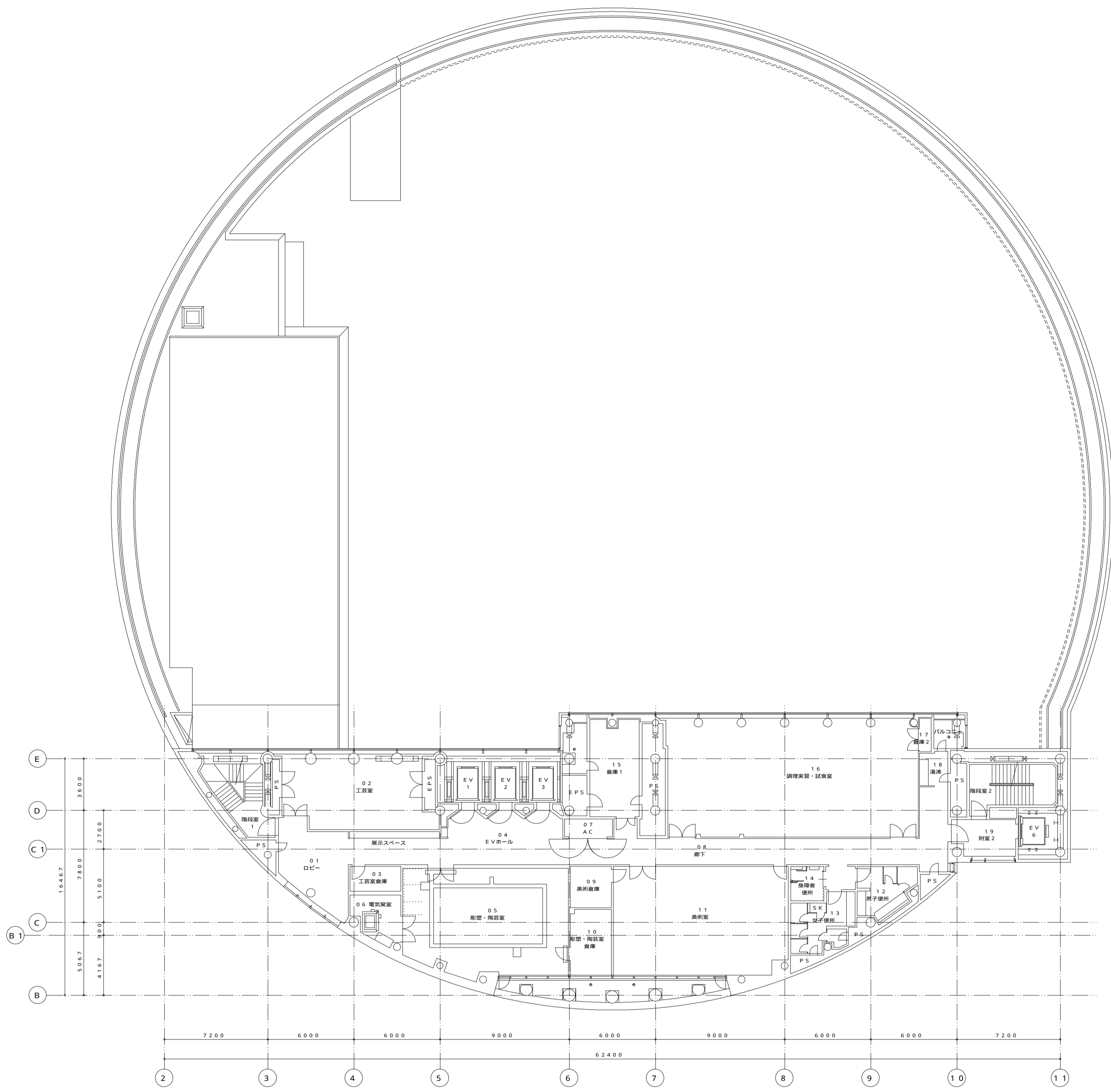
10階平面図
