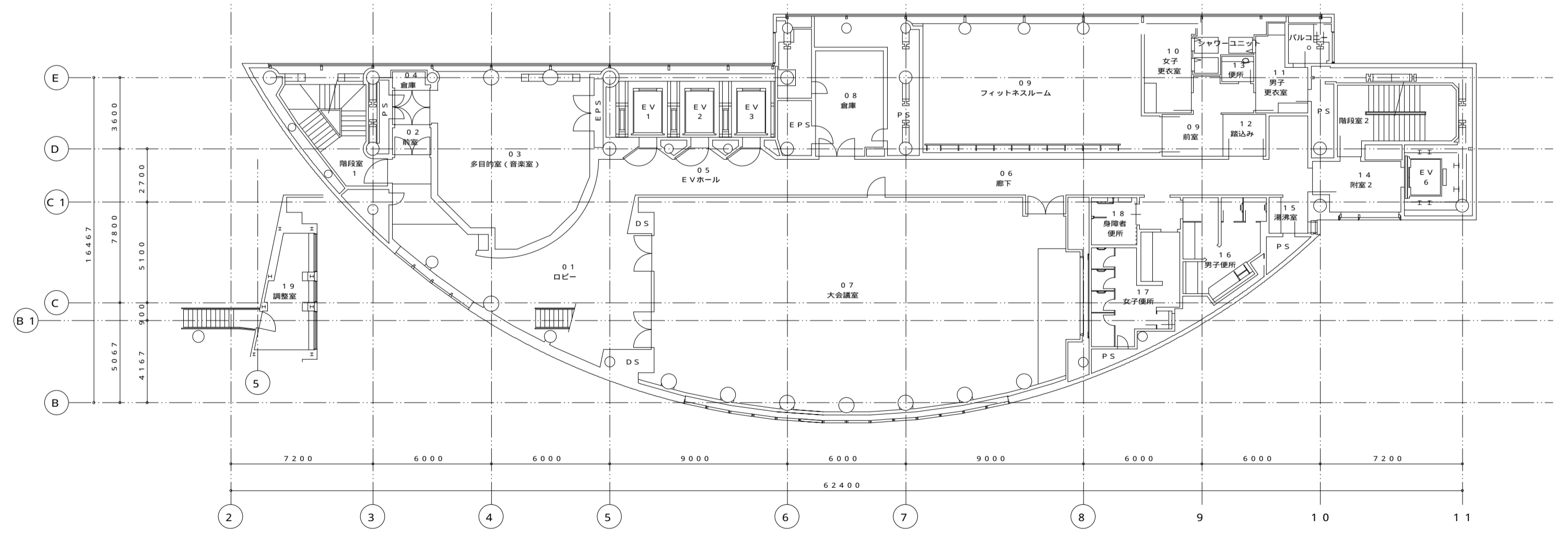
11階平面図
