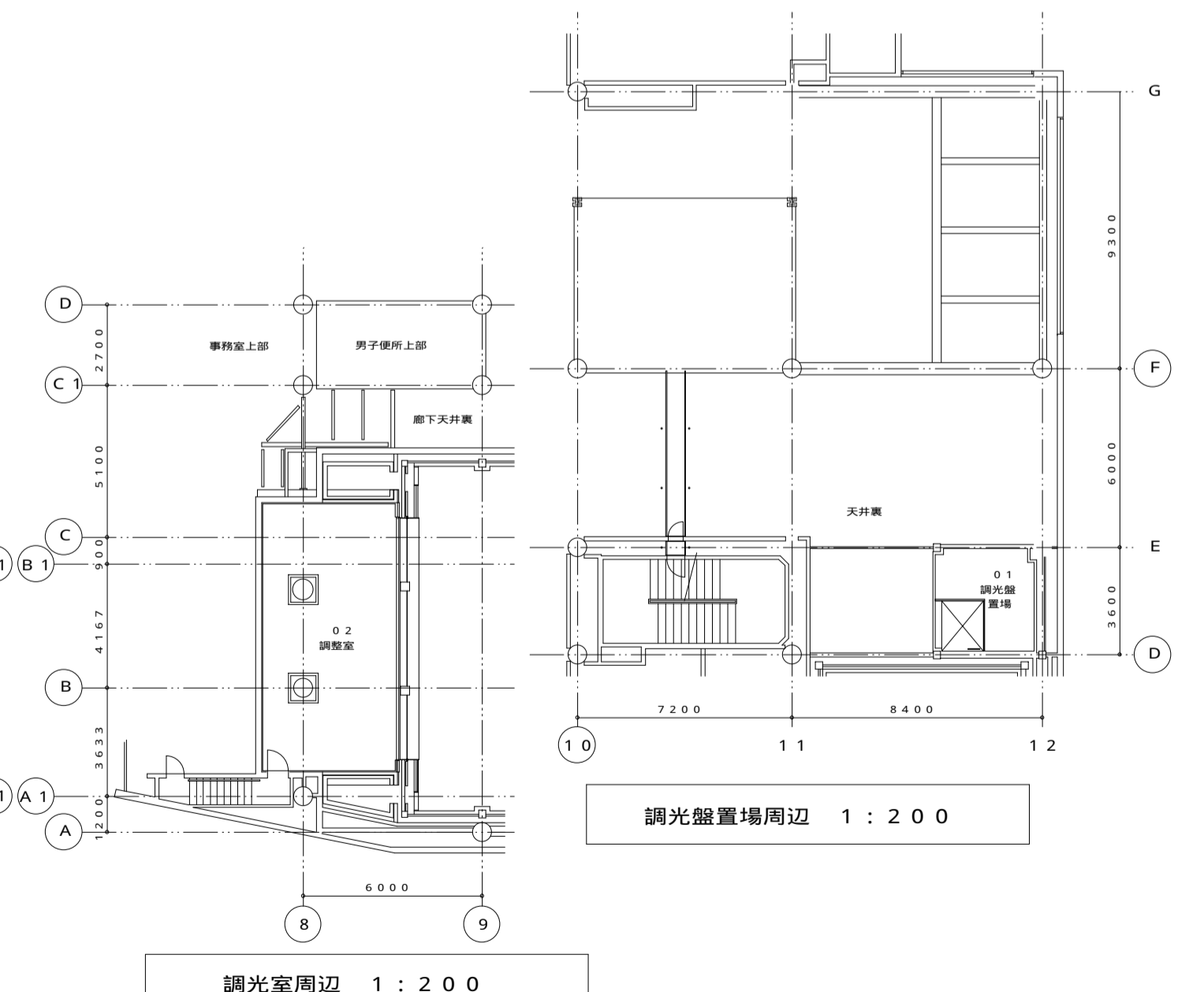
調光室周辺 1 : 200
