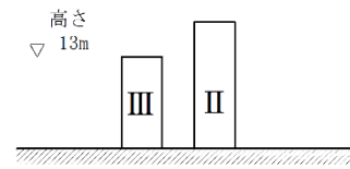
図. 1-2 地表面粗度区分(都市計画区域外)
