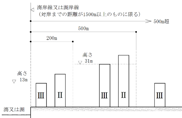
図. 1-1 地表面粗度区分(都市計画区域内)
