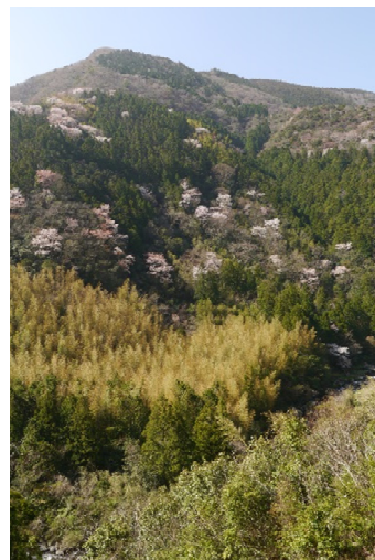
No23 狩山河内神社（イチイガシ）と吉原川（右の写真は吉原川沿いの山地斜面）
