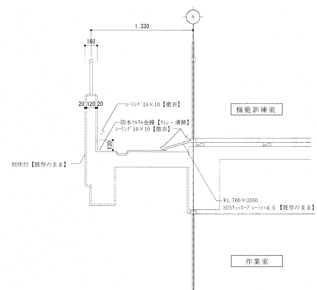
2 階断面詳細図 S=1/30
