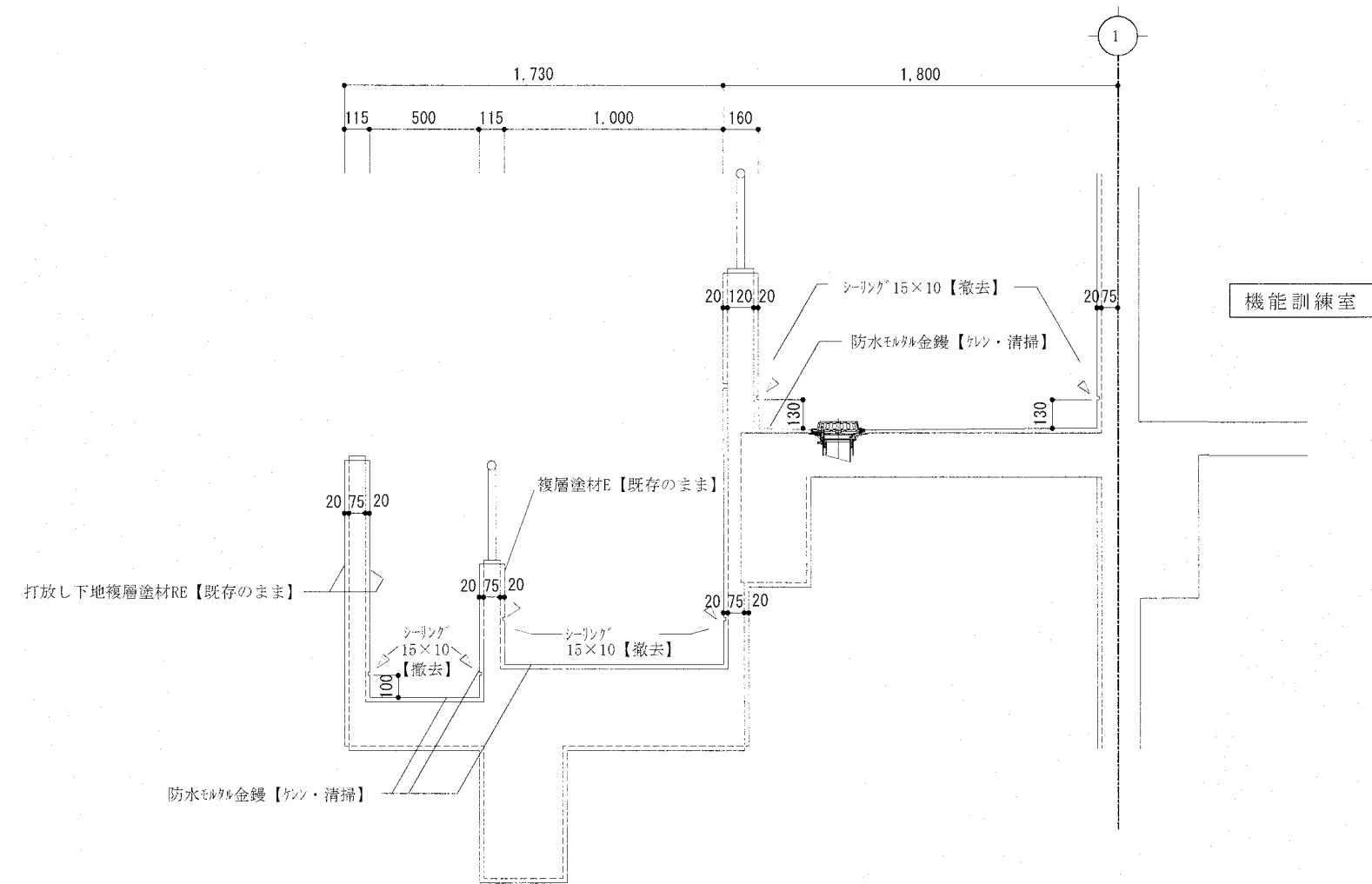
2階階段断面詳細図 S=1/30
