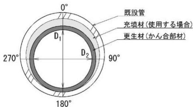
図 参 5-7-2 仕すり内径の測定位置(製管タイプ)
