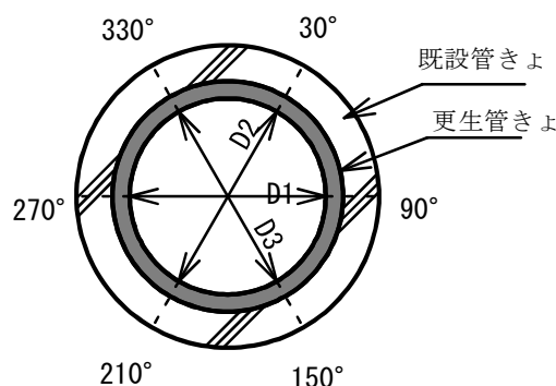
図 参 5-7-1 仕上り内径の測定位置(熱硬化タイプ、光硬化タイプ、熱形成タイプ)
