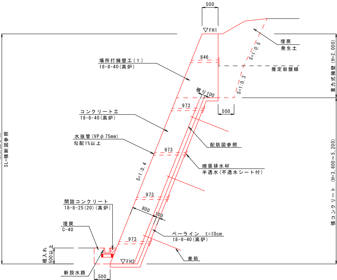
コンクリート擁壁構造図 S=1:50
