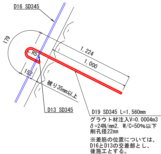
差筋構造図 S=1:20
