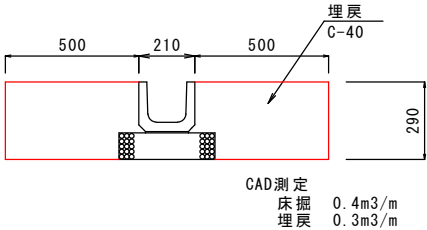
土工図 S=1:20 土工延長 L=1.4m (P0.0~P-1.4)
