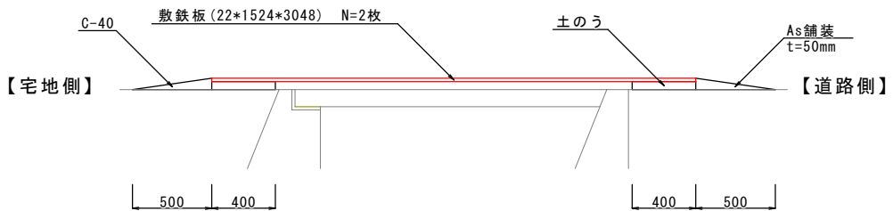
仮設道平面図 S=1:50
