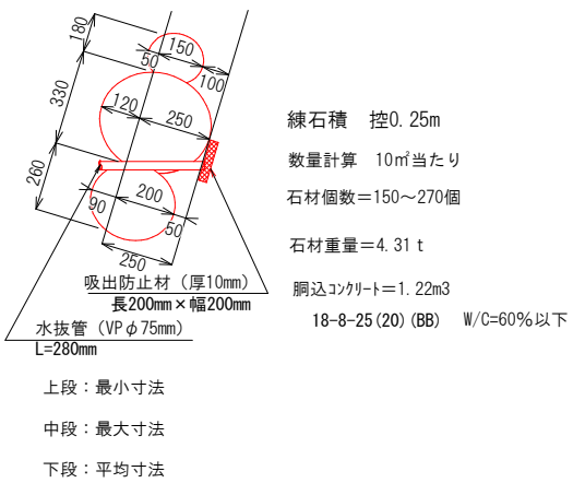
摺付工 S=1:20
