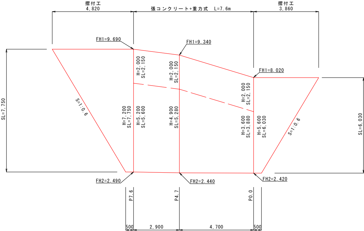
展開図 S=1:100
