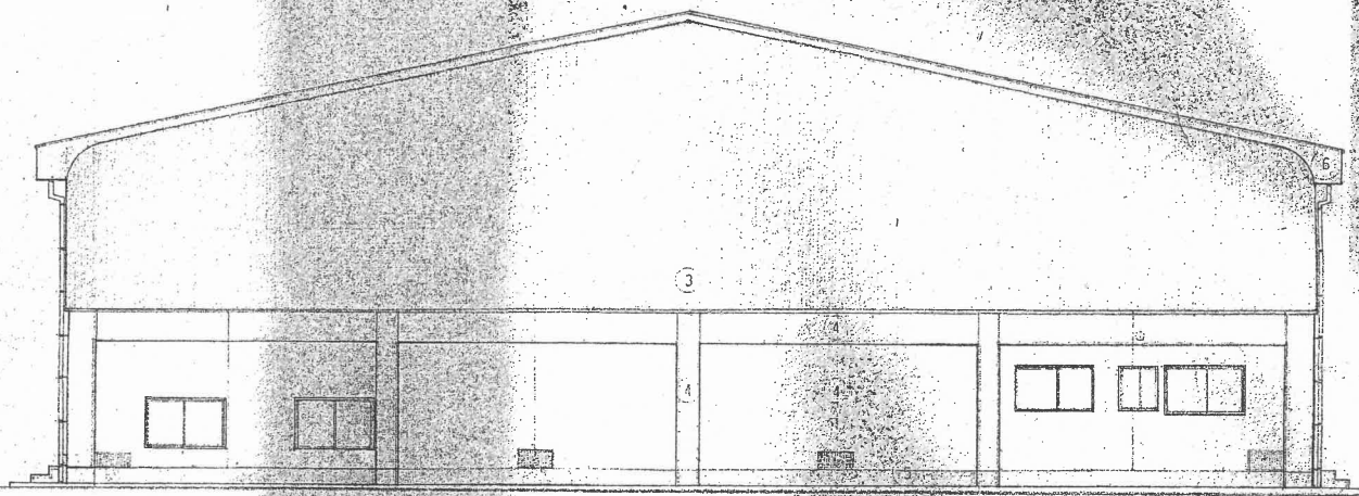
西面立面图 S=1:100
