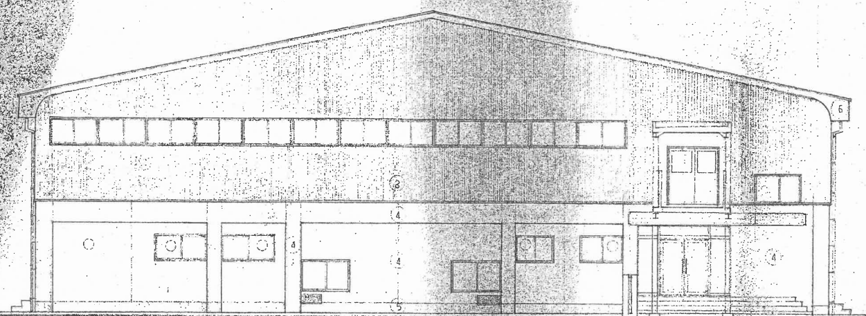
东面立面图 S=1:100
