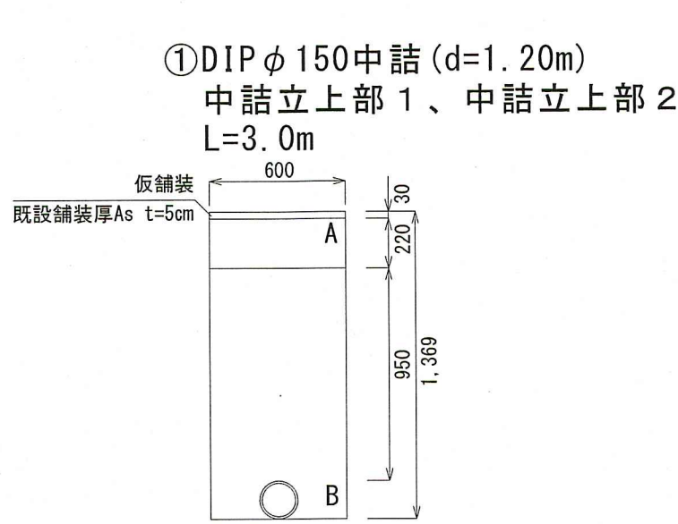
廃止管土工図 S=1:30
