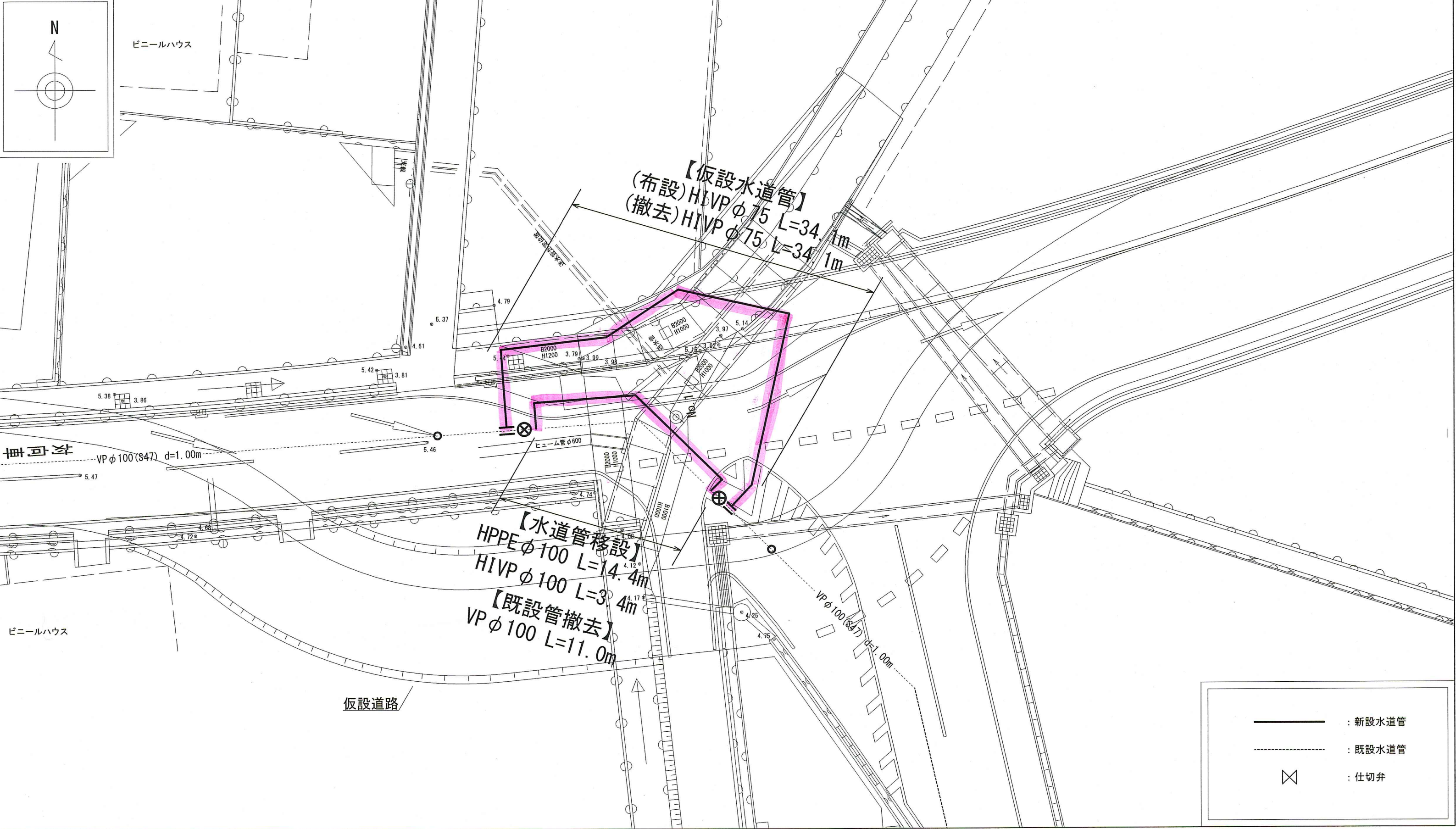
平面図 S=1:200
