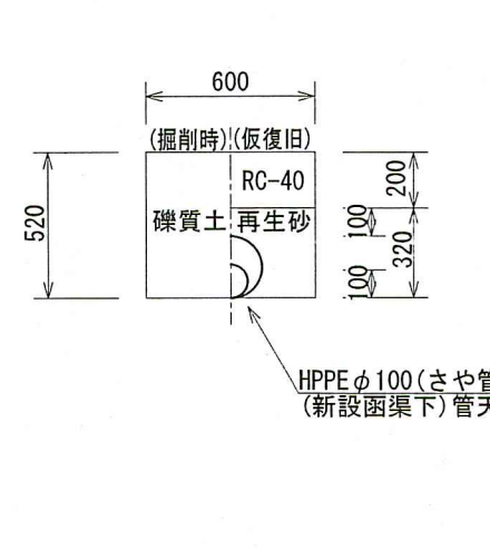
HPPE φ100 新設函渠下部 (県道車道部) L=3.0m
