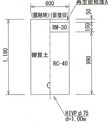
【仮設撤去】HIVP φ75 (d=1.00m) (県道車道部) L=12.7m
