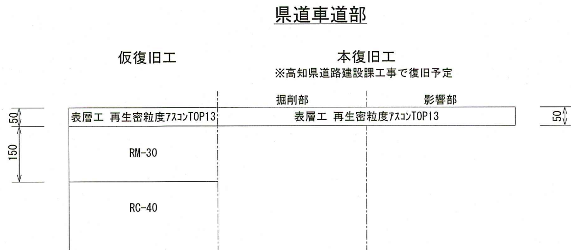
舗装復旧断面図 S=1:Free
