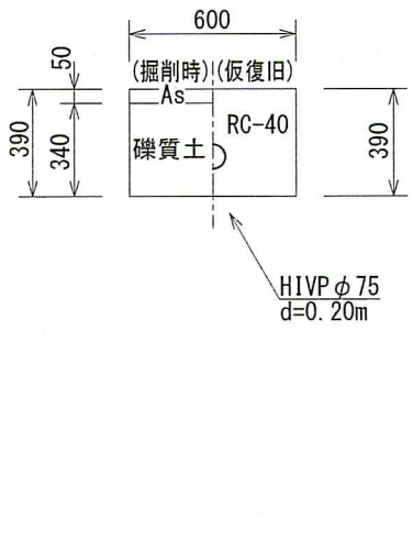
【仮設】HIVP φ75 (d=0.20m) (県道車道部) L=4.5m
