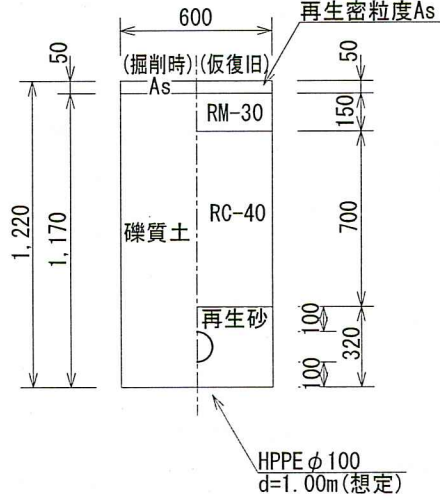
HPPE φ100 (d=1.00m) (県道車道部) L=3.0m
