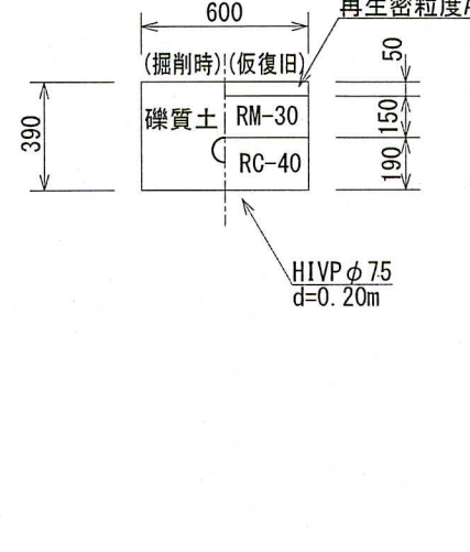
【仮設撤去】HIVP φ75 (d=0.20m) (県道車道部) L=4.5m
