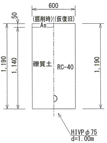
【仮設】HIVP φ75 (d=1.00m) (県道車道部) L=12.7m
