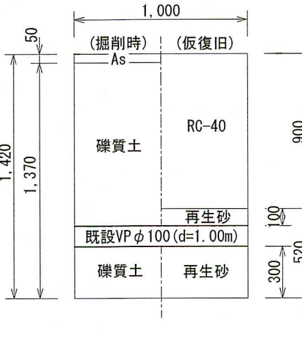
不連続分岐部 φ100 × φ75 (県道車道部) L= 2.5m × 2箇所
