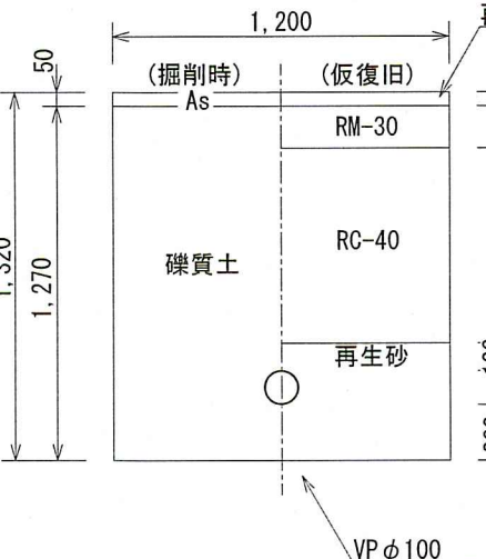
不連続簡易仕切弁部 φ100 (県道車道部) L= 1.5m × 2箇所
