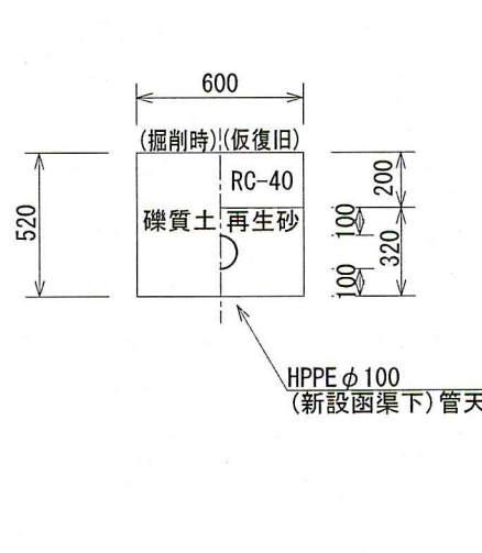
HPPE φ100 伏越し部 (県道車道部) L=3.0m
