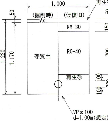
VP φ100 補強金具取付部 (d=1.00m) (県道車道部) L=12.0m
