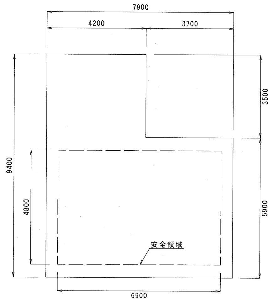
土舗装展開図 S=1:100
