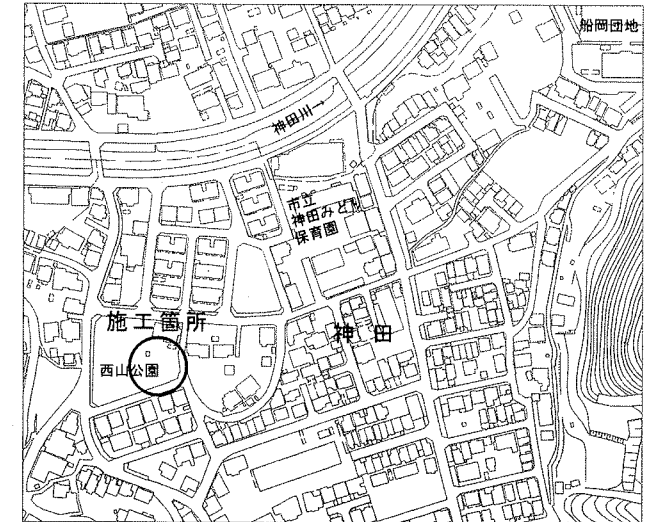
位置図 S=1:5000
