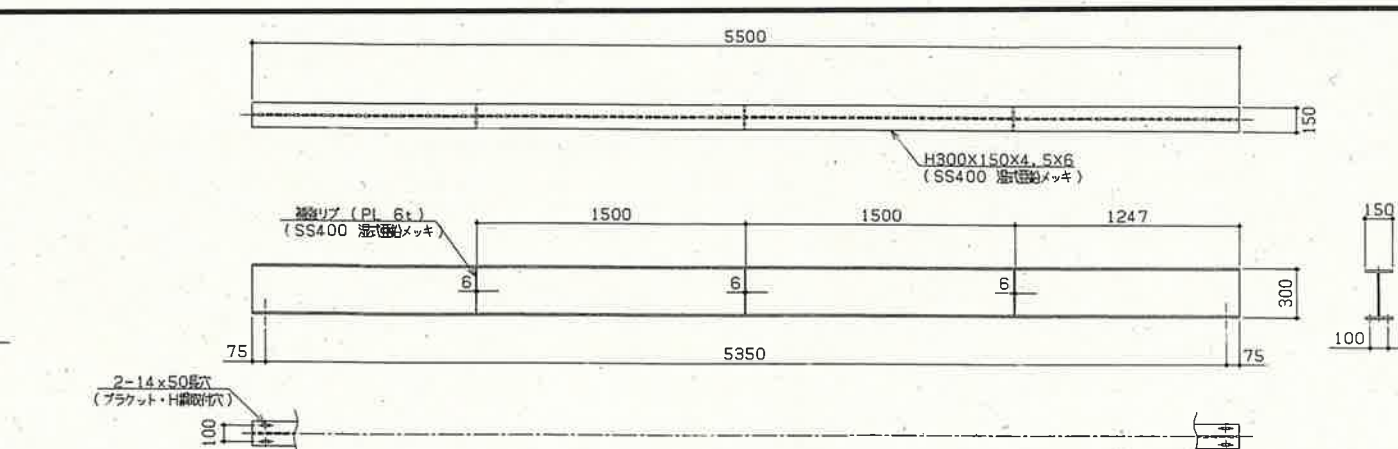
既設受桁④
