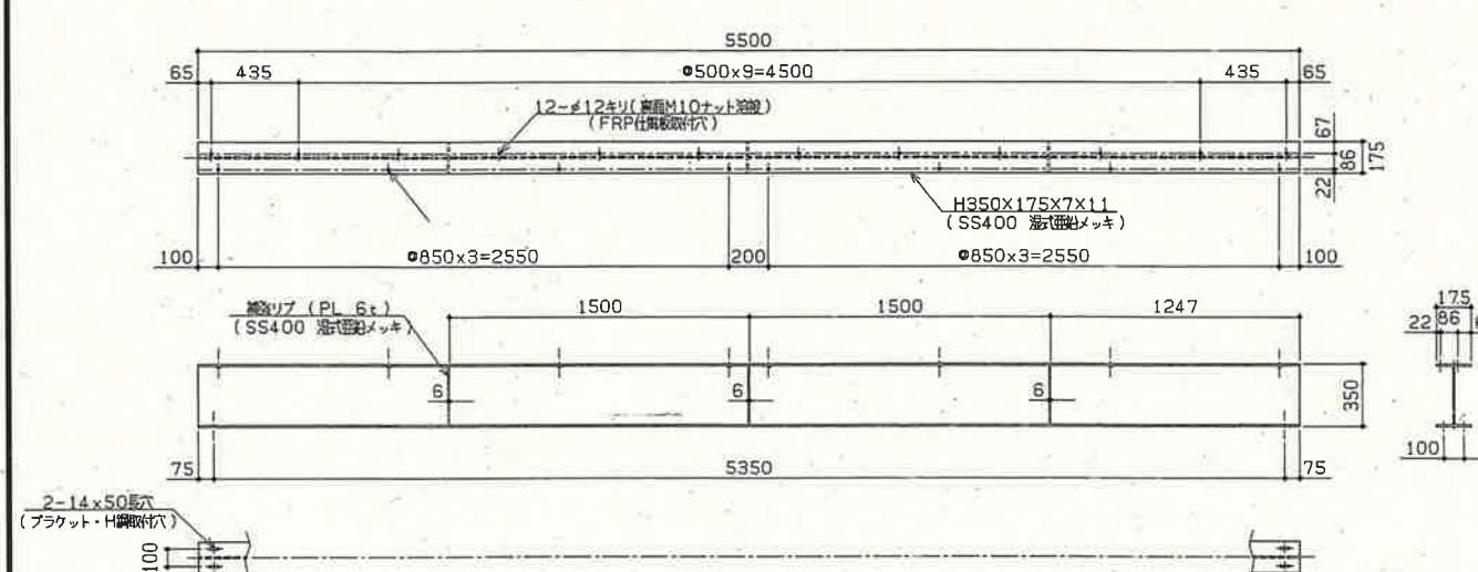
既設受桁②
