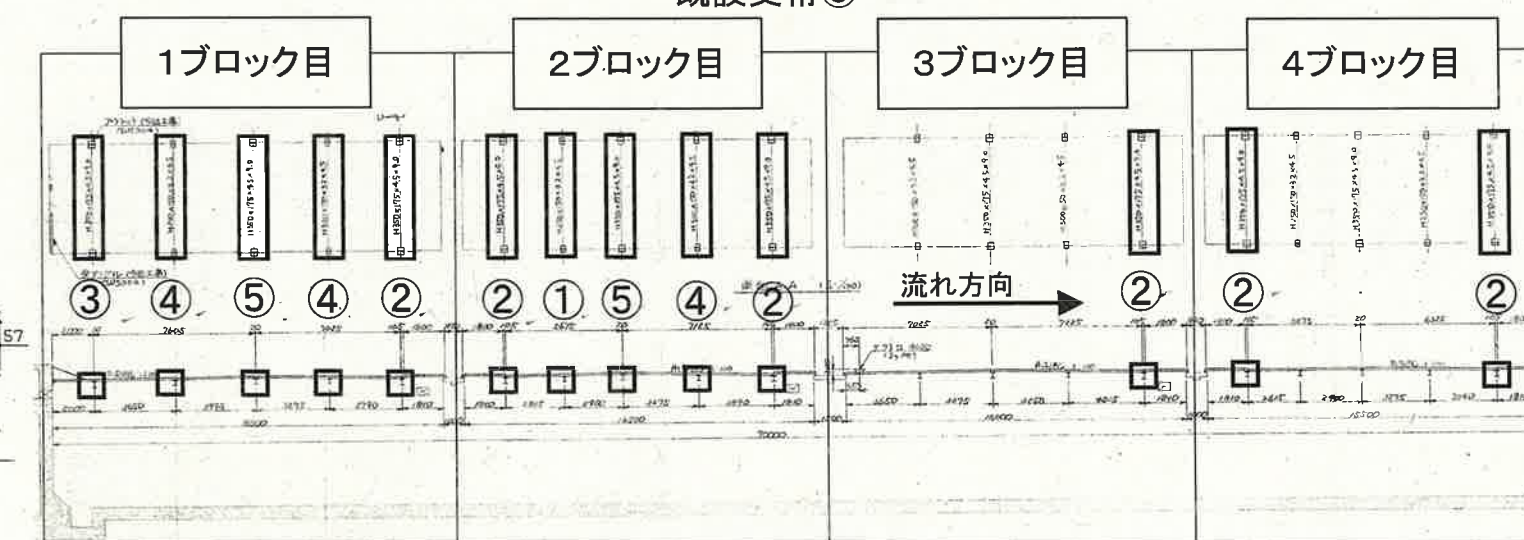
3系エアレーションタンク受桁配置図
