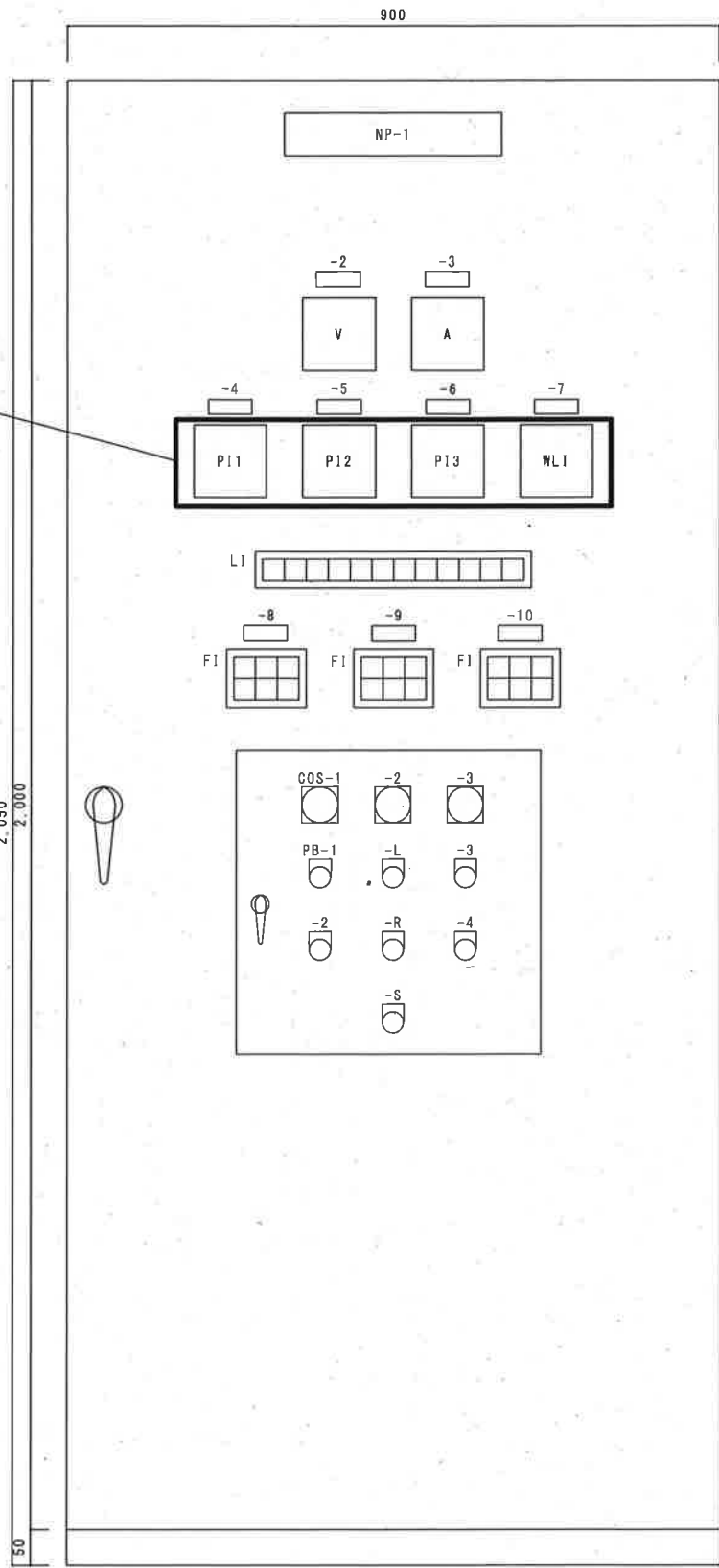
正面図
