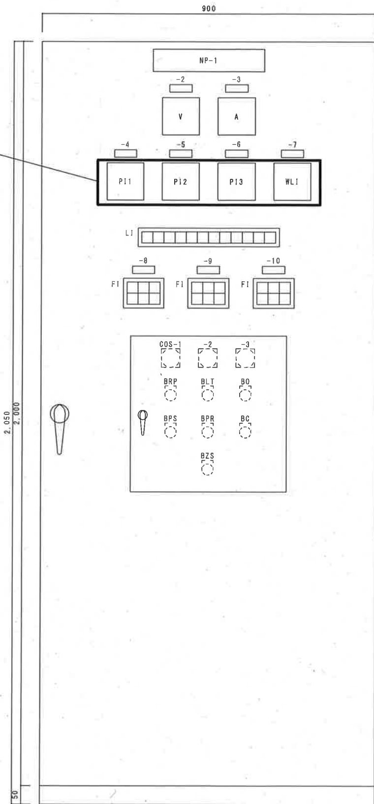
正面図
