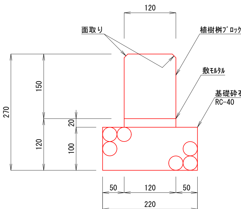
【植樹柵ブロック(共通)】 S=1:5
