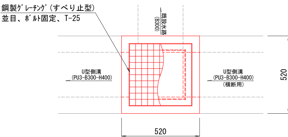
3号集水樹 (口300×300)
