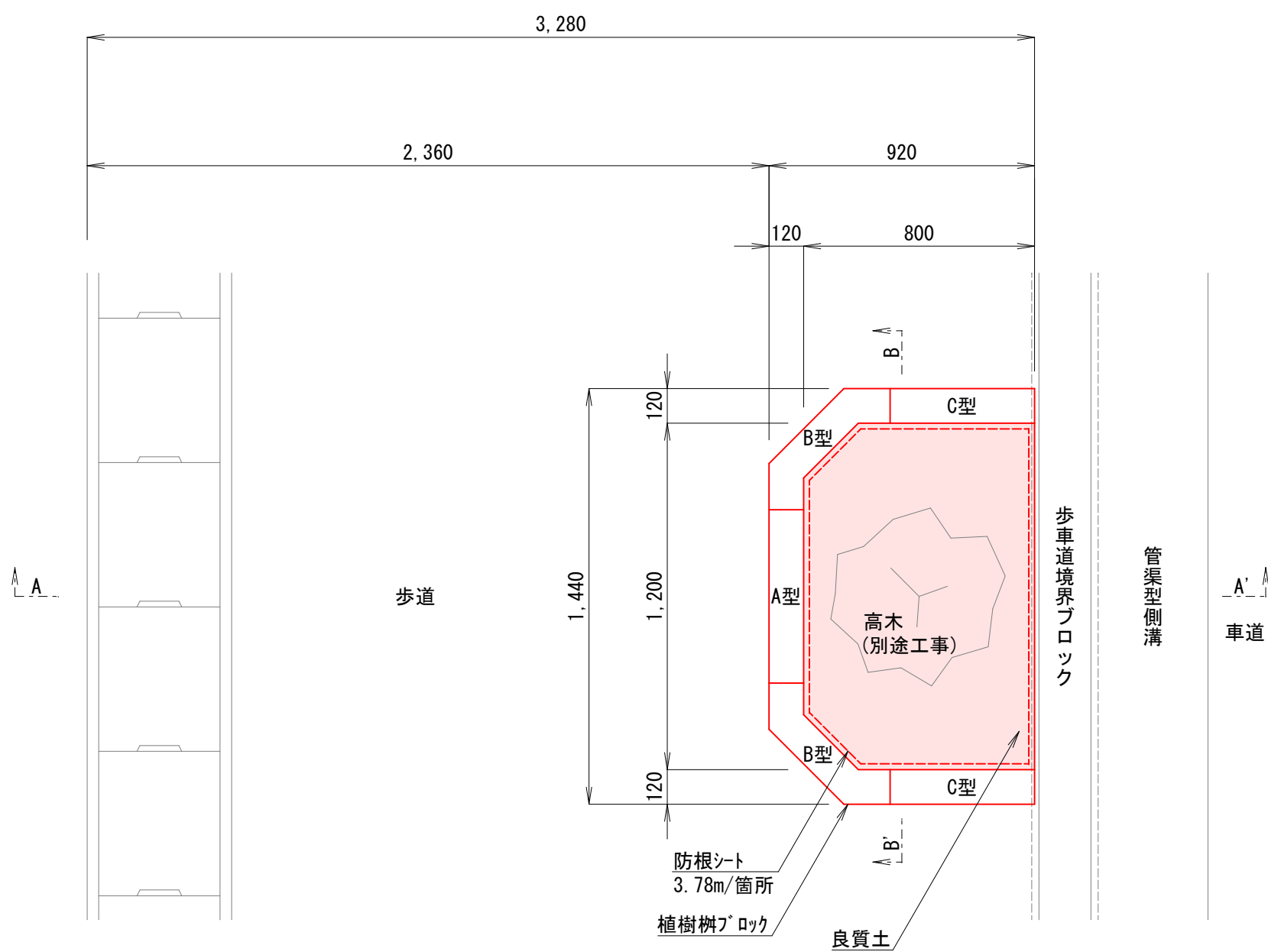
拡大平面図 S=1:20
