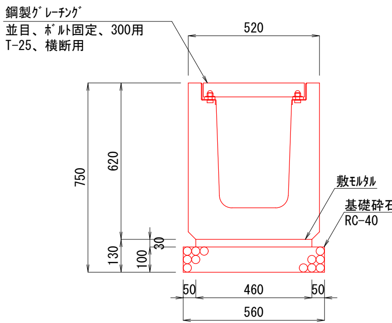
U型側溝 【PU3-B300-H400 (横断用)】
