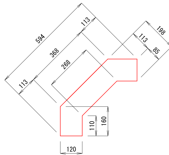
【植樹柵ブロック(B型)】 S=1:10
