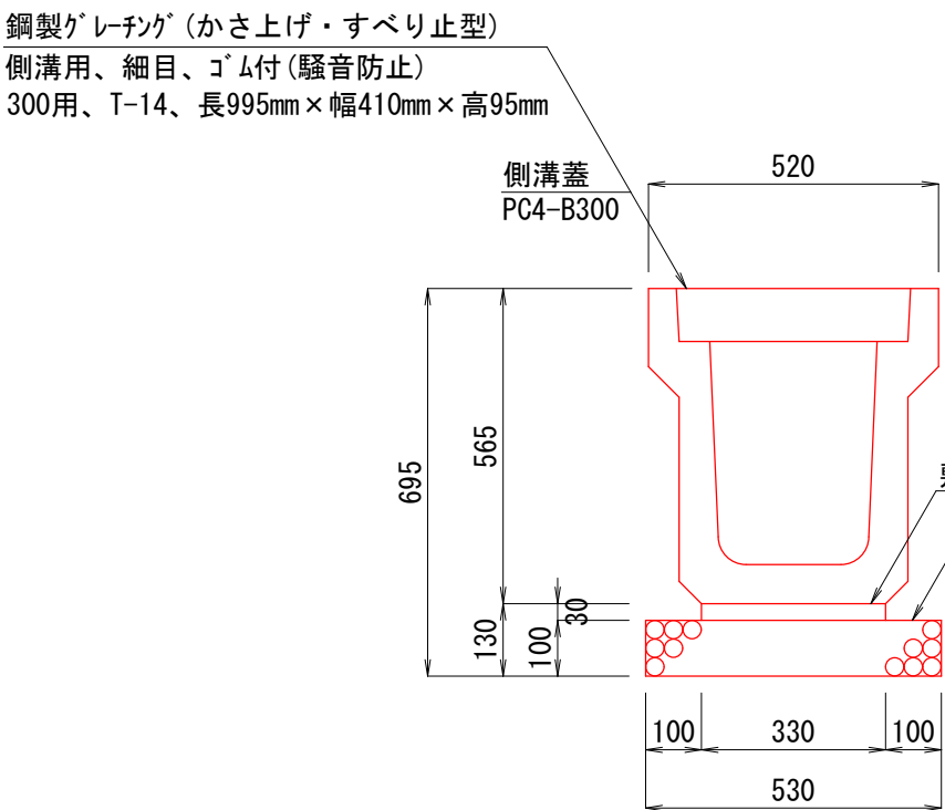
U型側溝 (PU3-B300-H400)
