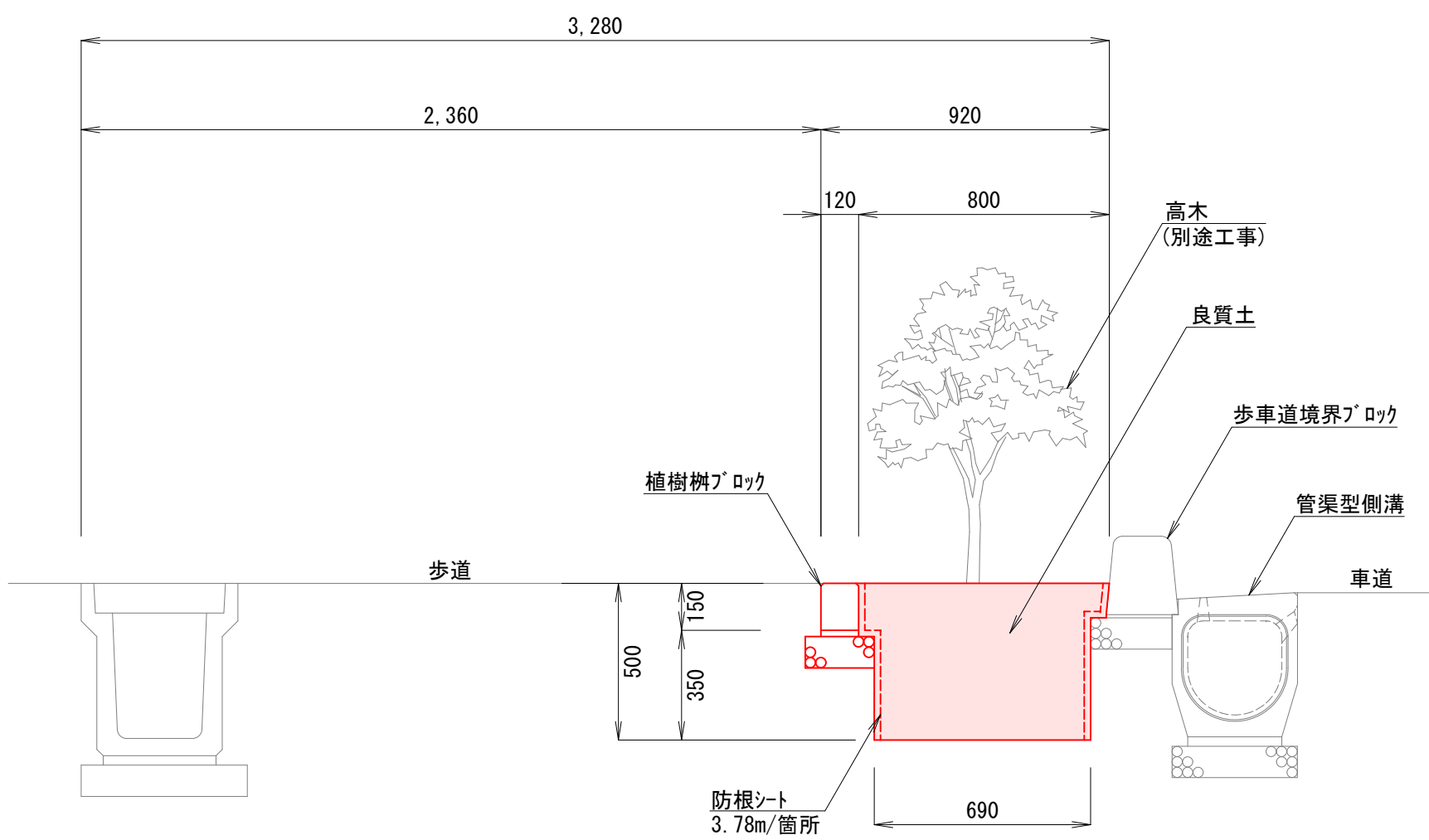
A-A' 断面図 S=1:20
