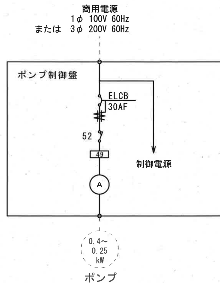
單線結線図
