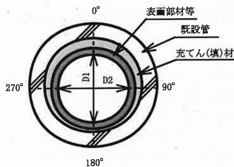
図1 仕上がり内径を測定する位置
