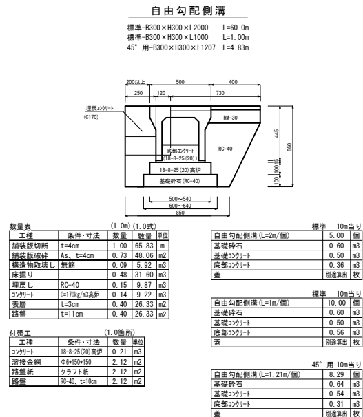
構造図 S=1:30
