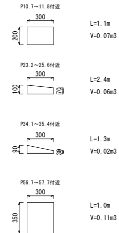
構造物取壊し図 S=1:30
