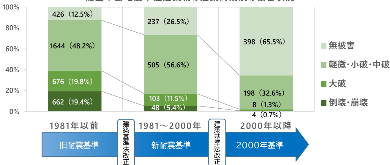
能登半島地震木造建築物の建築時期別の被害状況
