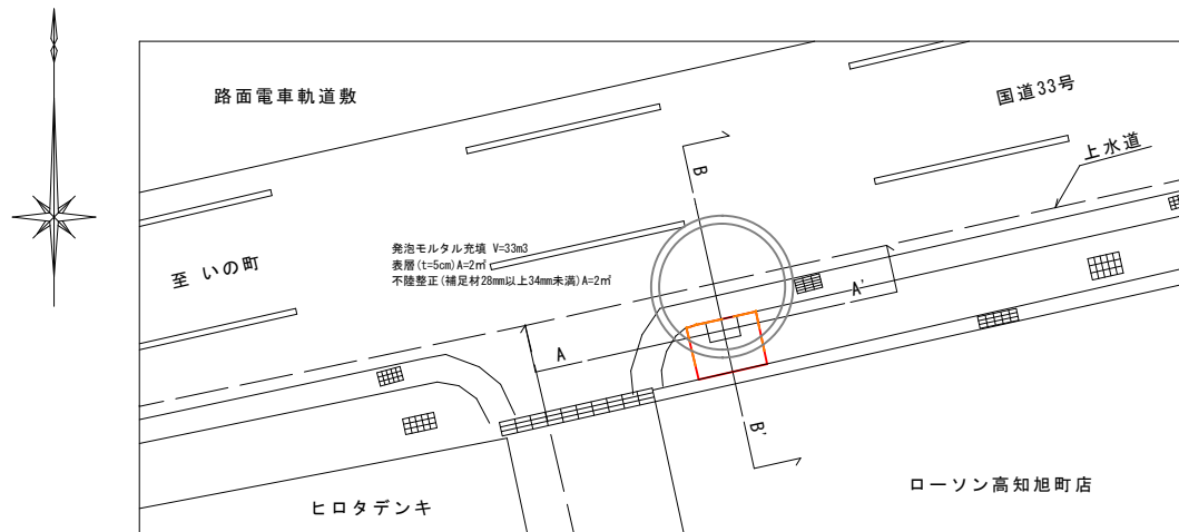
舗装展開図 S=1:30
