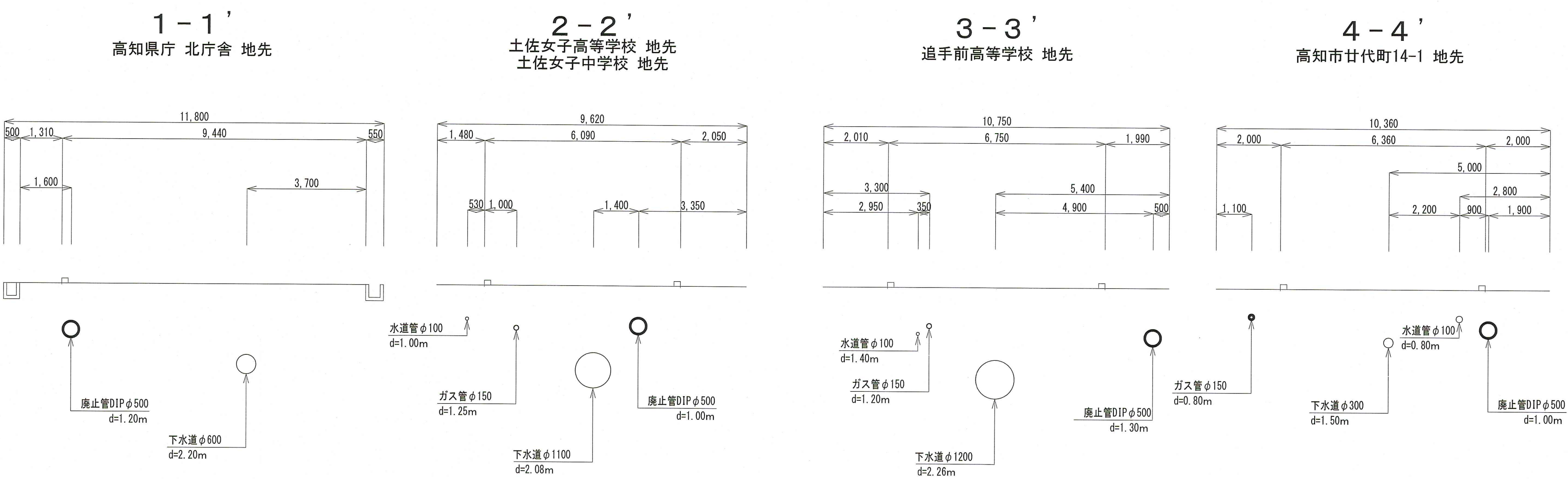
横断図（１） S=1:100
