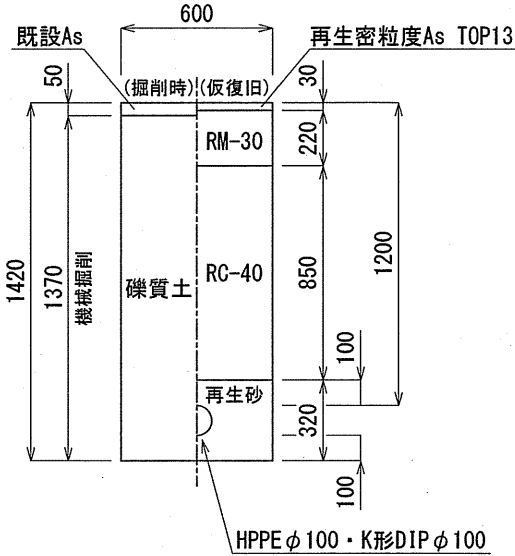
HPPEφ100・K形DIPφ100連絡部 L=4.7m
