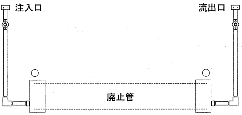
中詰充填工詳細図 S=Free
