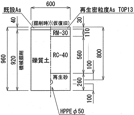
HPPEφ50標準部① L=2.8m
