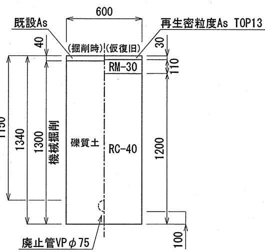
廃止管土工図③
