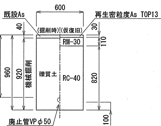
廃止管土工図④
