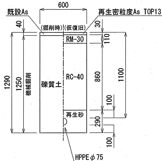
HPPEφ75標準部② L=173.5m
