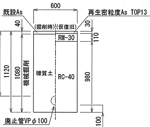
廃止管土工図⑥
