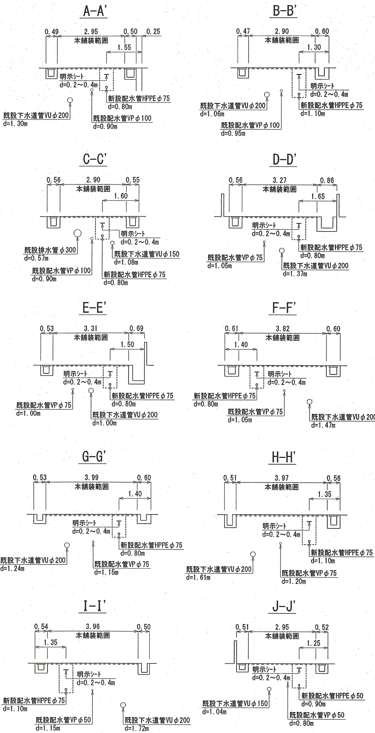
横断面図 S=1:100
