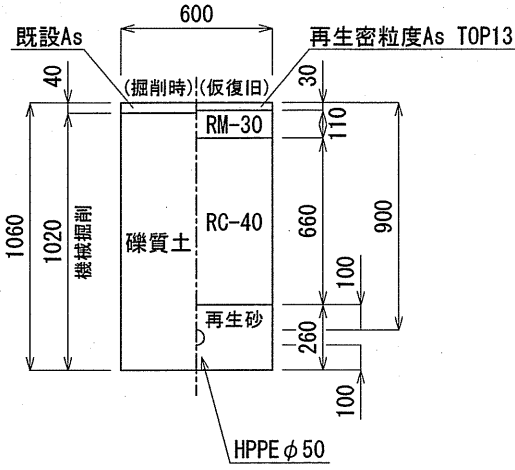
HPPEφ50標準部② L=39.6m
