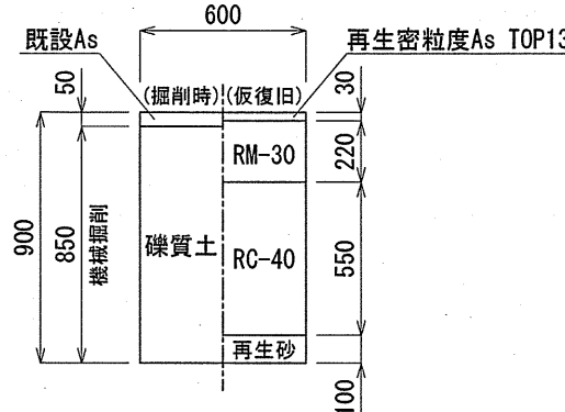
既設割字管副弁部 L=1.0m×2箇所
