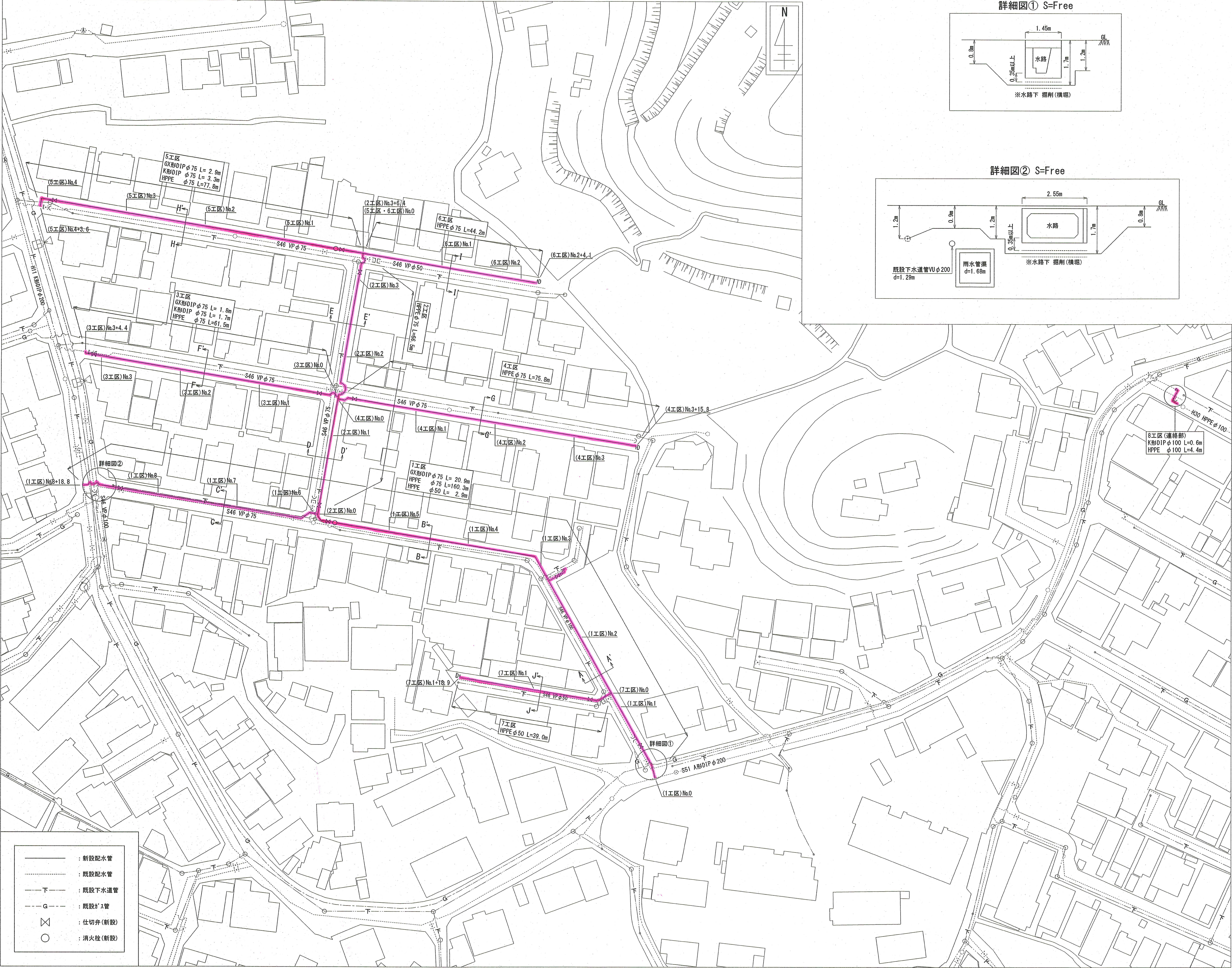
配水管平面図 S=1:500
