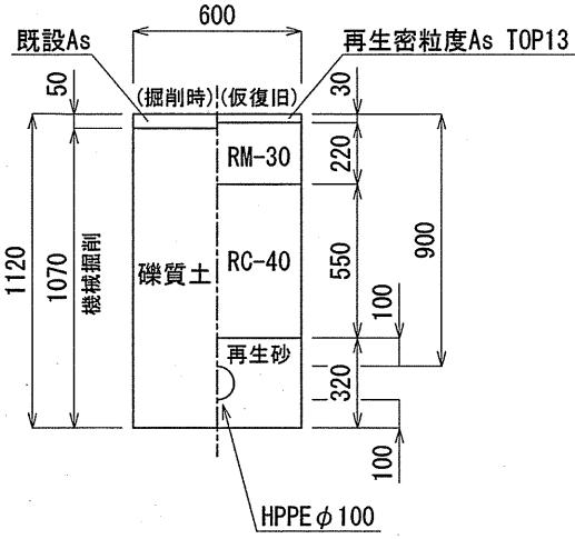
HPPEφ100連絡部 L=2.4m
