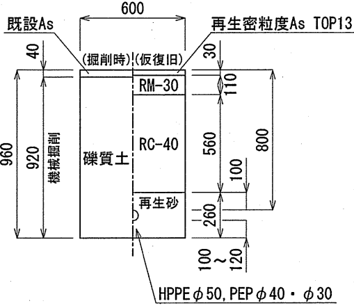
給水管切替土工図① S=1:30 L=3.5m 切替番号4
