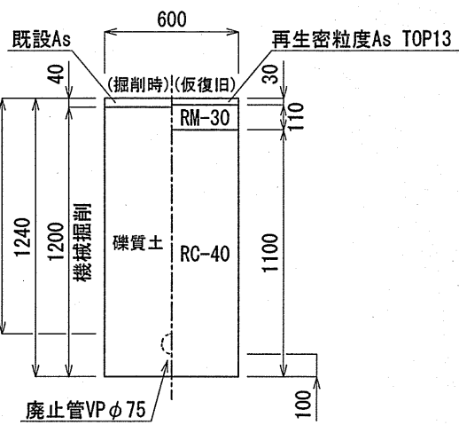
廃止管土工図②
