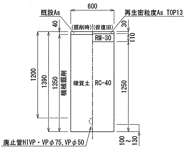
廃止管土工図①
