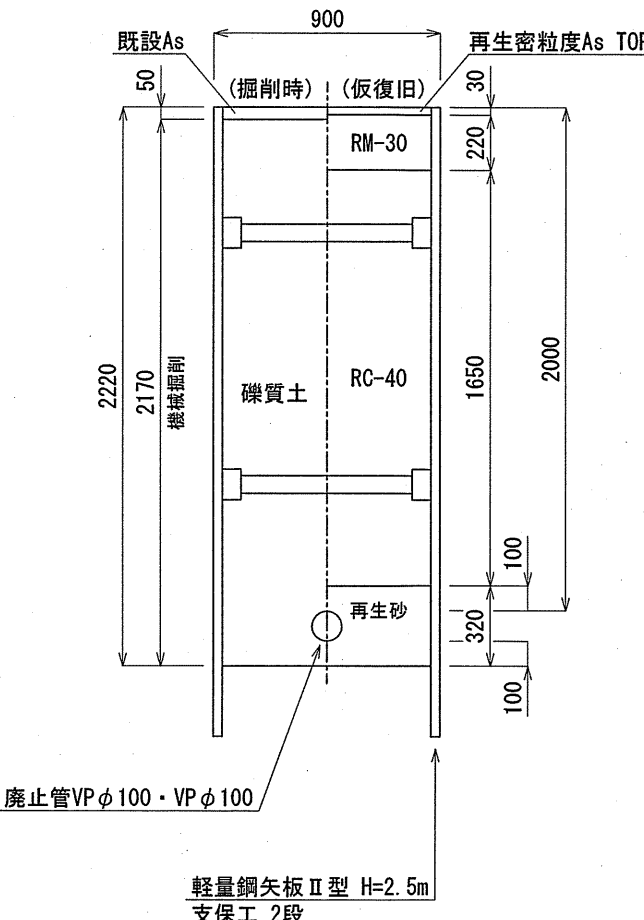
廃止管土工図⑤
