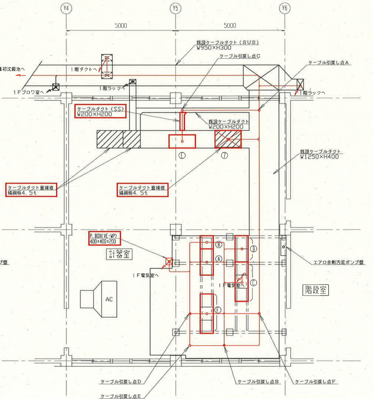
管理棟2階計器室平面図 S=1/100 (更新)
