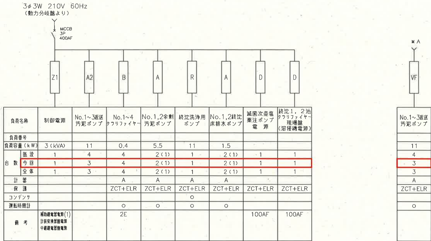
コントロールセンタ (CC-W1N) 単線結線図
