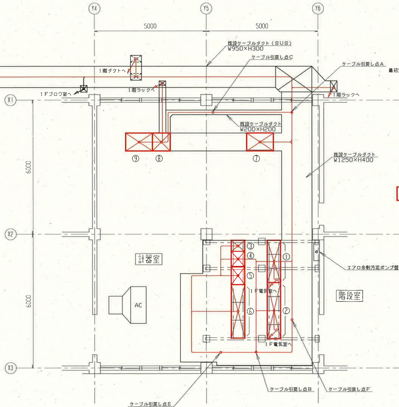
管理棟2階計器室平面図 S=1/100 (撤去)
