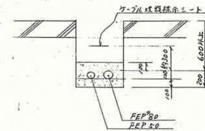
C部詳細断面図 S=1/20
