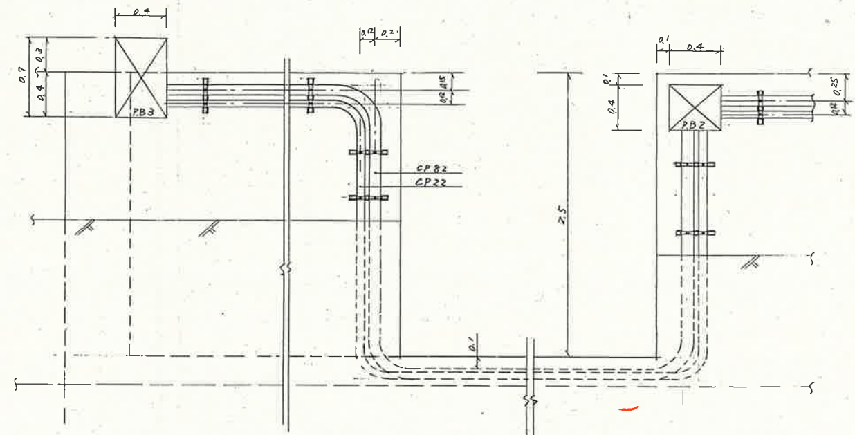
B-B 矢視図 S=1/20
