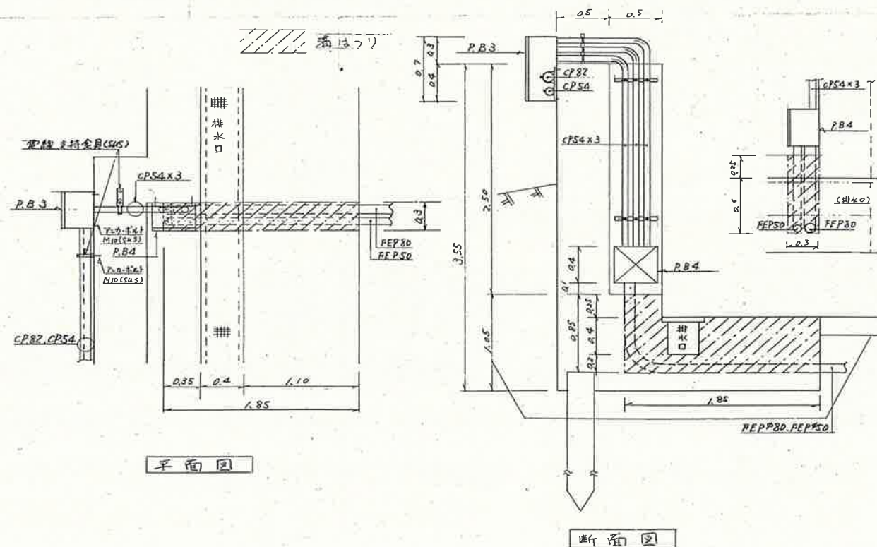
断面図
