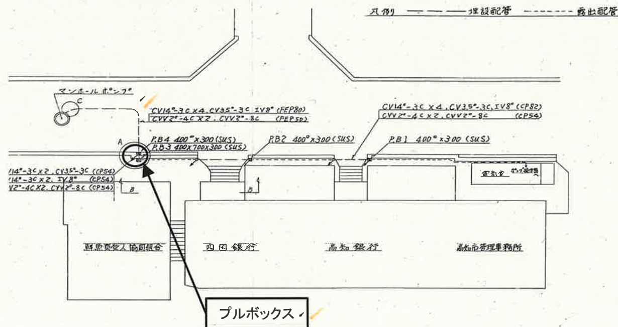
外部平面図 S=1/200
