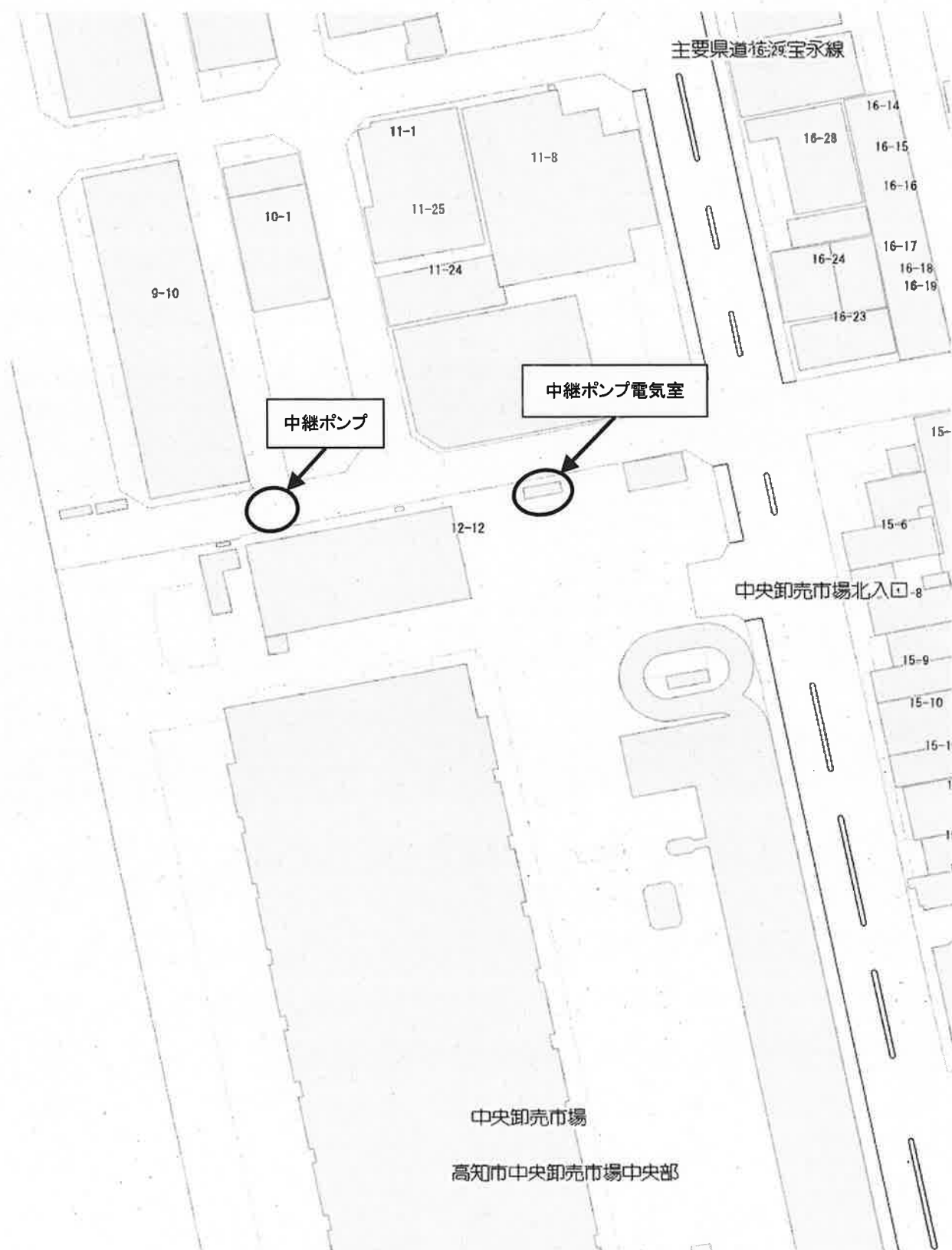
工事場所位置図(弘化台中継ポンプ場)
