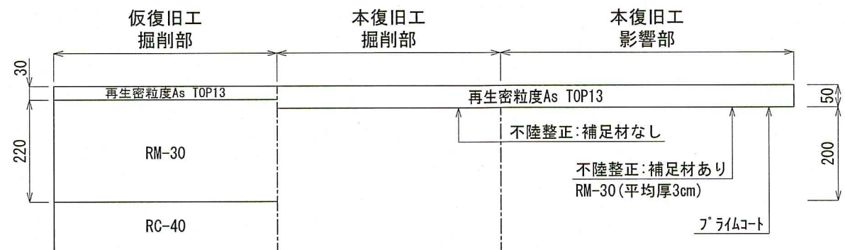
市道車道部 (As舗装)
