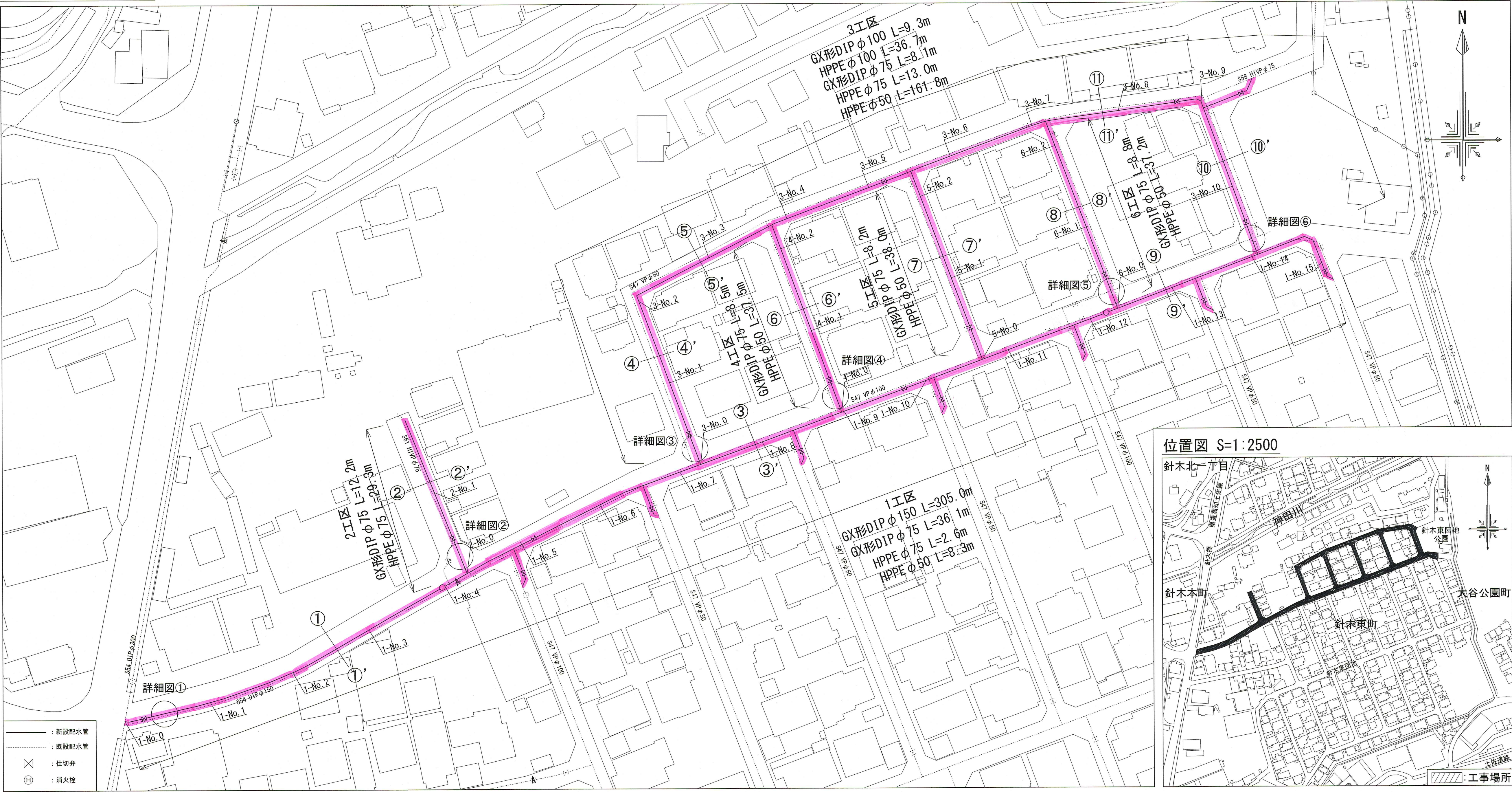
配水管平面図 S=1:500
