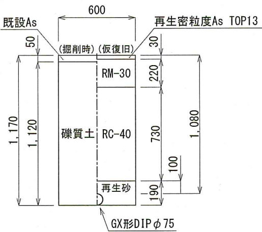
GX形DIPφ75伏越部②
