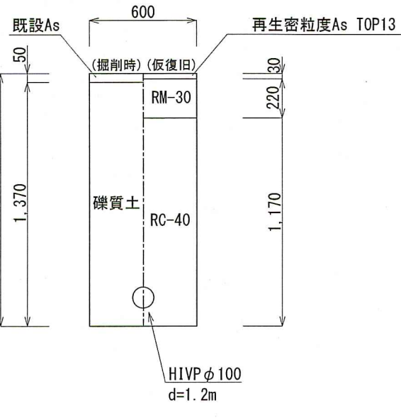
流出口①-2、流入口② L=2.0m 市車道 (4.0m以上)
