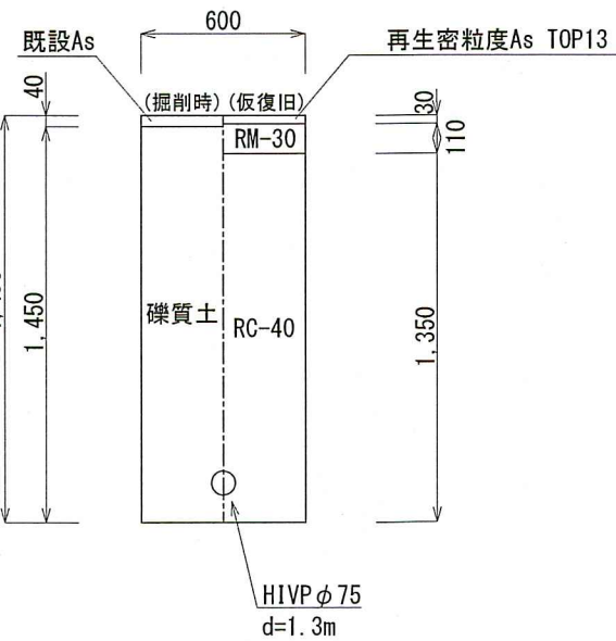
流出口①-1 L=2.0m 市車道 (4.0m未満)
