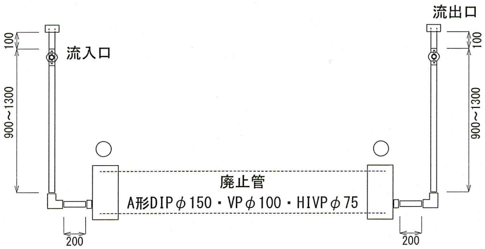
中詰め充填工詳細図 S=Free 廃止管 L≤250.0m×2区間
