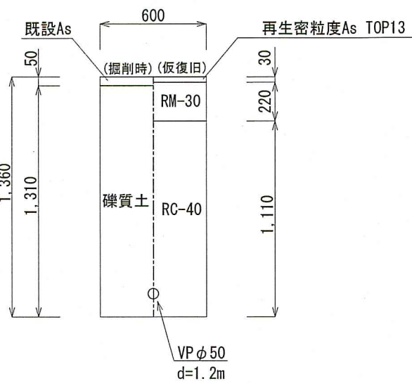
VP φ50閉塞部 L=2.0m×6箇所 市車道 (4.0m以上)
