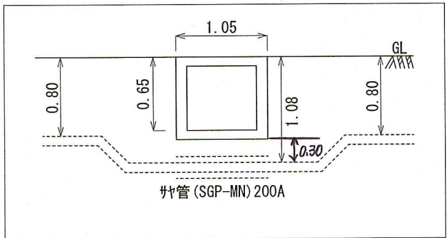
詳細③④⑤配管図
