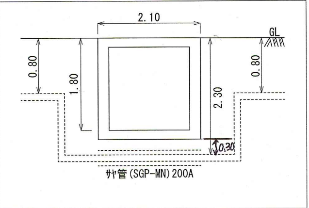
詳細②配管図
