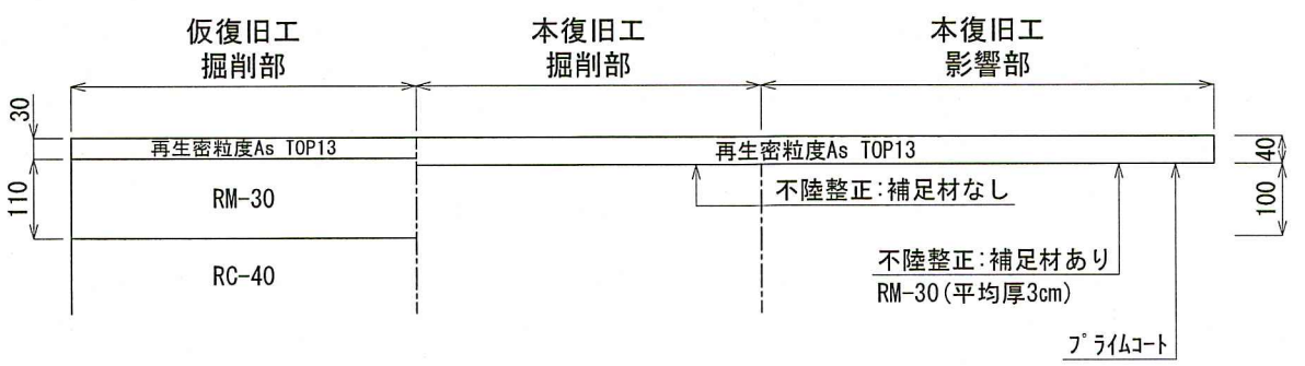
市道車道部 (As舗装)
