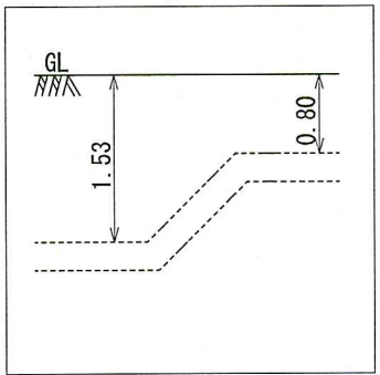
詳細①配管図
