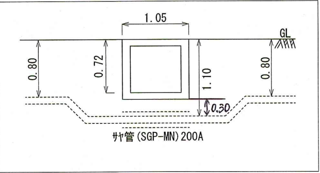
詳細⑥配管図
