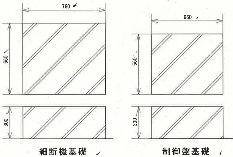
機械基礎図
