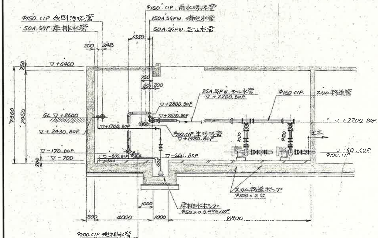
B-B 断面
