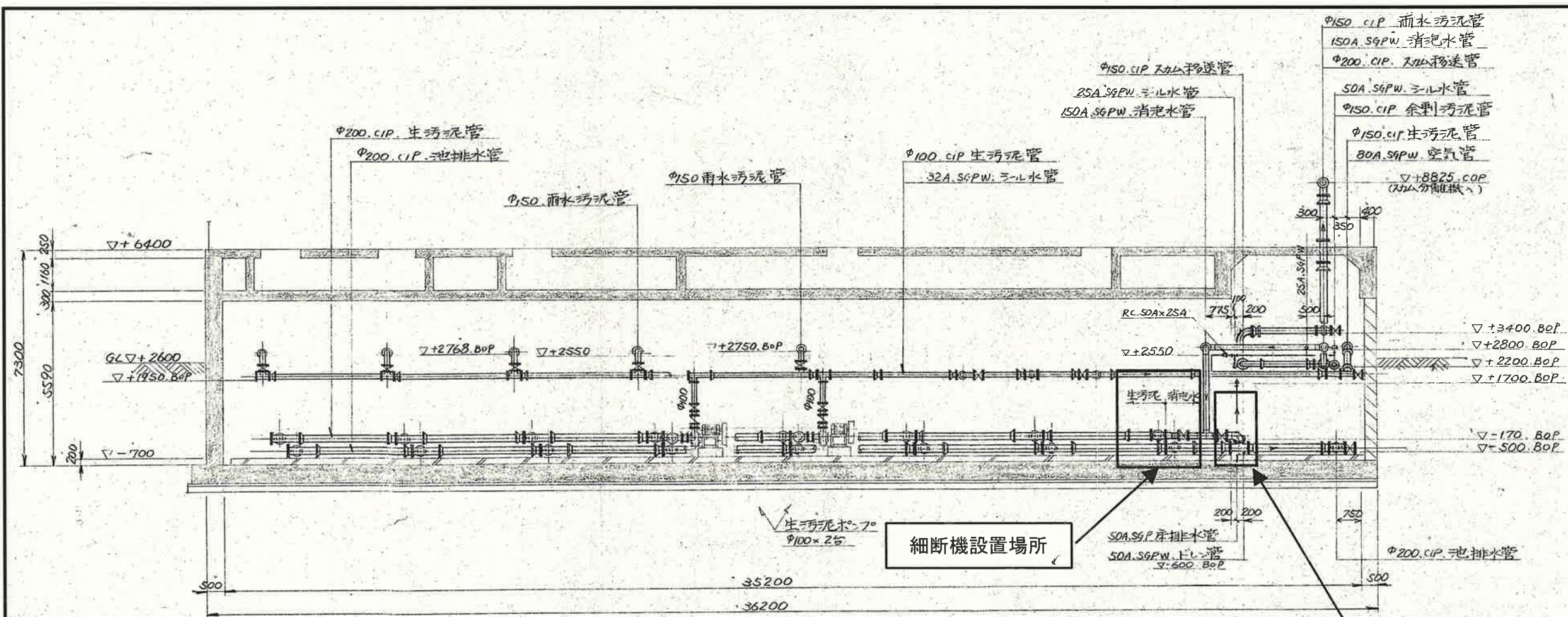
A-A 断面
