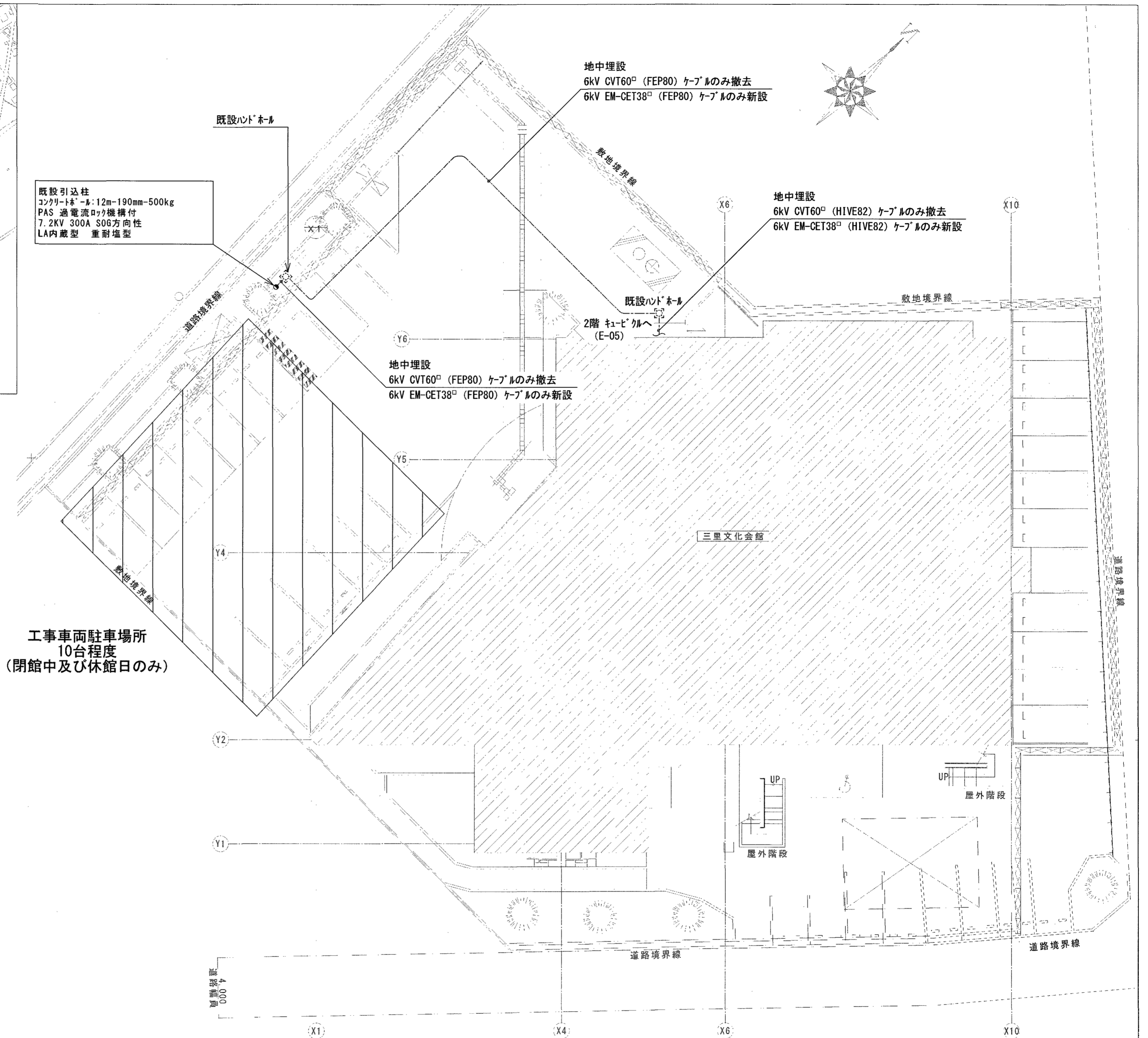
配置図 1/200
