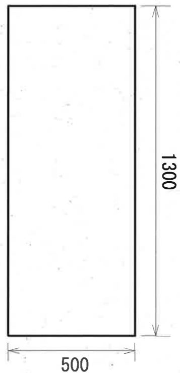
中板寸法図 (S=1/15) (SS製)
