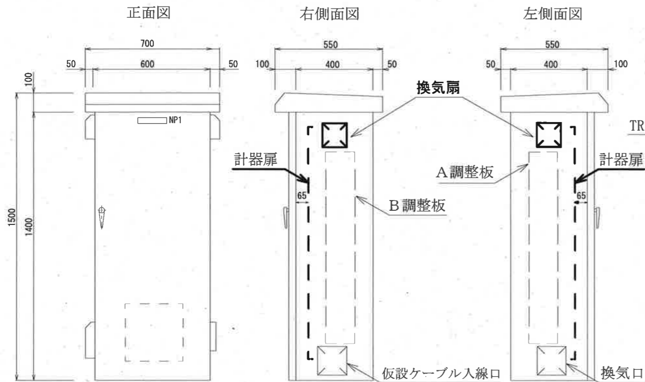
ポンプ制御盤外形図 (S=1/20) (ステンレス製)
