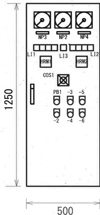
計器扉機器配置図 (S=1/15) (SS製)
