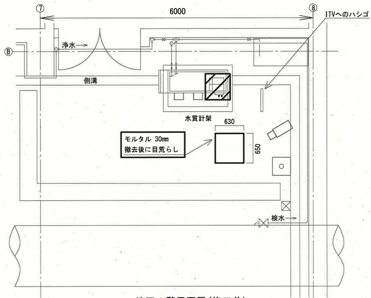
地下1階平面図(施工前) (S=1/50)
