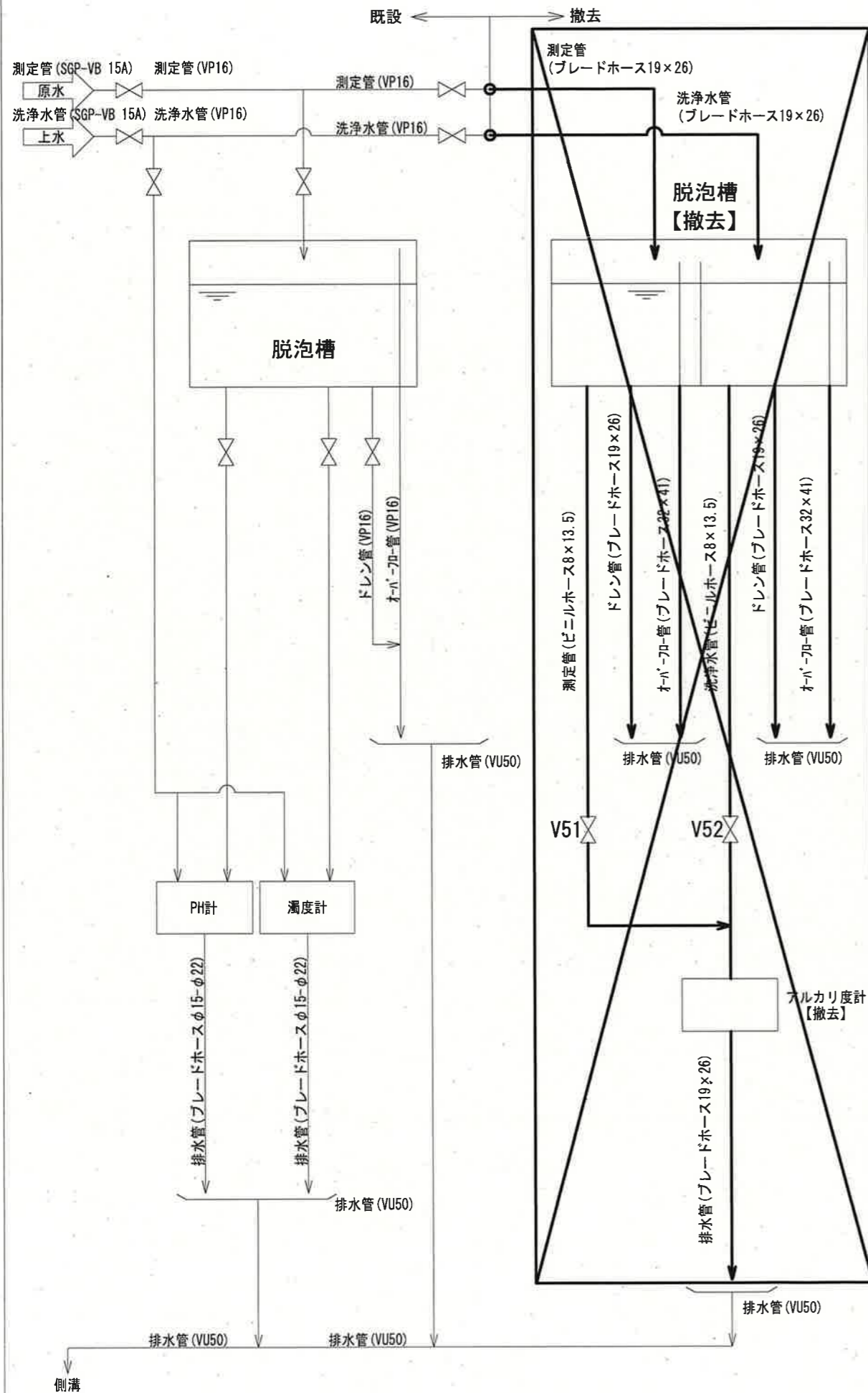
測定フロー図(施工前)
