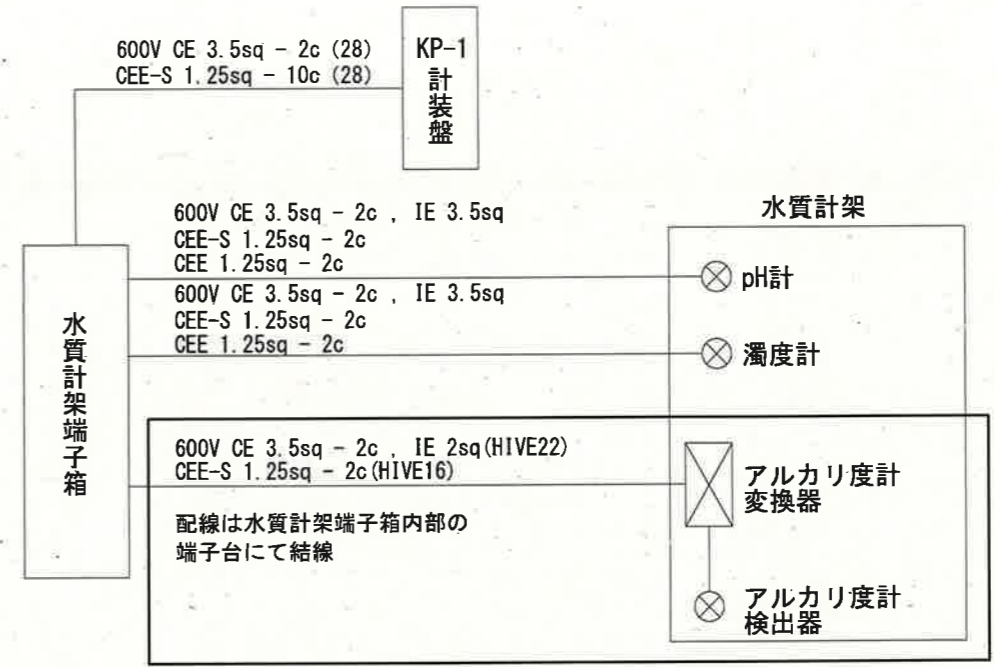
配線系統図 (施工後)
