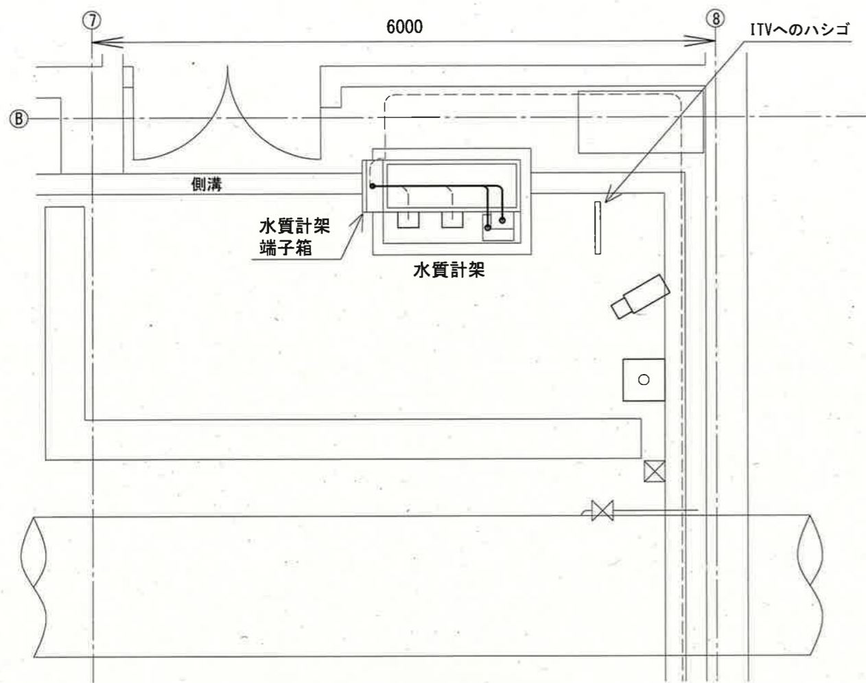
地下1階 平面図 (施工前) (S=1/50)
