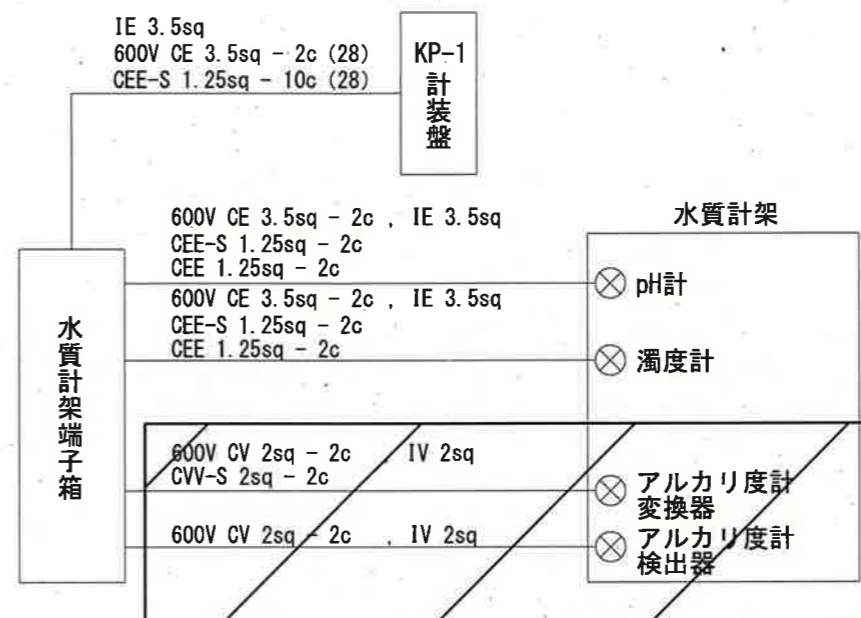
配線系統図 (施工前)
