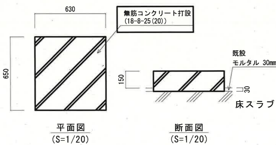
無筋コンクリート基礎図
