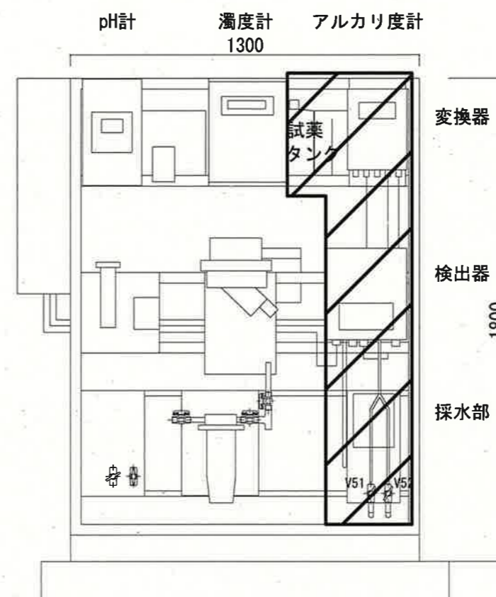
水質計架 立面図 (S=1/20)
