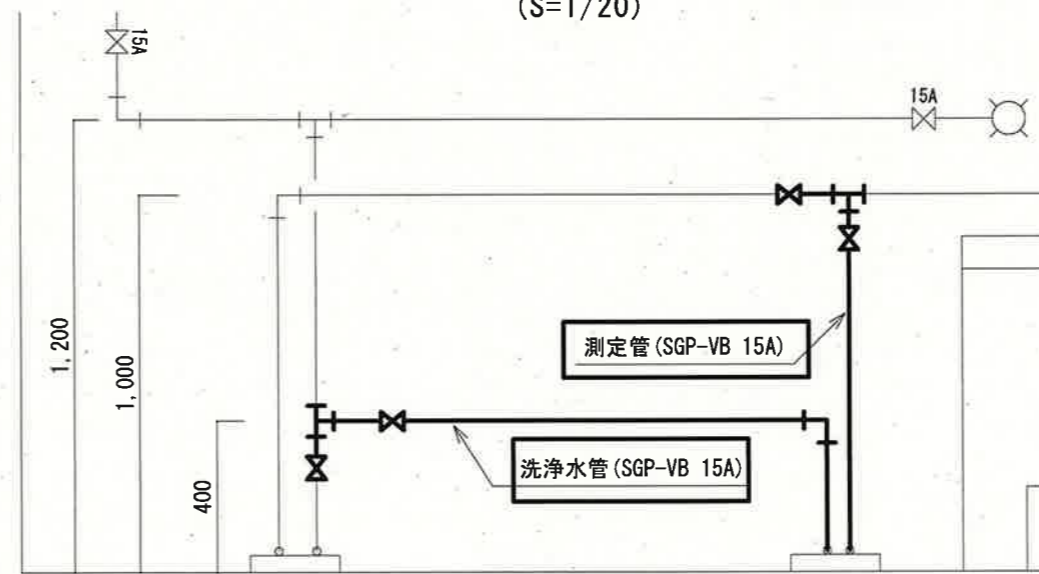
断面図 B-B (S=1/20)
