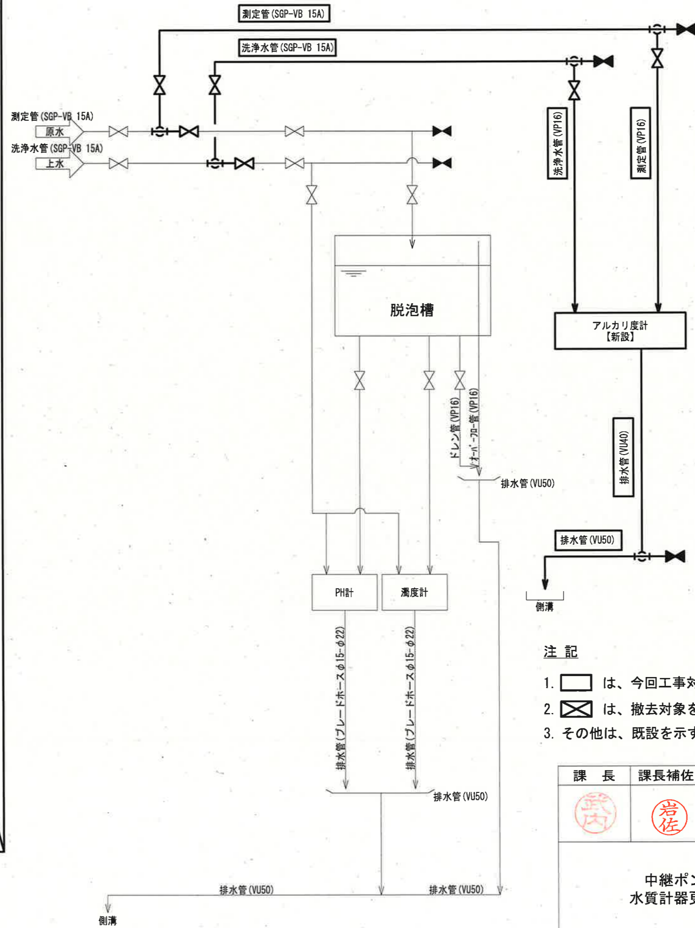
測定フロー図(施工後)
