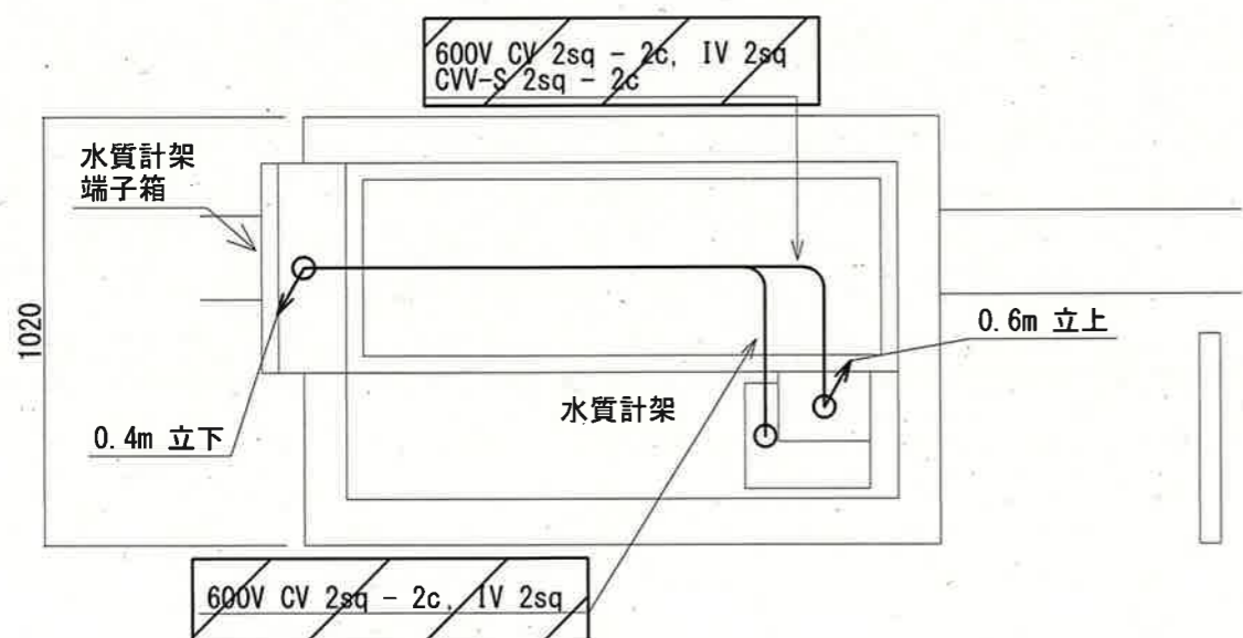
地下1階 配線平面図 (撤去) (S=1/20)
