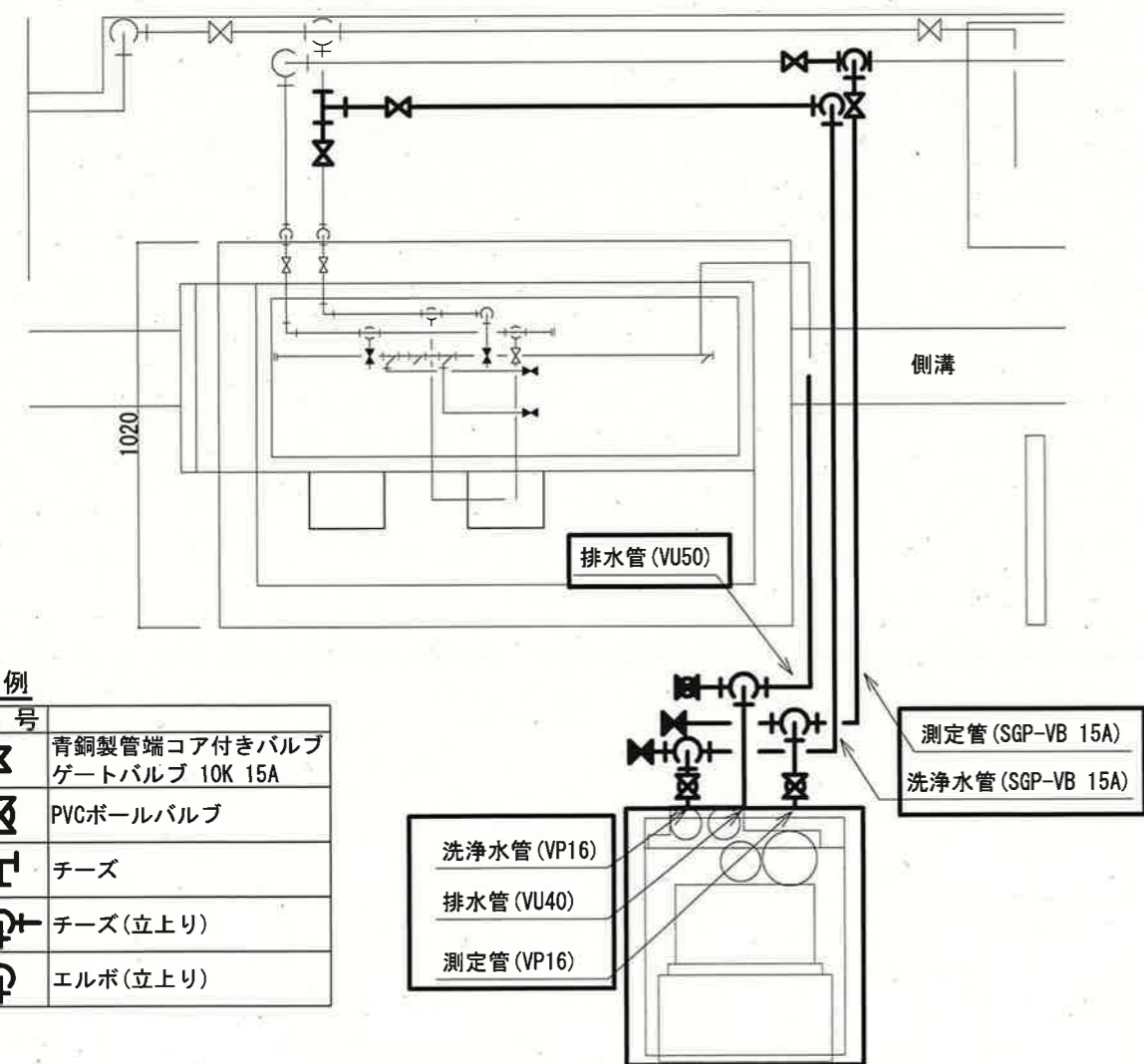
地下1階 配管平面図 (新設) (S=1/20)
