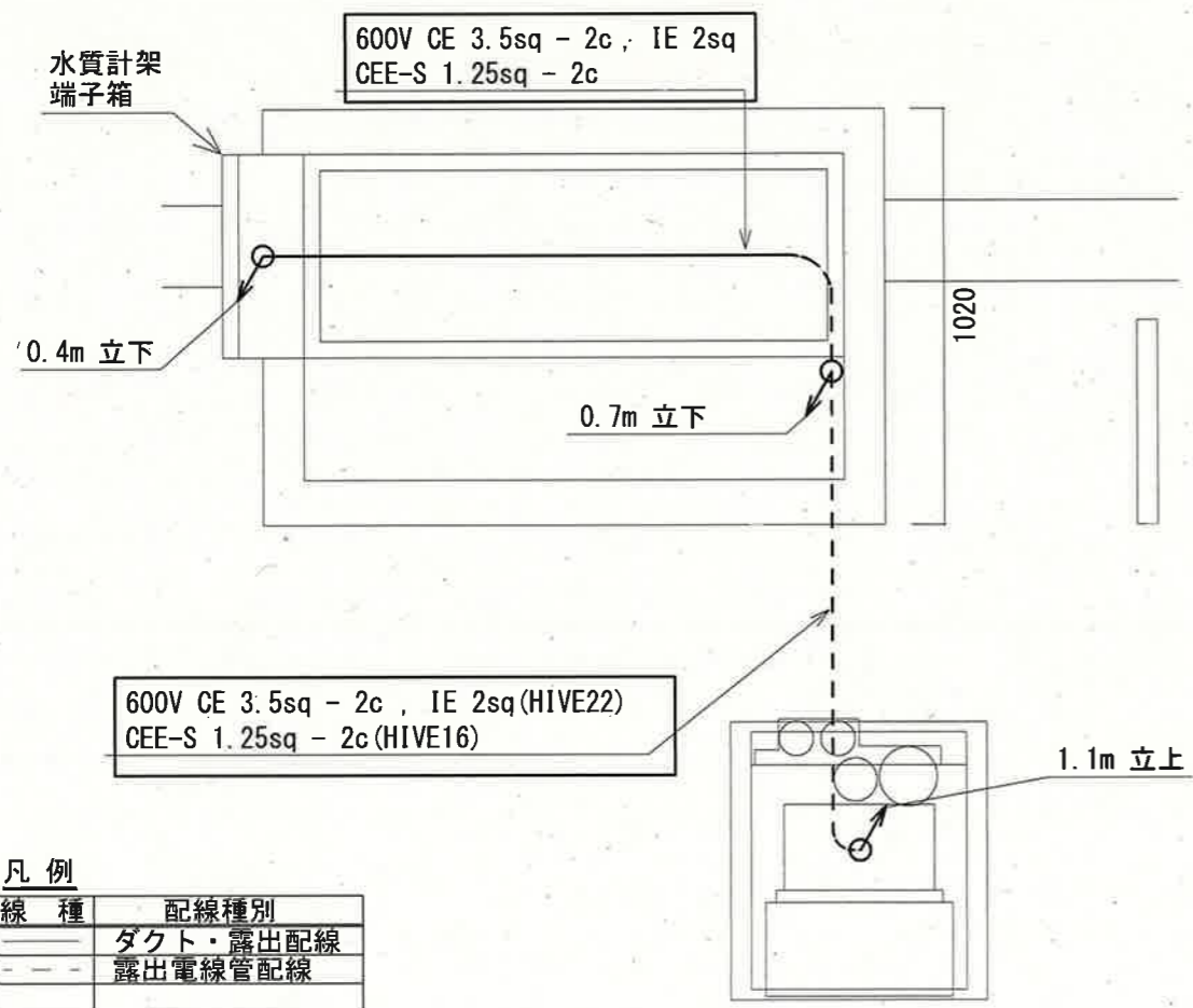
地下1階 配線平面図 (新設) (S=1/20)
