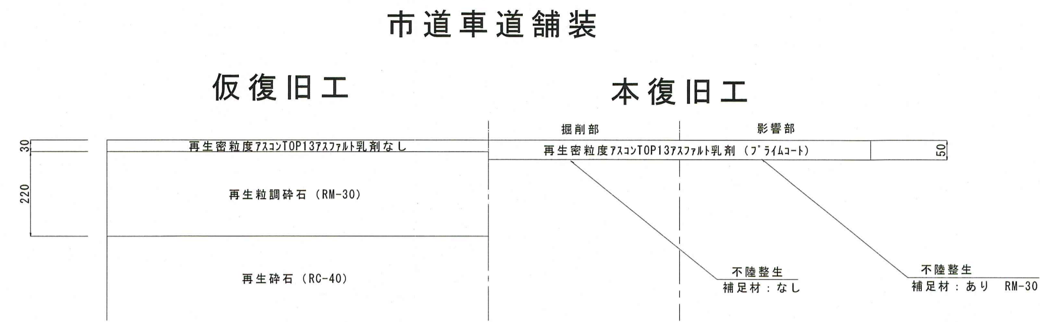
舗装構成図 S=1:10
