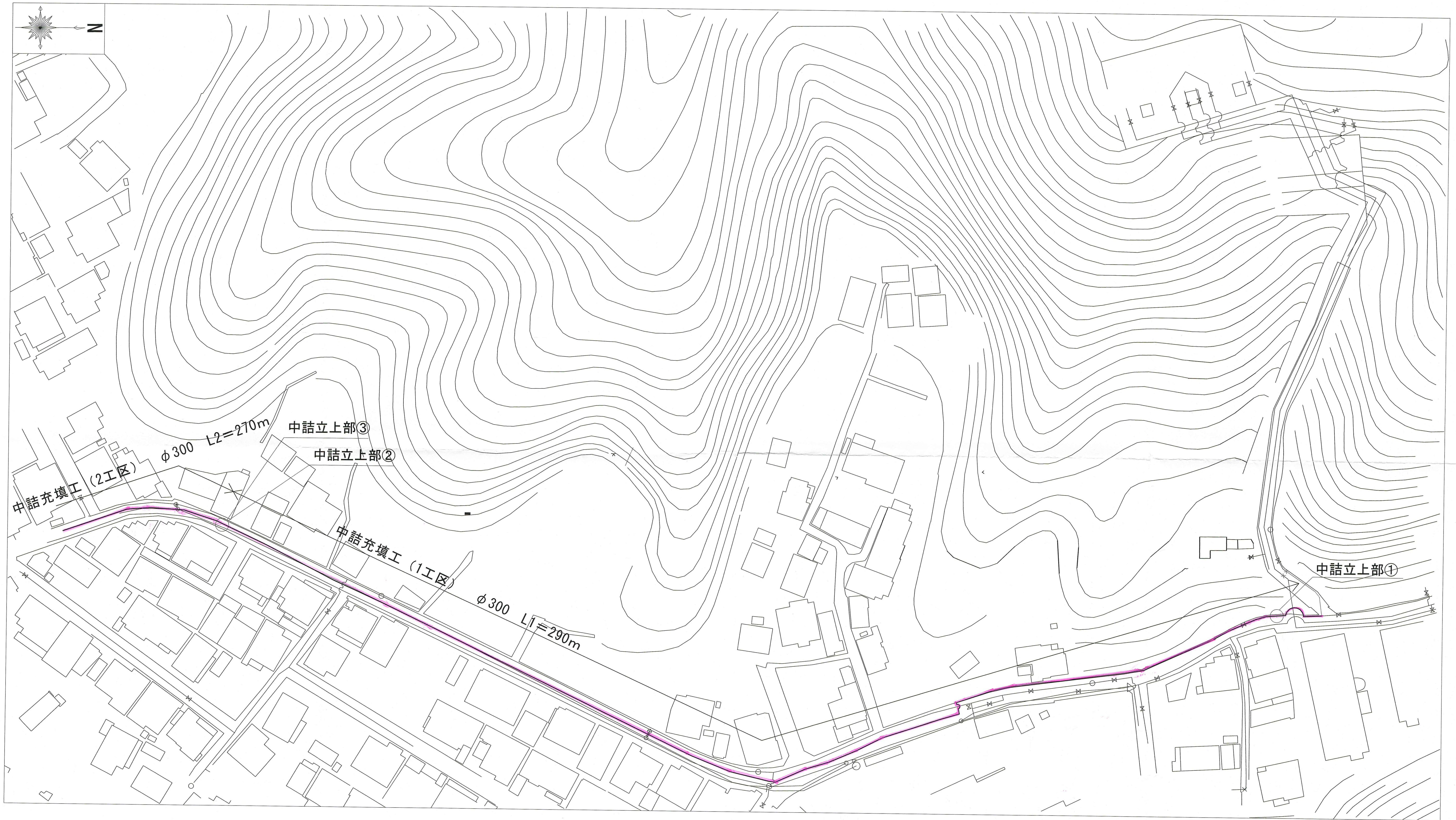
平面図 (1) S=1:500
