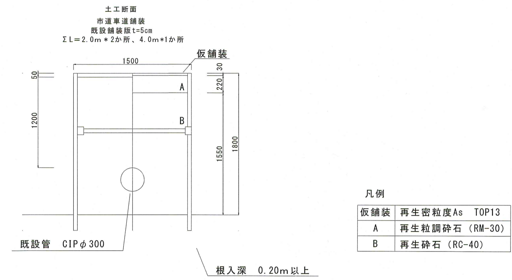
土工図 S=1:30
