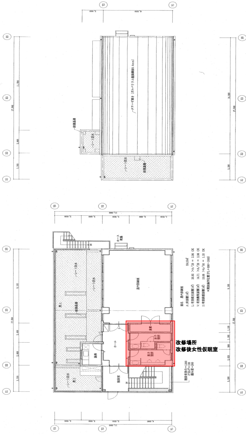
屋根伏図 1:100
