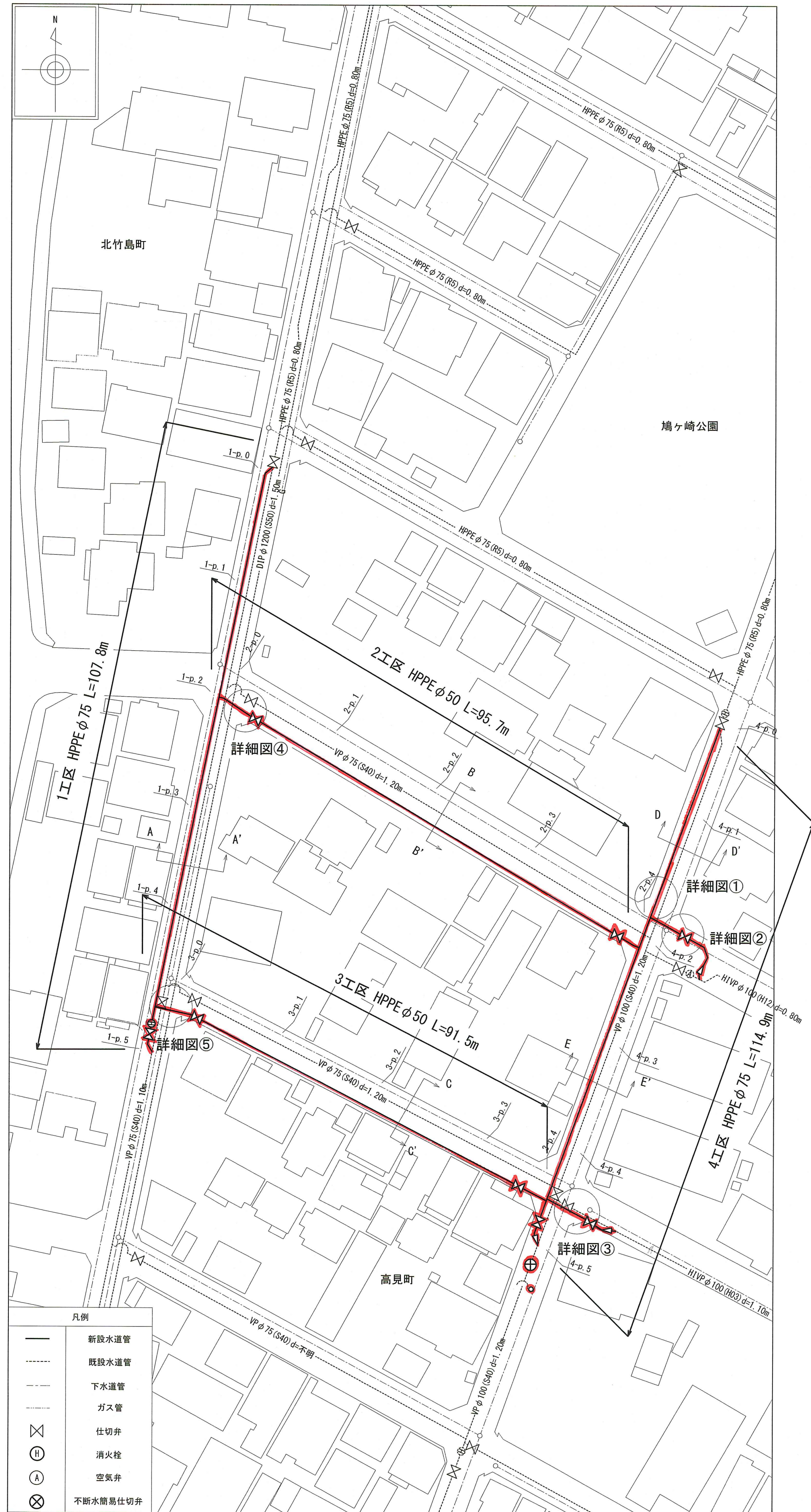
平面図① S=1:500
