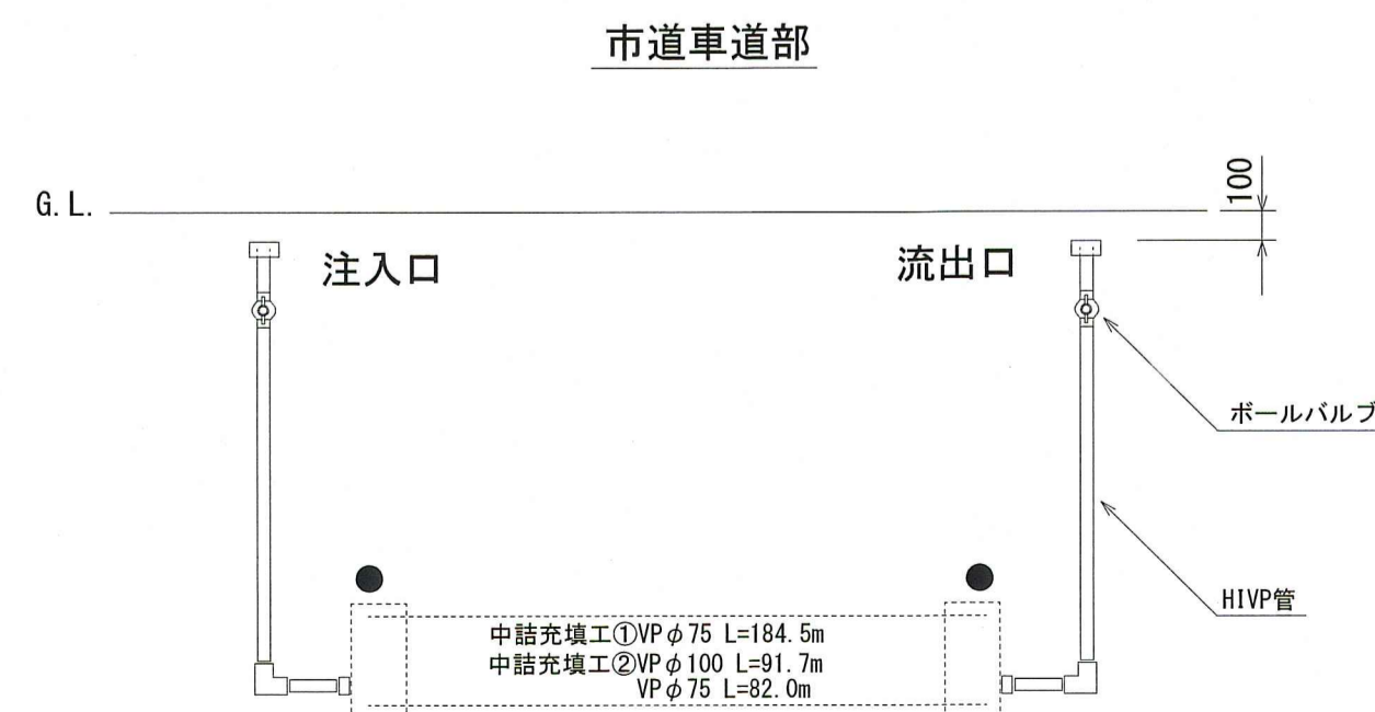
廃止管中詰充填図 S=1:Free
