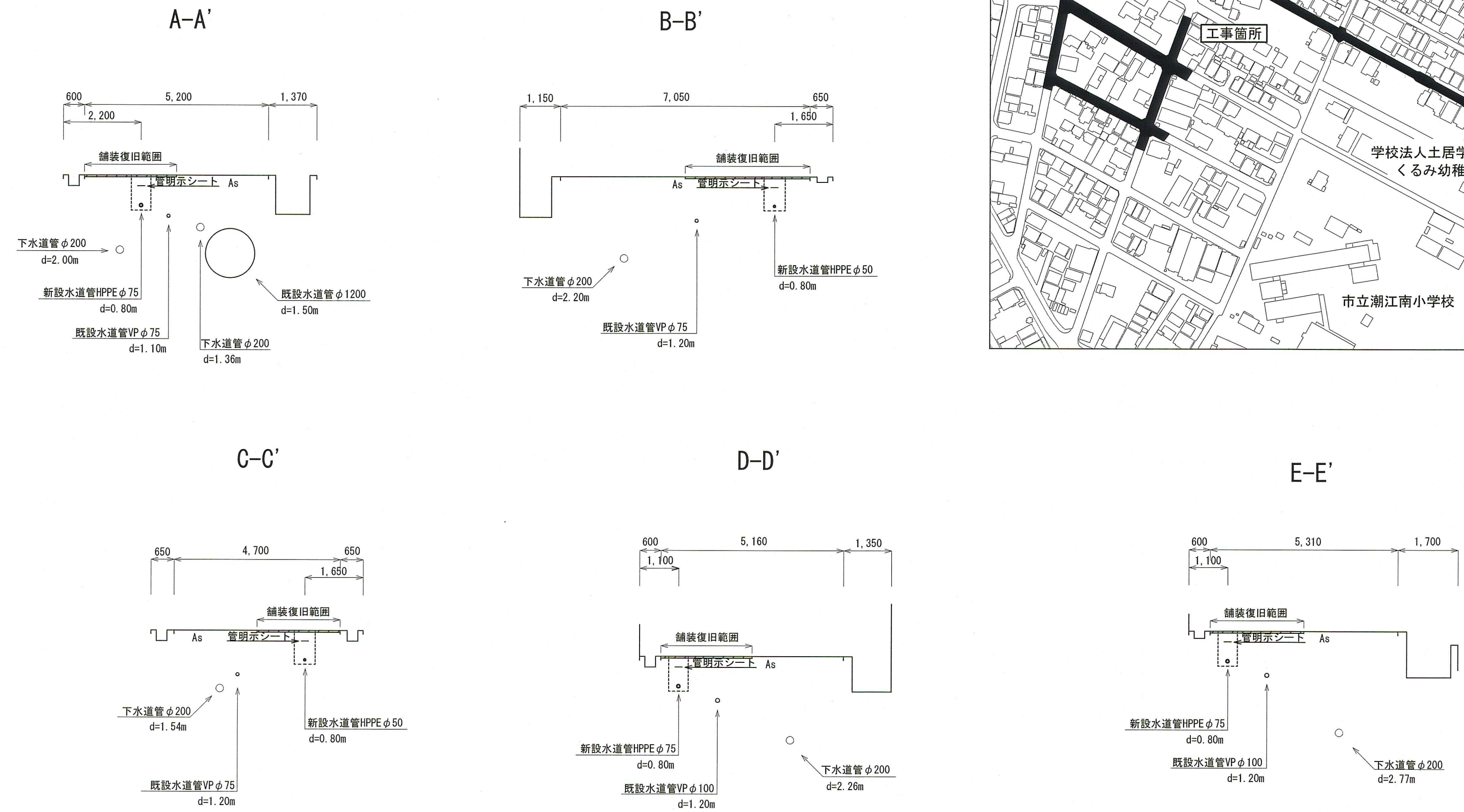
詳細図 S=1:Free
