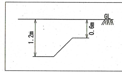
詳細図① S=Free
