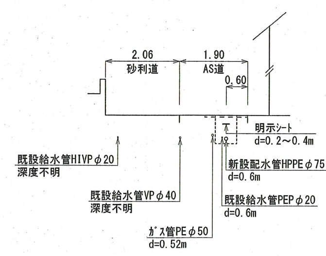
A-A' 横断面図 S=1:100
