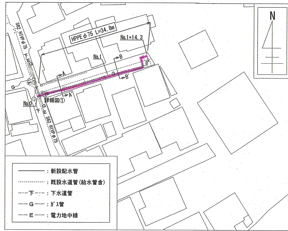
配水管平面図 S=1:500
