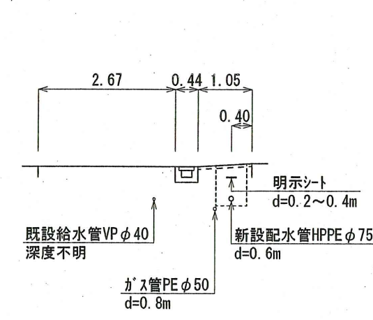
B-B' 横断面図 S=1:100
