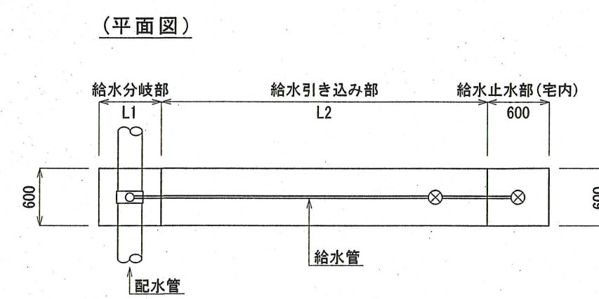
切替標準図 S=Free
