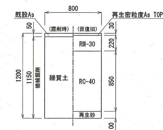
給水管外線撤去部 (分水栓キップφ20) L=0.8m 市車道
