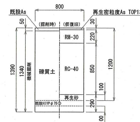
給水管外線撤去部 (SU用キップφ40) L=0.8m 市車道
