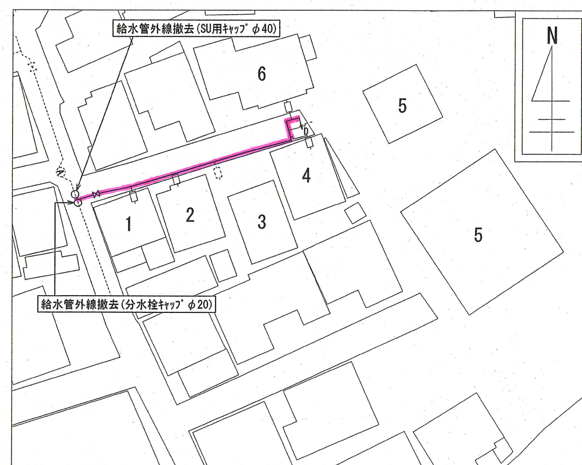
給水管平面図 S=1:500
