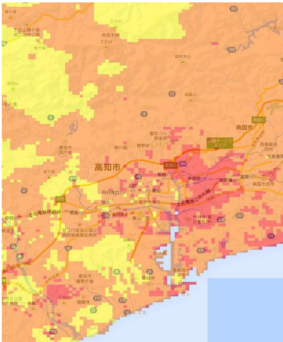
図 3-2 高知県における震度分布図（出典：高知県庁HPより）ooo999990
