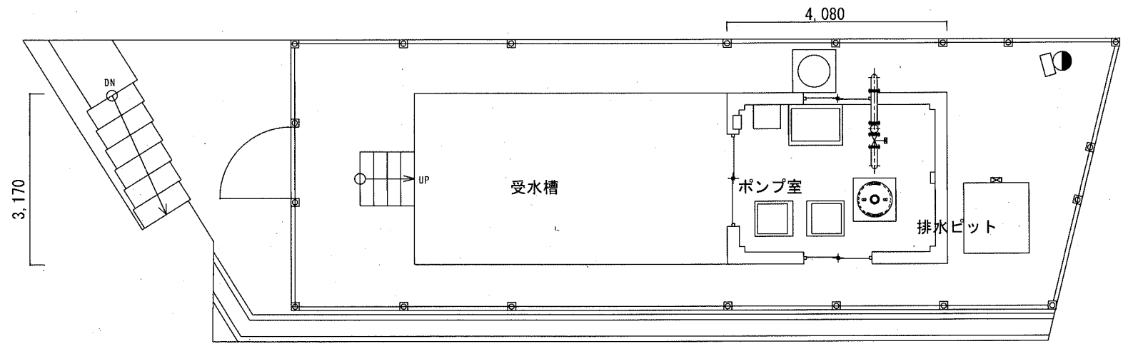
送水ポンプ所一般平面図 (S=1/100)
