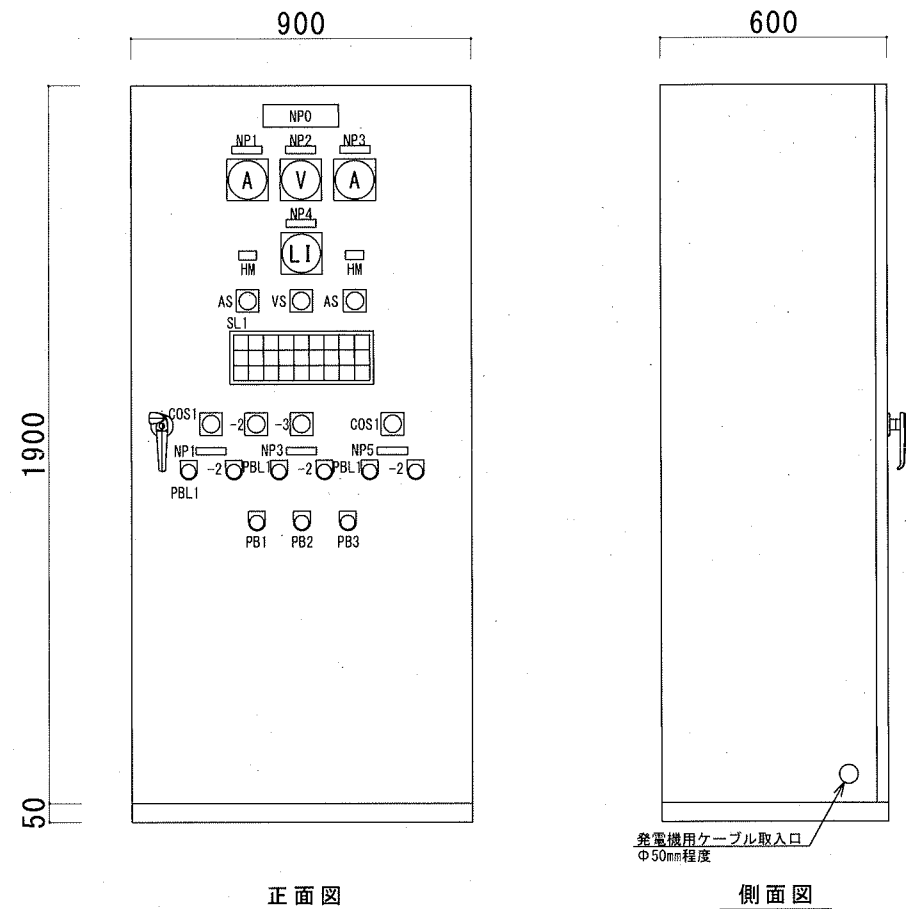
送水ポンプ盤 S=1/20
