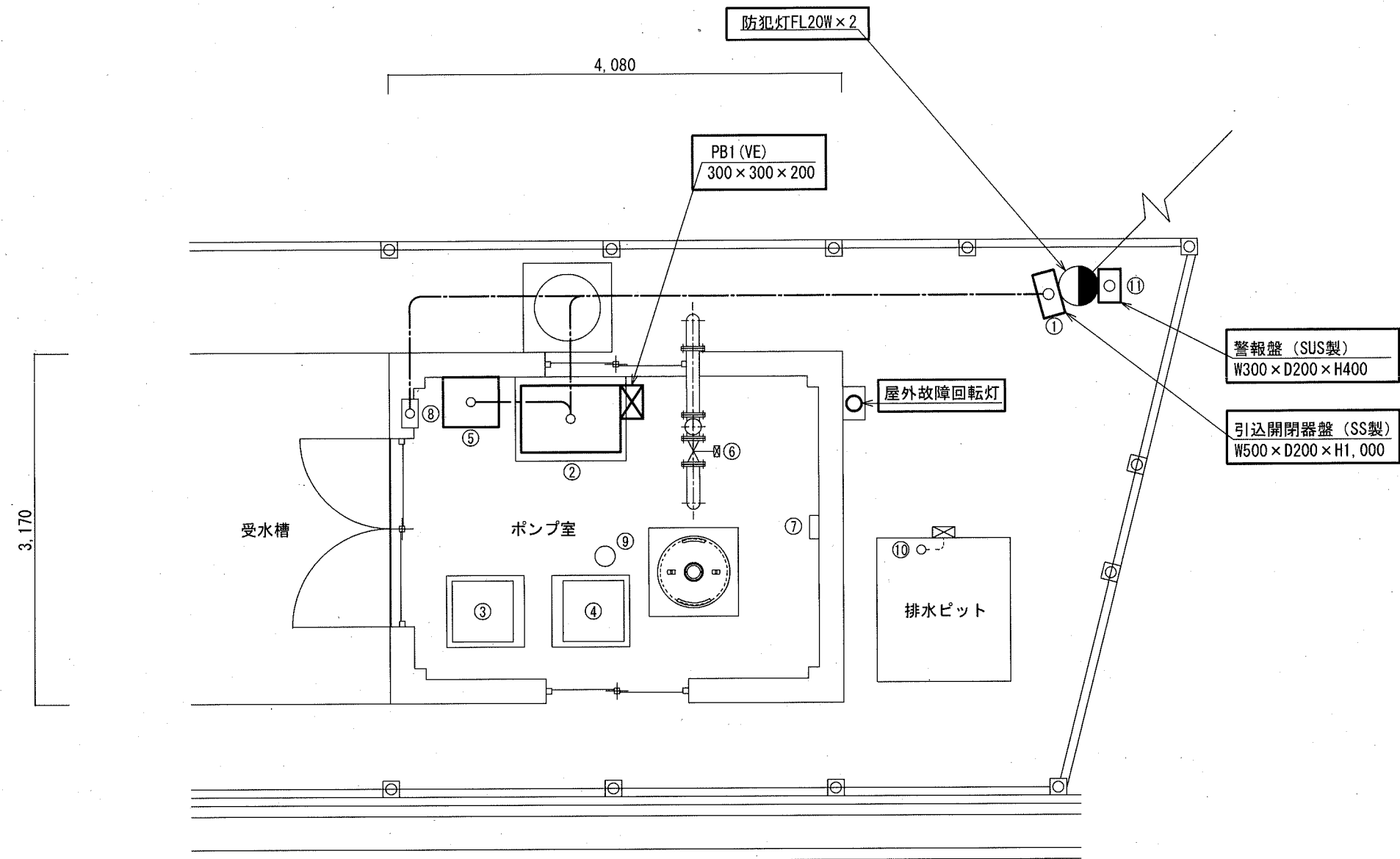
改修前平面図 (1/50)
