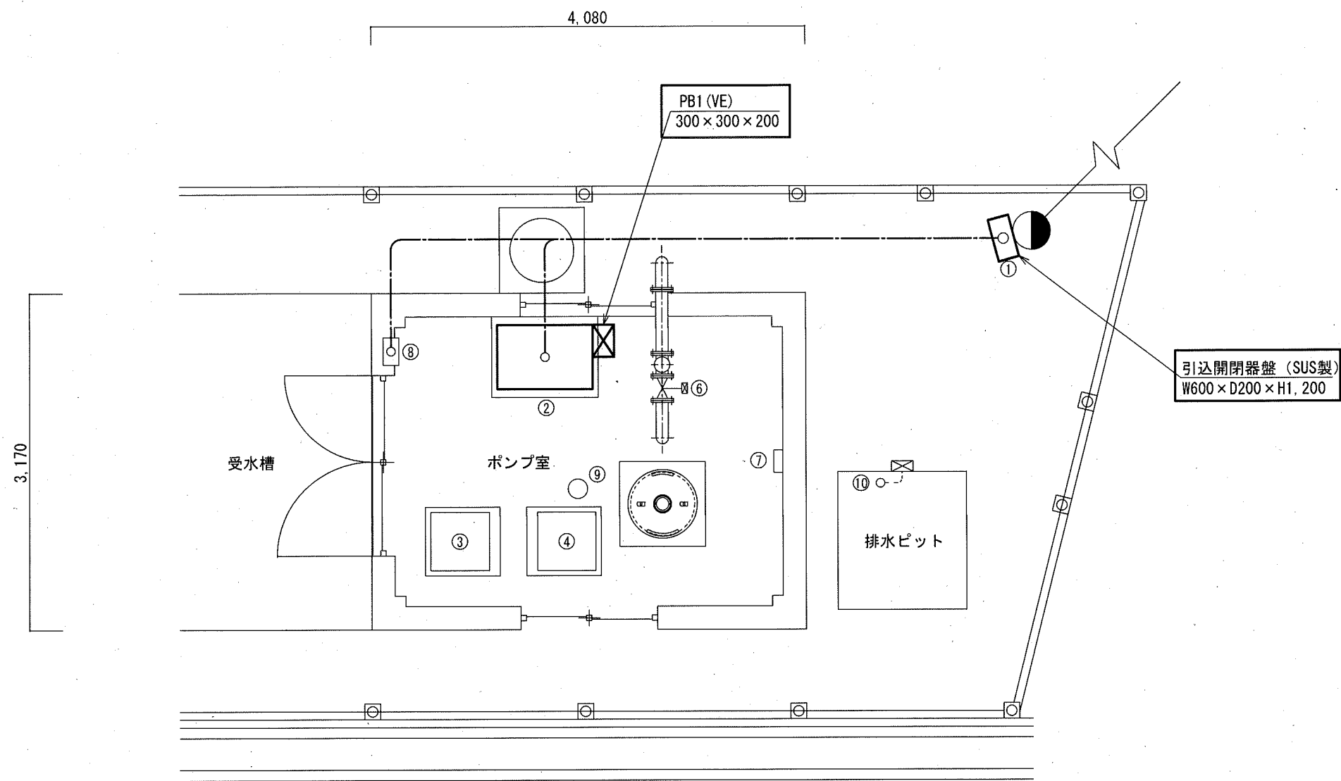
改修後平面図 (1/50)
