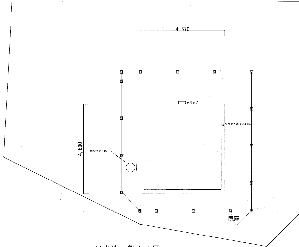
配水池一般平面図 (S=1/100)
