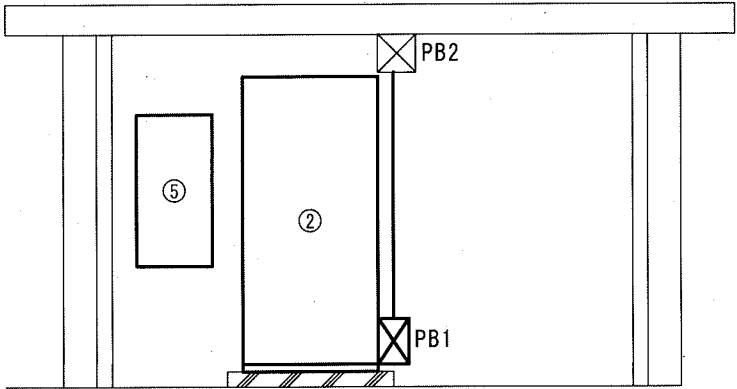
改修前断面図 (1/50)
