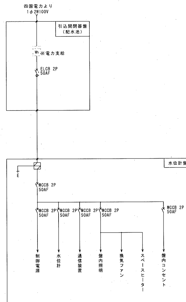
単線結線図
