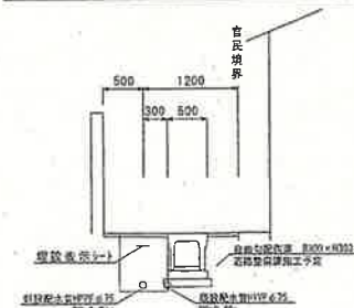
横断面図 S=1/50
