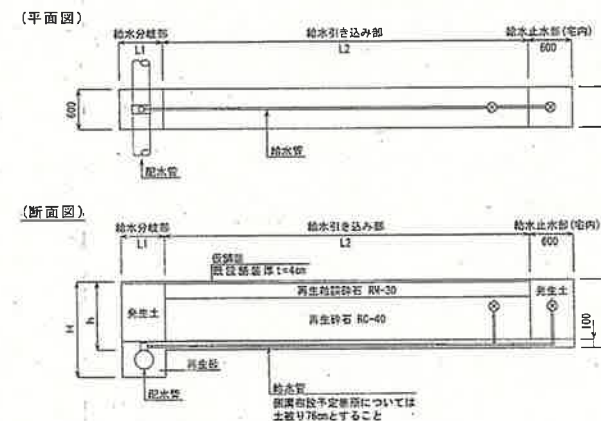
給水切替標準図 S=Free
