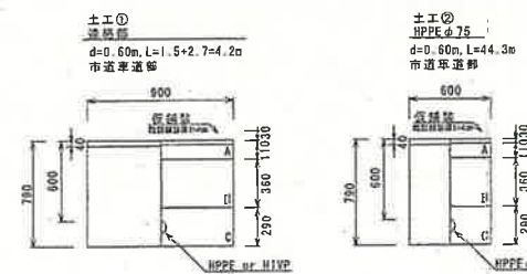
土工断面図 S=1:30
