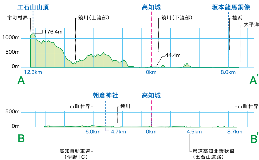
高知市地形断面図
