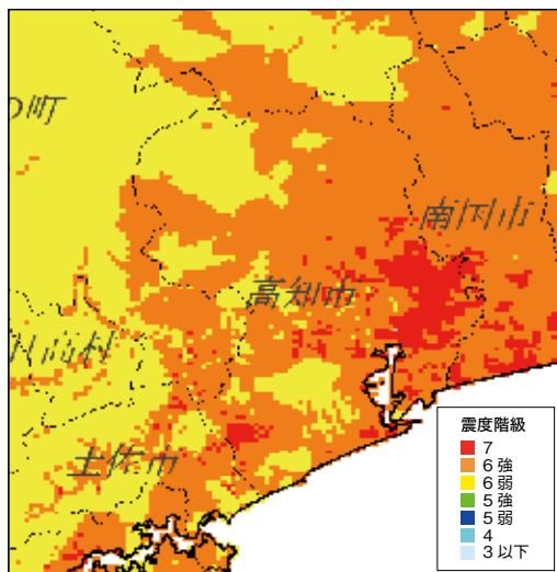
【震度分布図】
