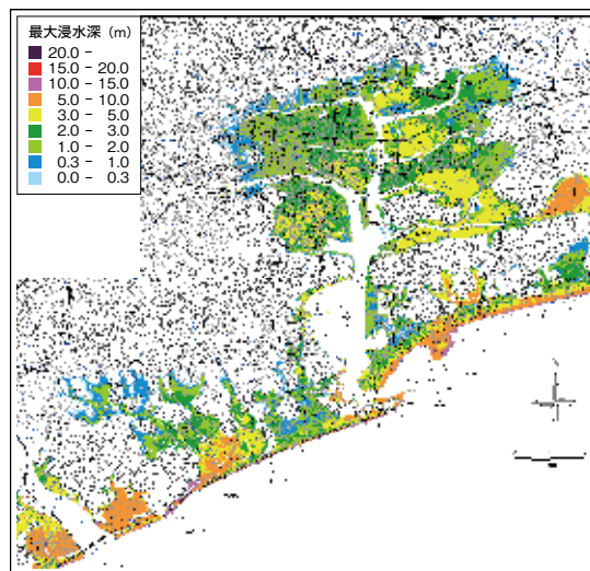
【津波浸水予測図】
