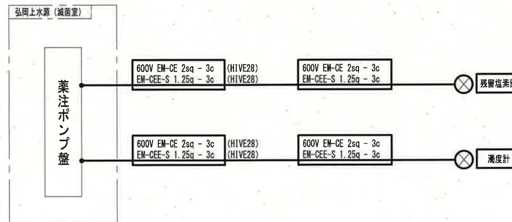
配線系統図 (更新) (S=NON)
