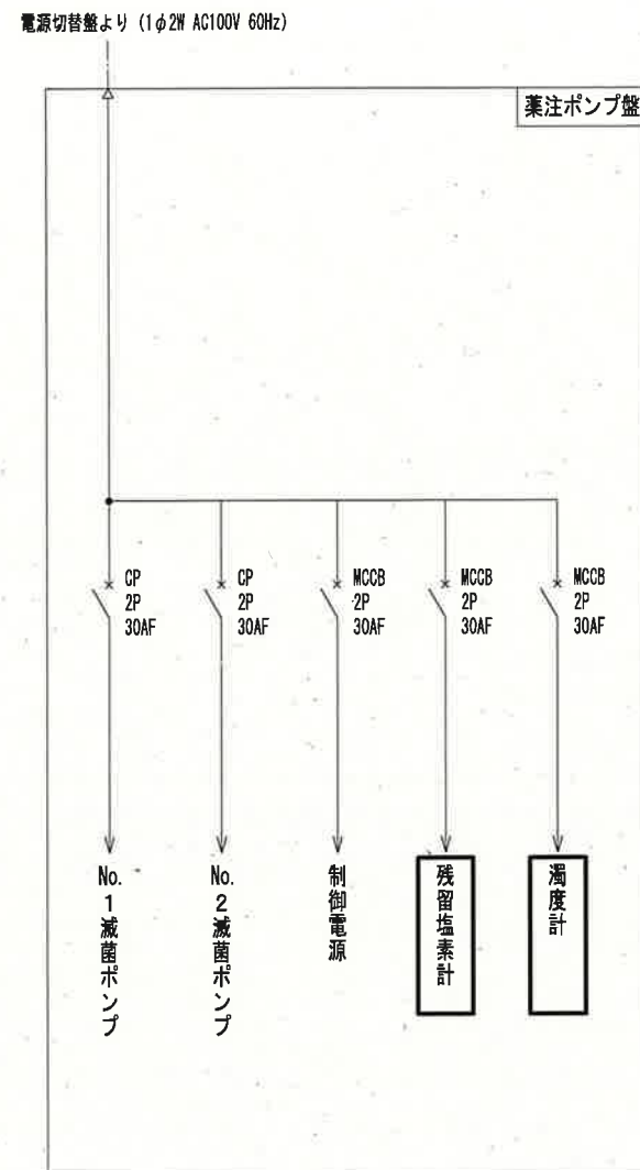
単線結線図 (薬注ポンプ盤) (S=NON)
