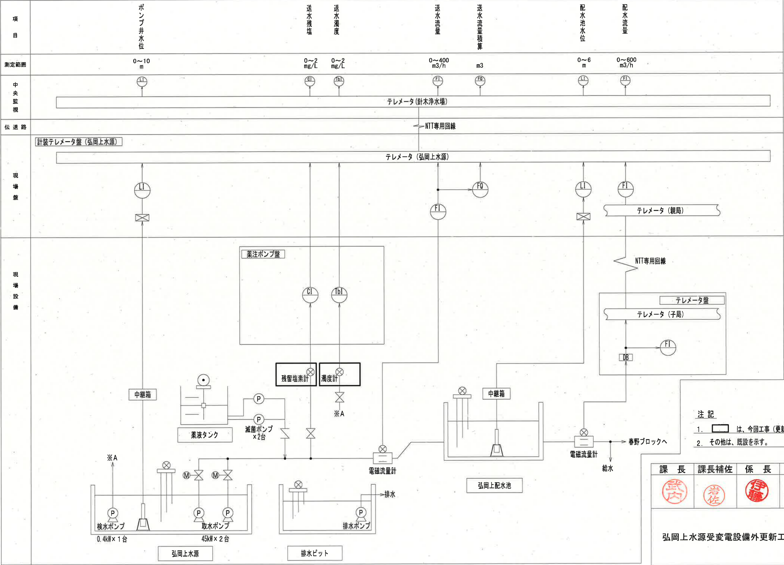
計装フローシート (S=NON)
