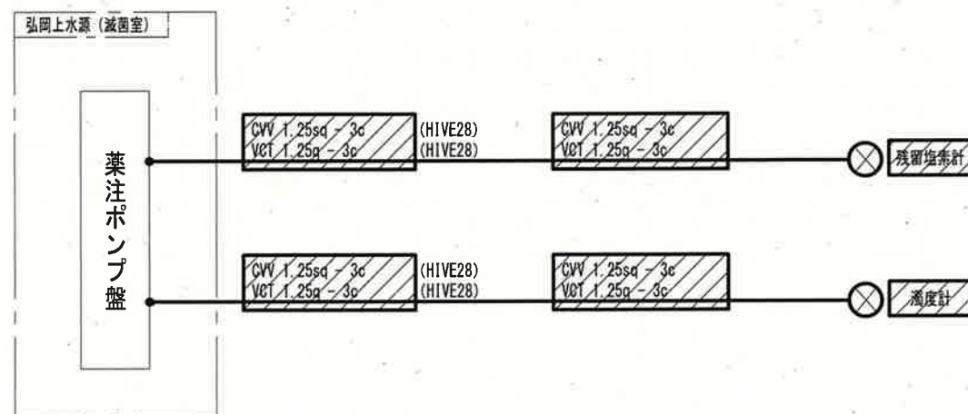
配線系統図 (撤去) (S=NON)
