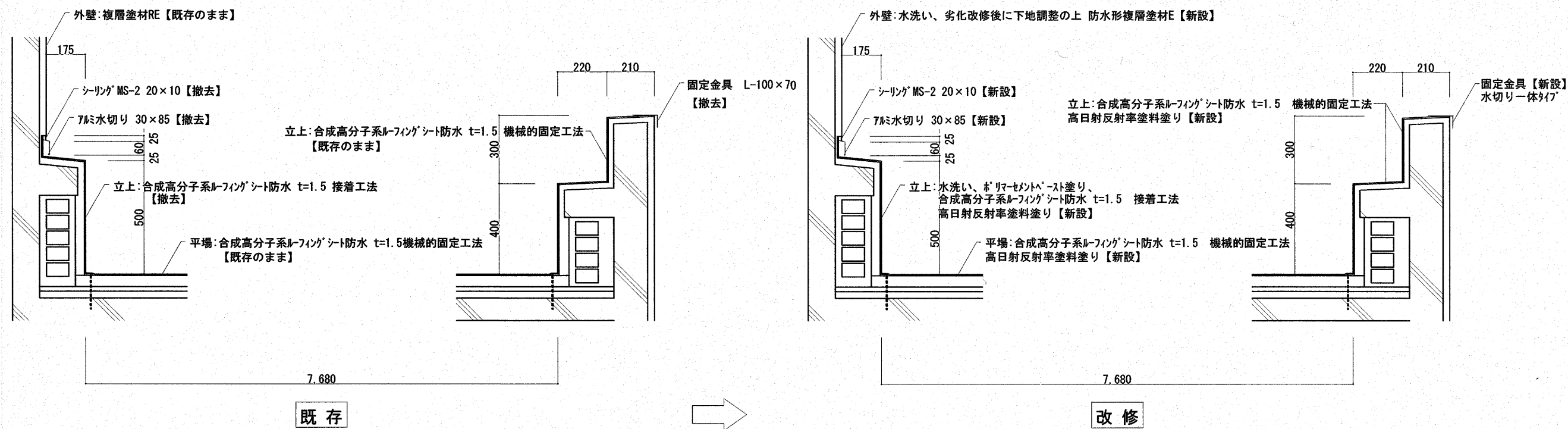
屋根 2 ② 部分詳細図 S=1:20
