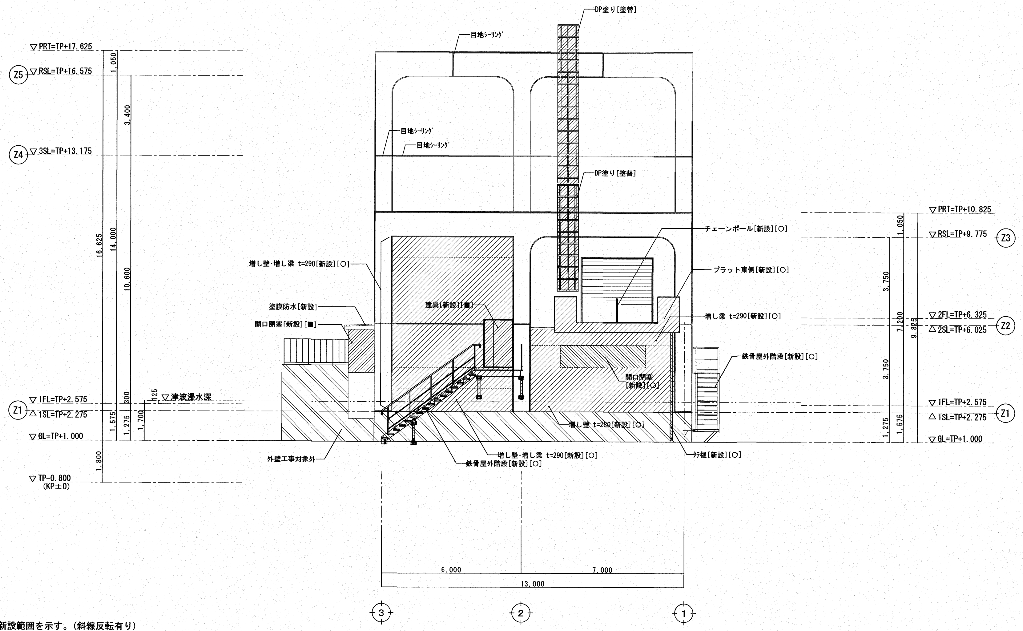
東面 立面図 [改修後]
