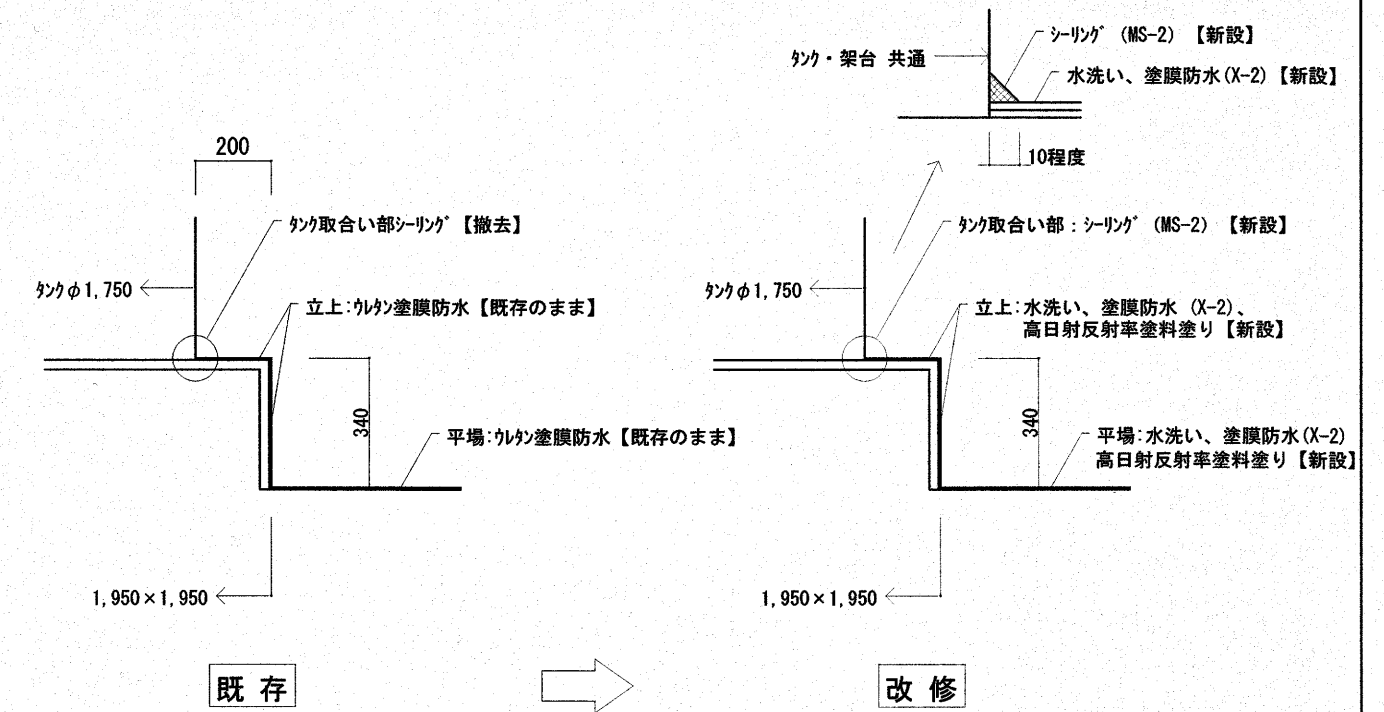
屋根 2 ③・⑩ 部分詳細図 S=NONE
