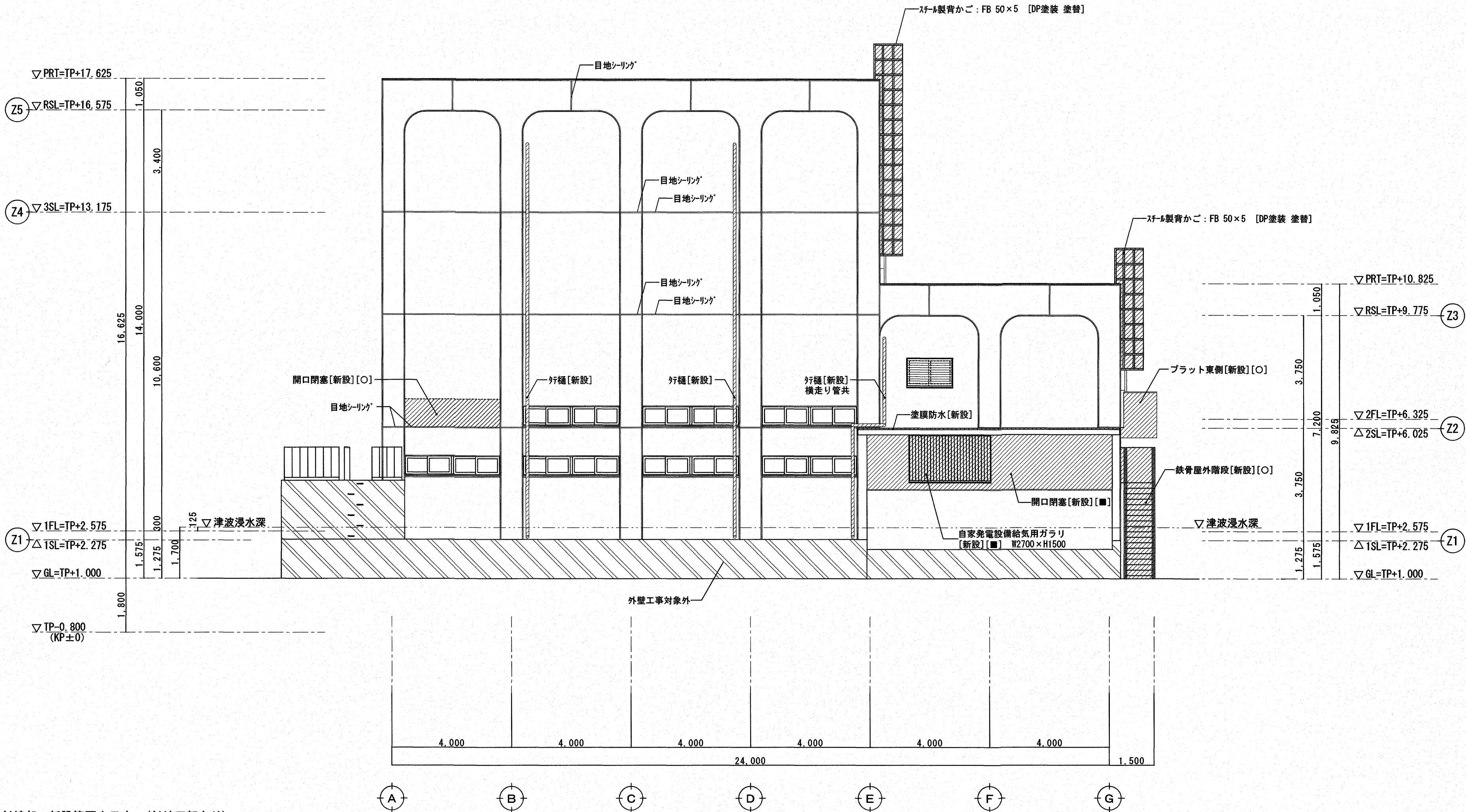
南 面 立 面 図 [ 改 修 後 ]
