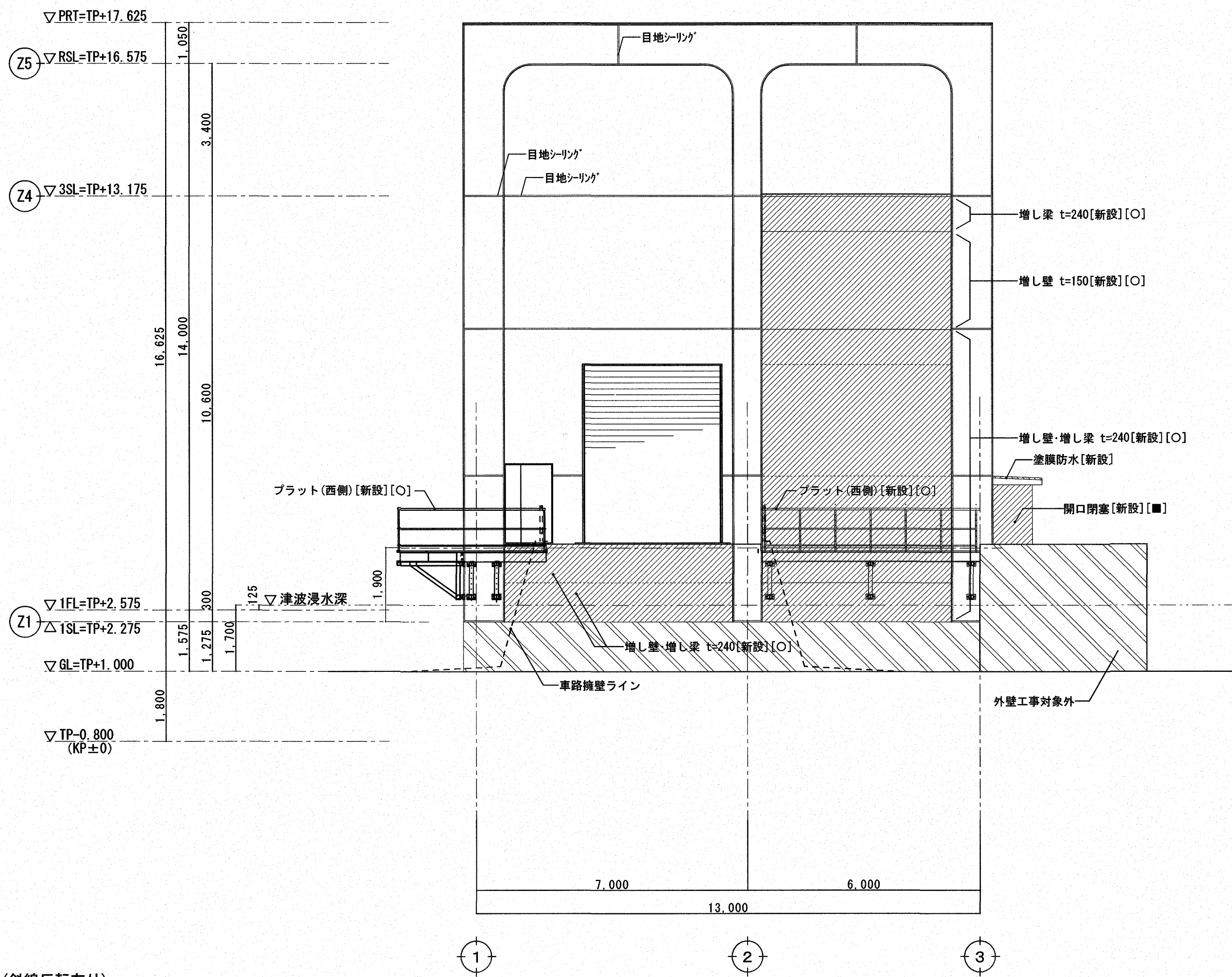
西 面 立 面 図 【 改 修 後 】
