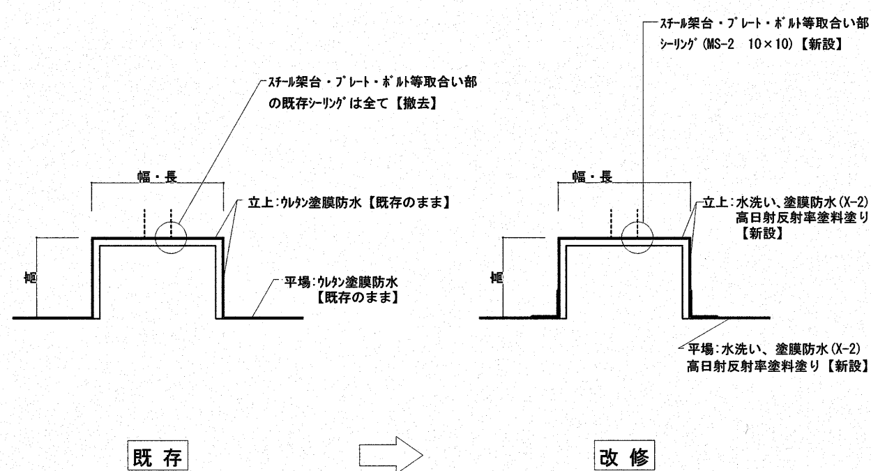
屋根 2 ④～⑨・⑪・⑫ 部分詳細図 S=NONE
