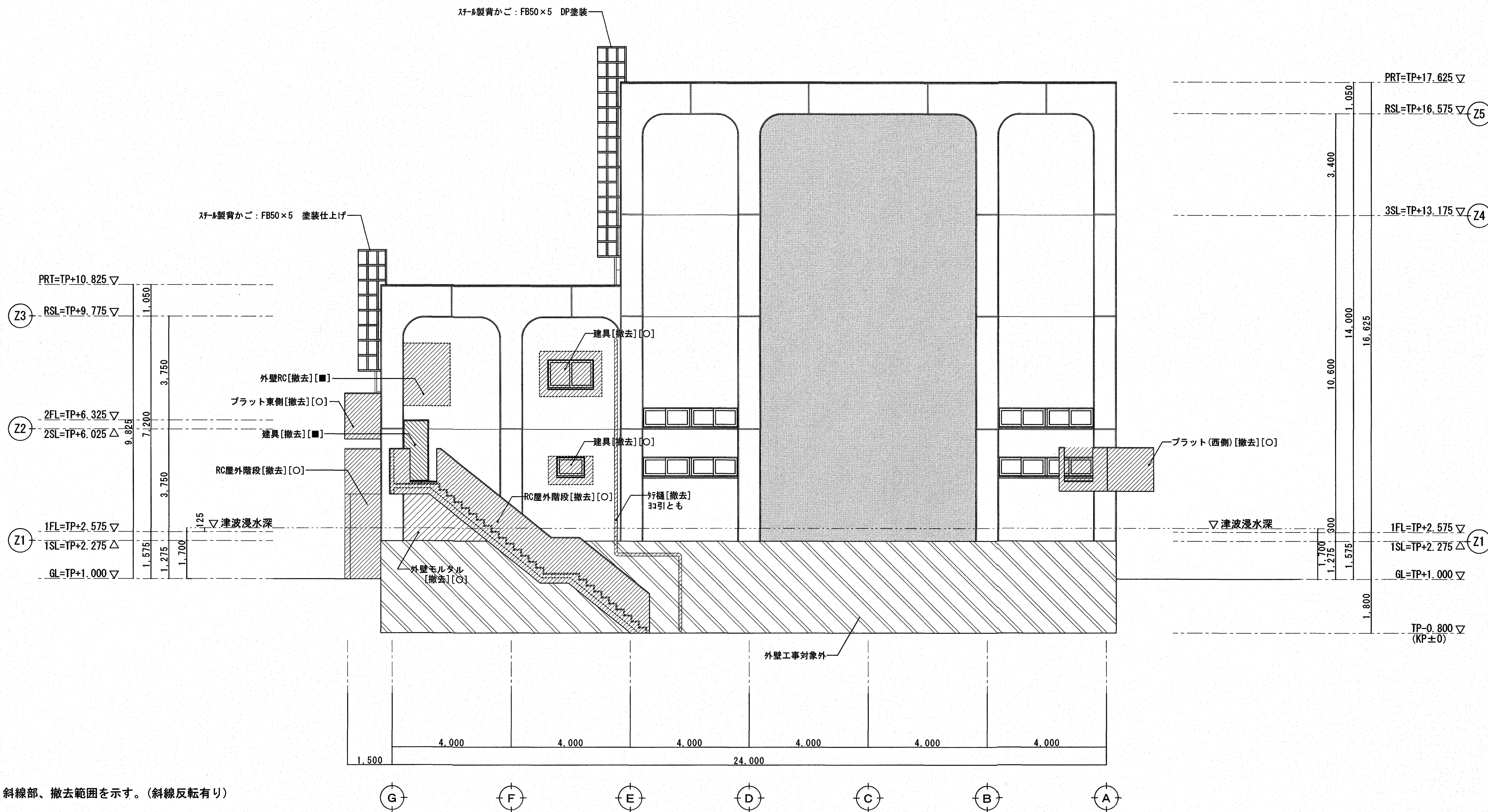
北面 立面図 [改修前]
