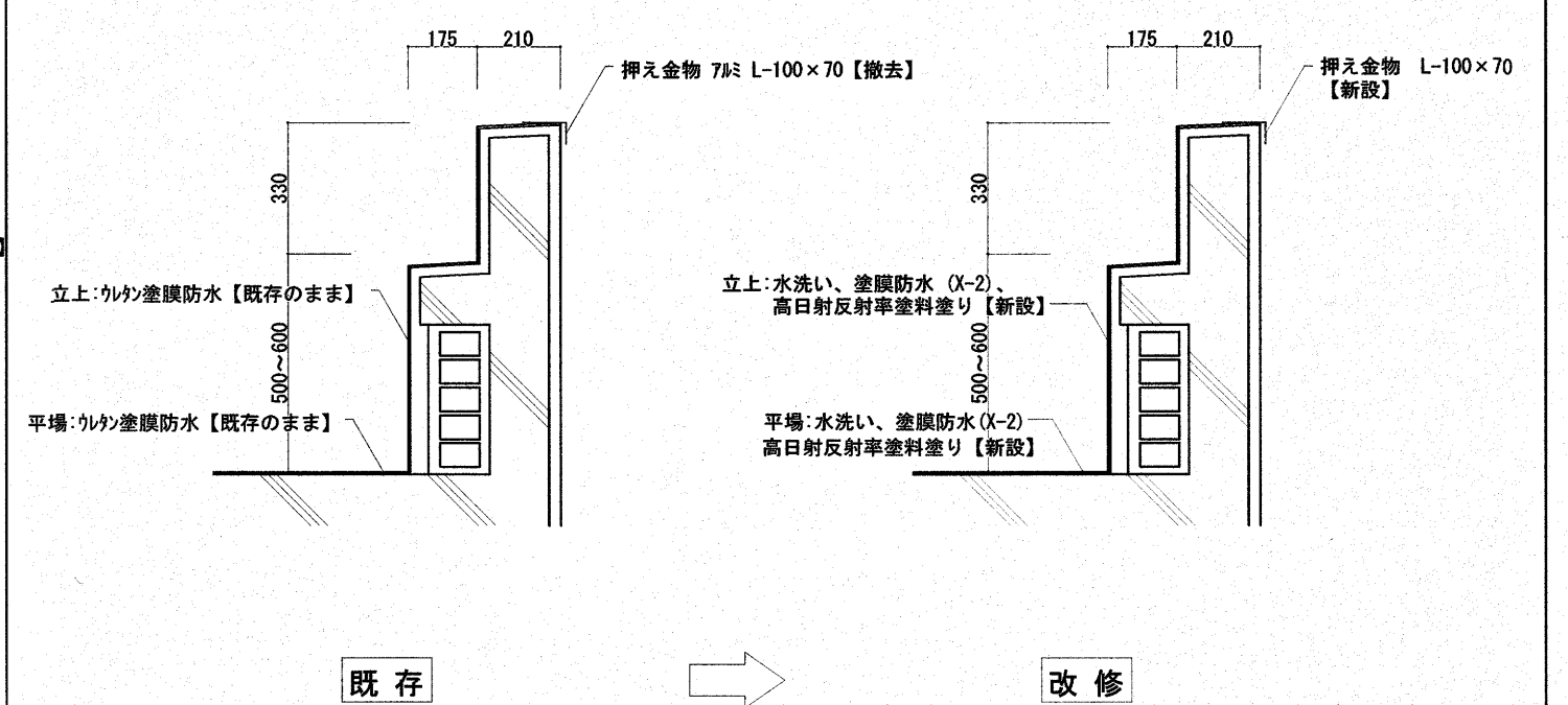
屋根 2 ハラヘツト 部分詳細図 S=1:20
