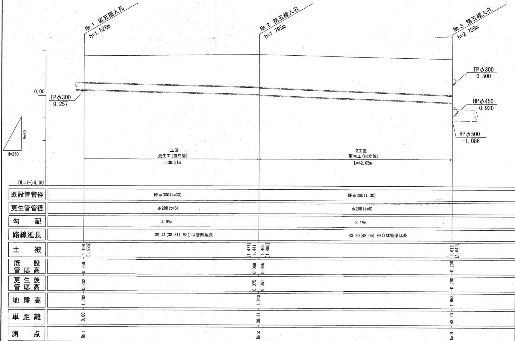
縦断図 V=1:50 H=1:250
