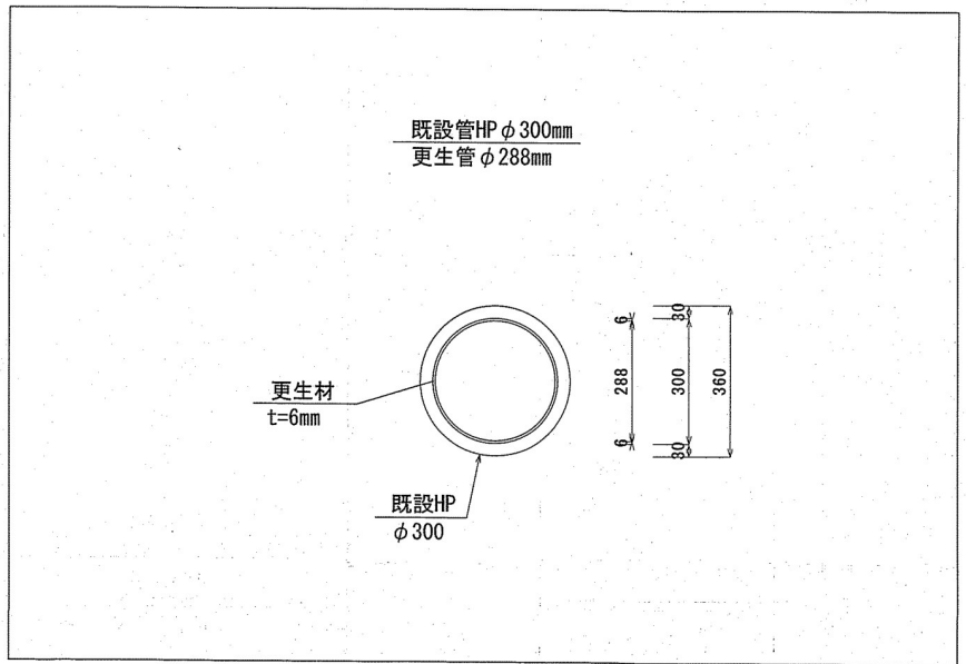
更生管詳細図(参考図) S=1:10
