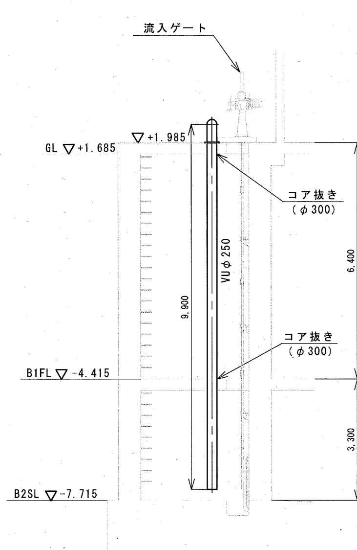
A-A 断面
