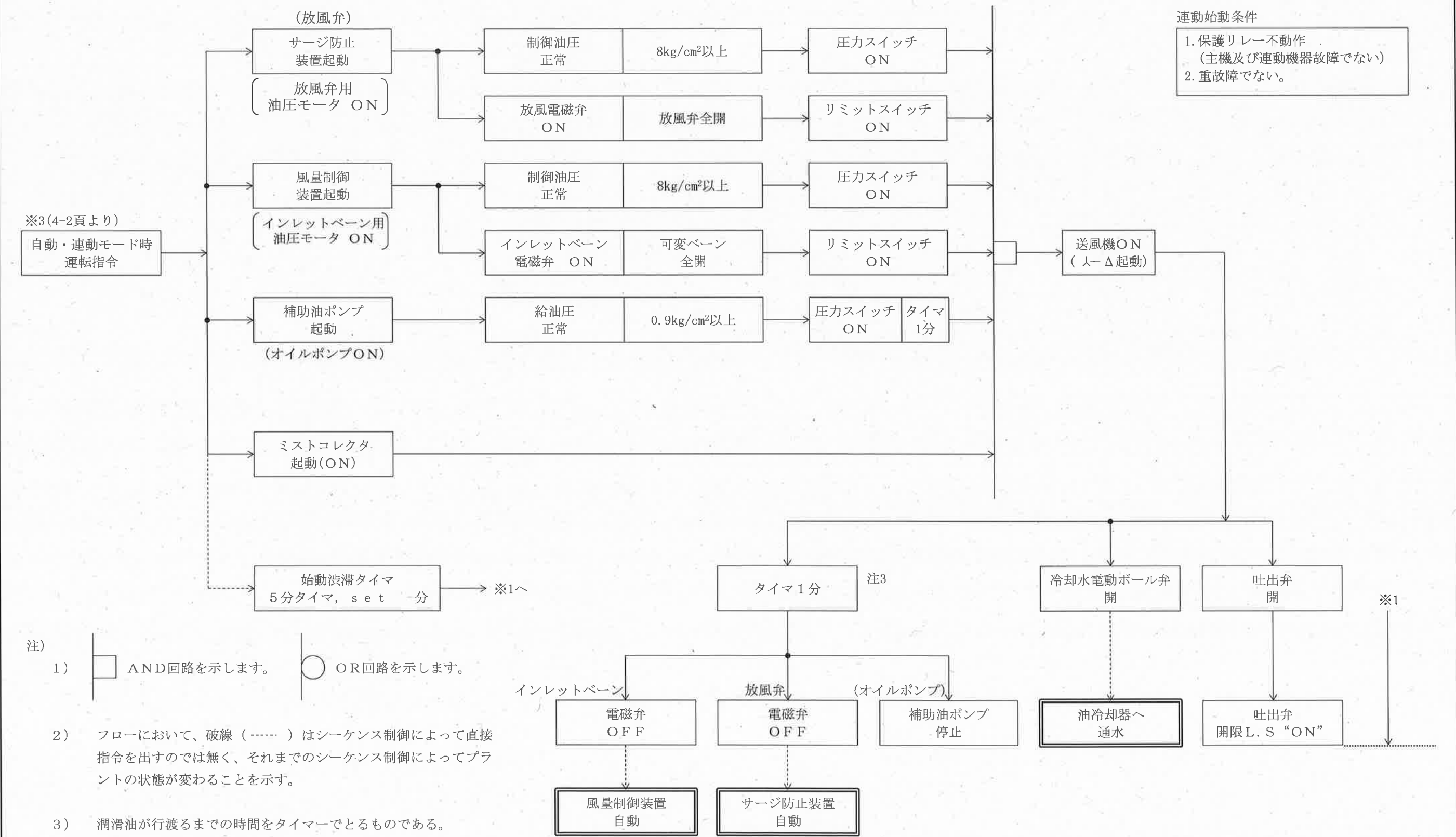
[自動・連動モード時 No.3, 4送風機フロー図(1/2)]
