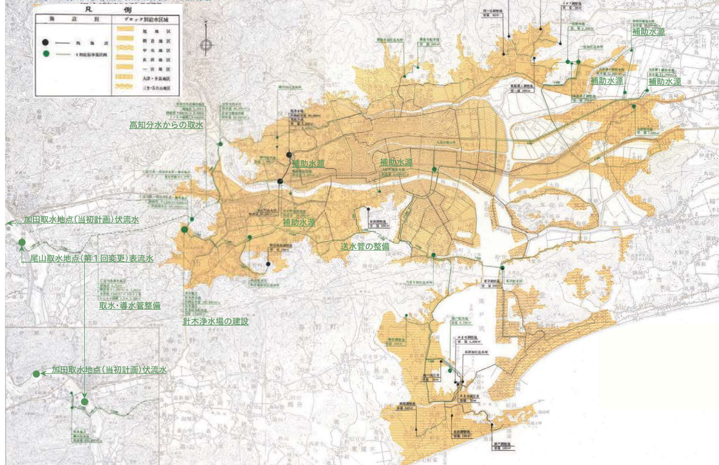
■第4期拡張事業計画概要図(第1回変更)
