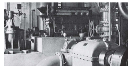
送水ポンプ（ディーゼルエンジン直結）
