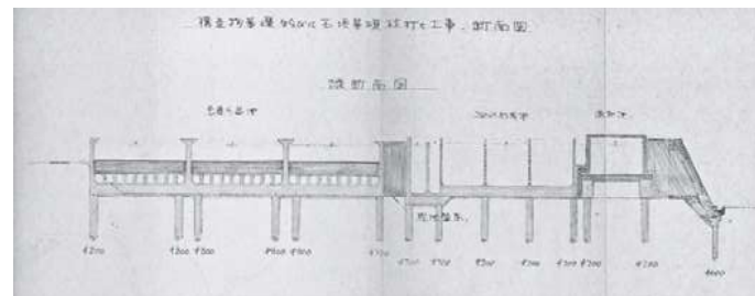
凝集池(平成17年頃)
