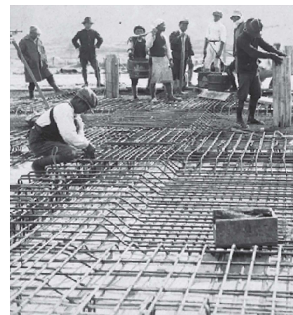
配水池での鉄筋組立作業
