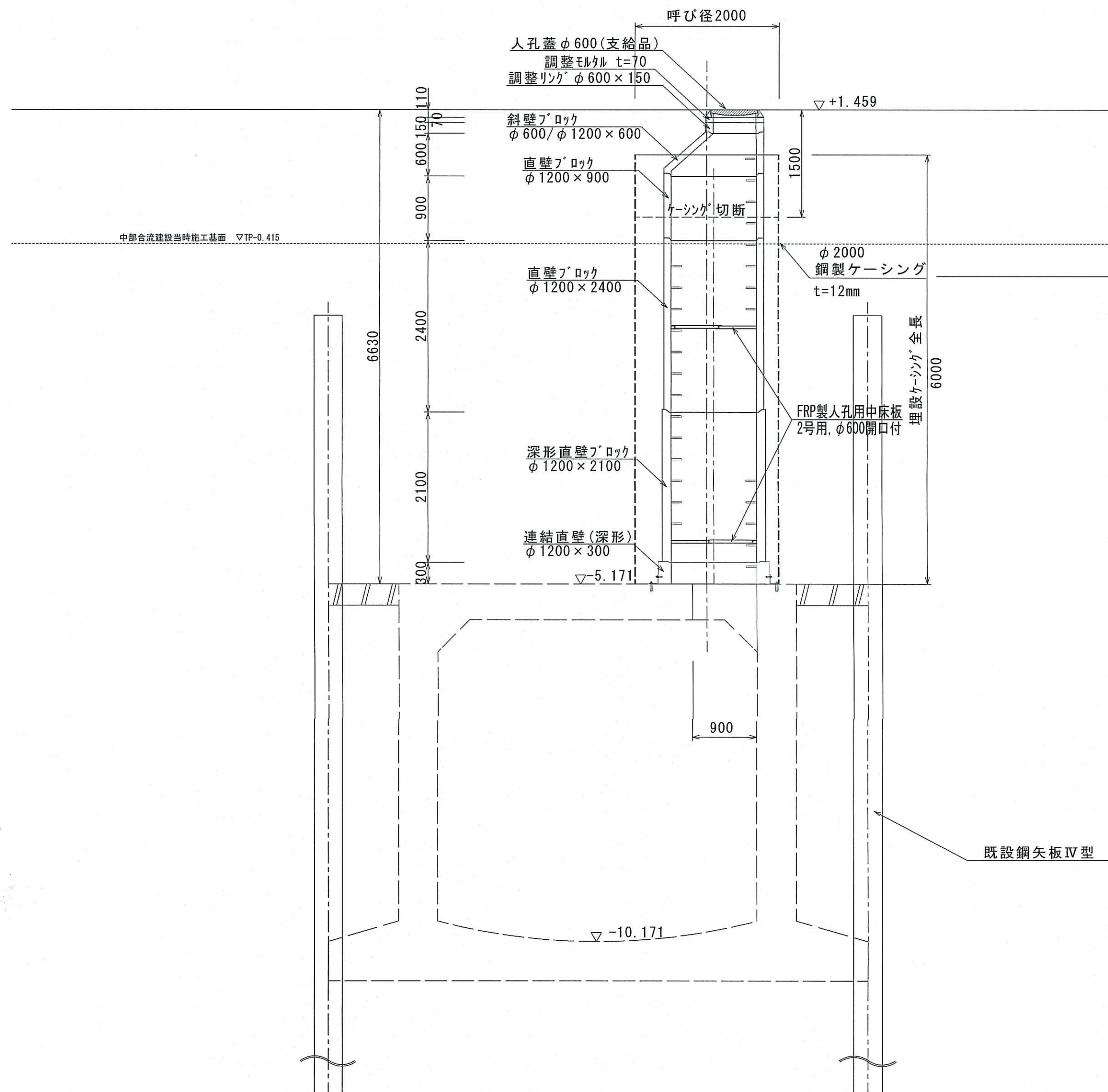
断面図
