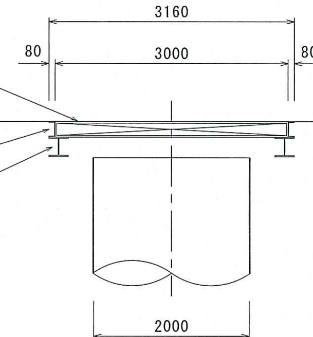
B-B 断面図
