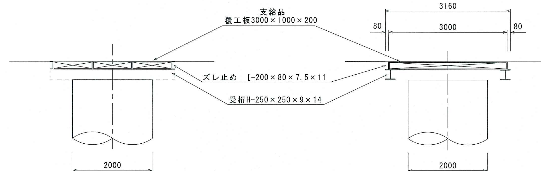
A-A 断面図
