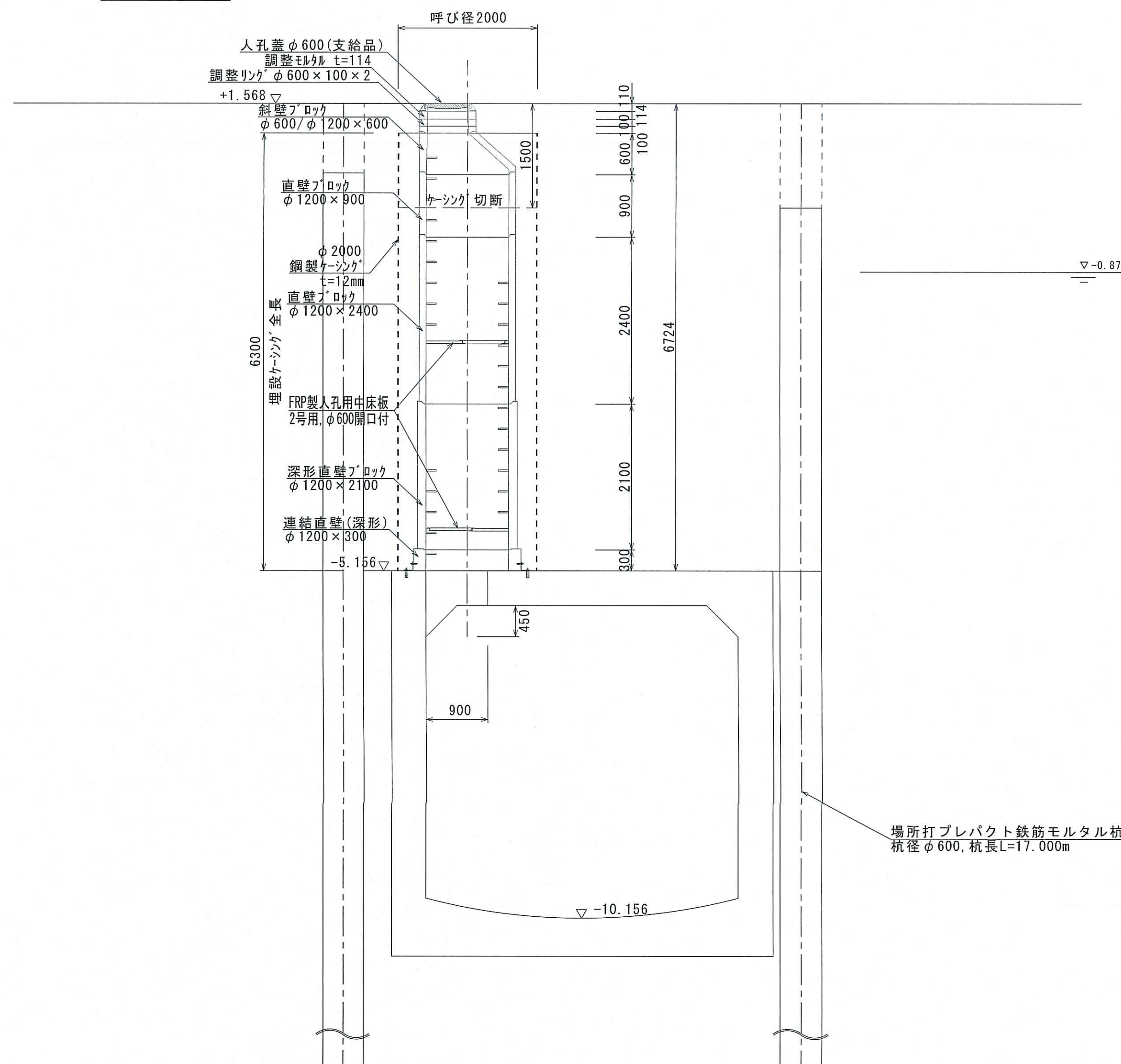
断面図
