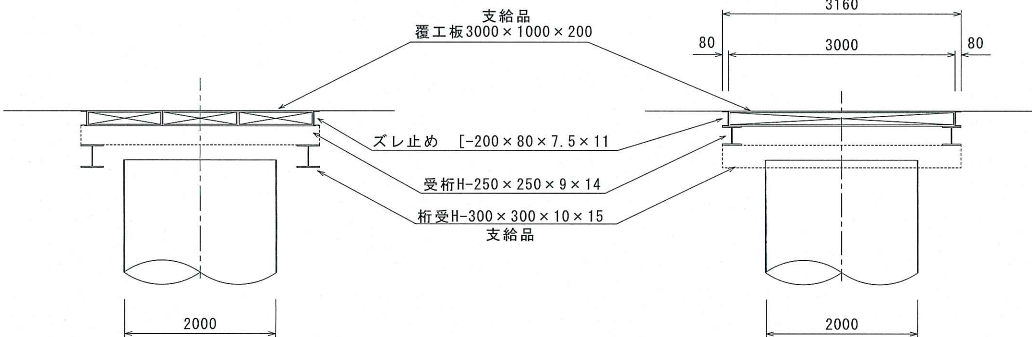
A-A 断面図
