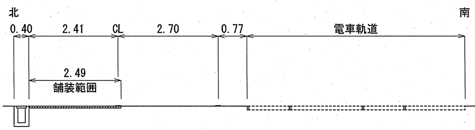
A-A' 横断面 S=1:100
