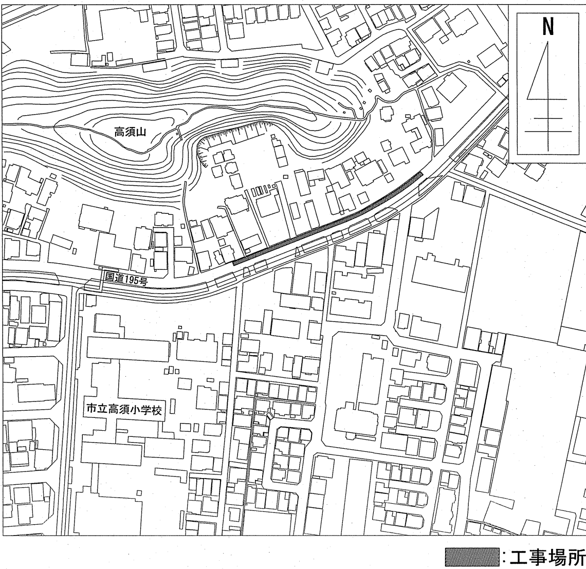
位置図 S=1:2500
