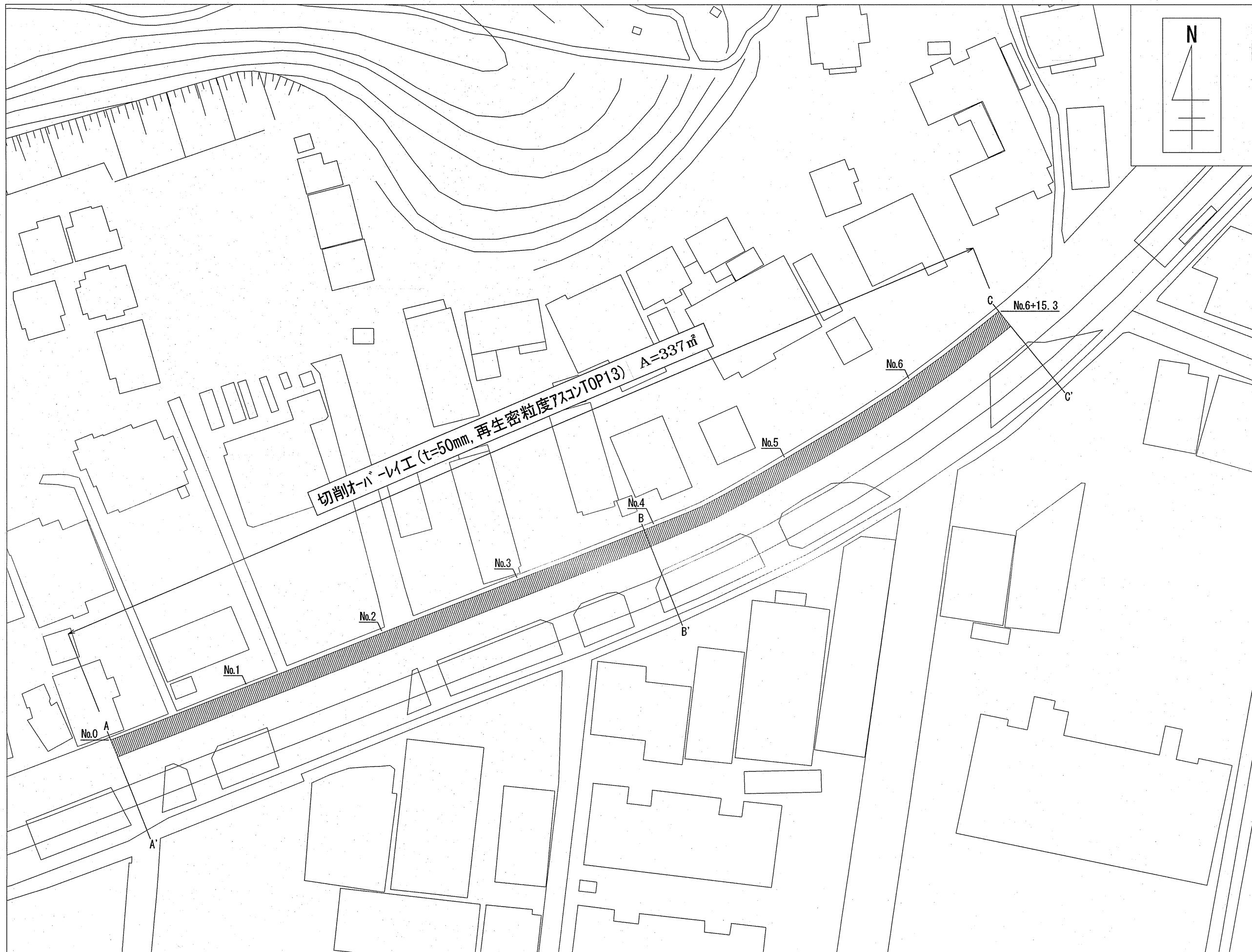
平面図 S=1:500
