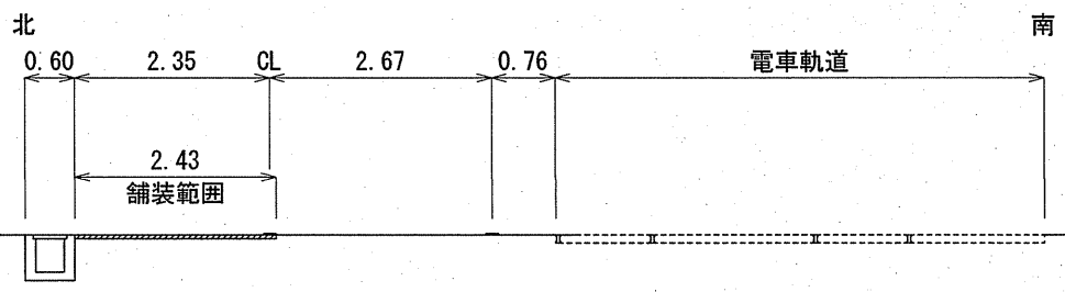
B-B' 横断面 S=1:100
