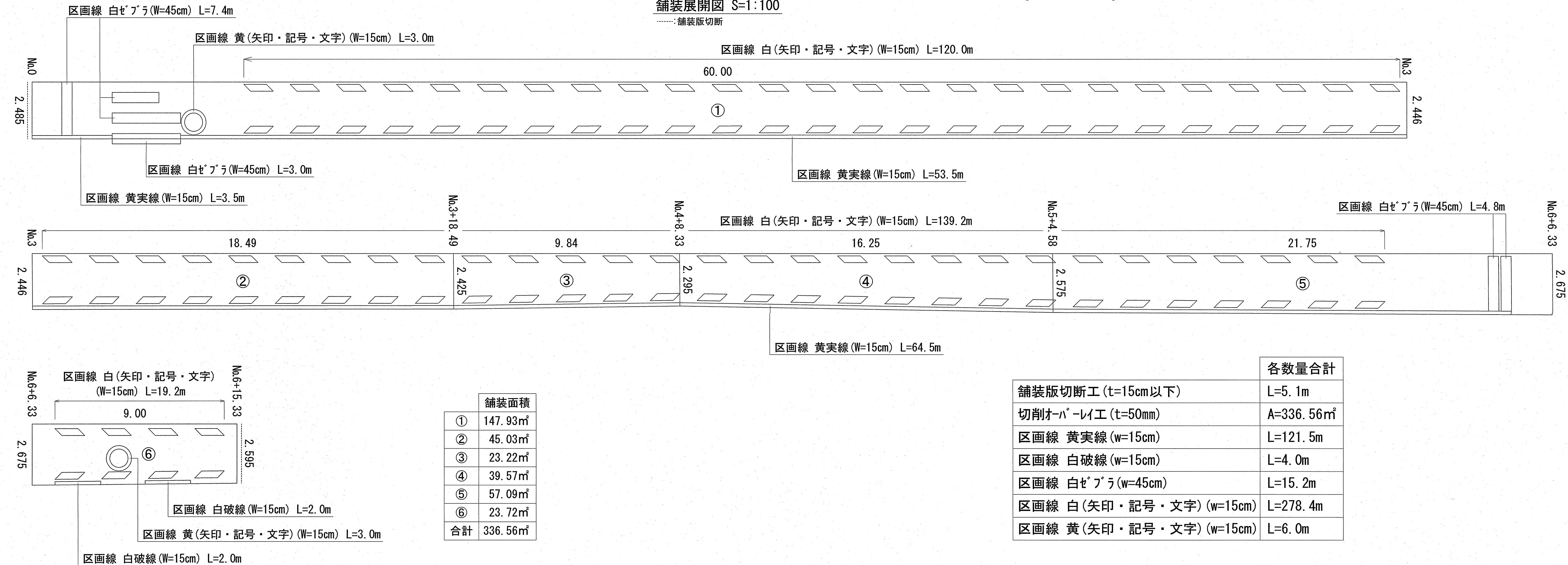
舗装展開図 S=1:100
