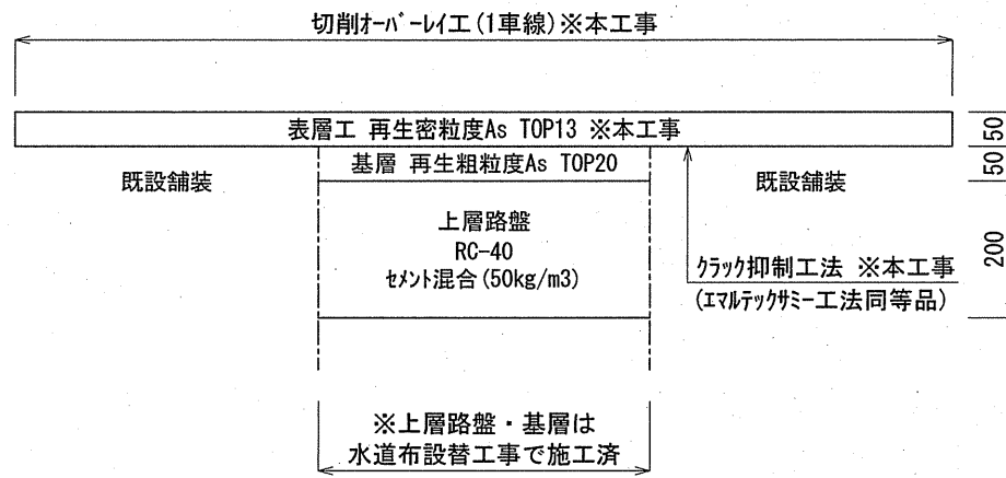
舗装構成図 S=Free
