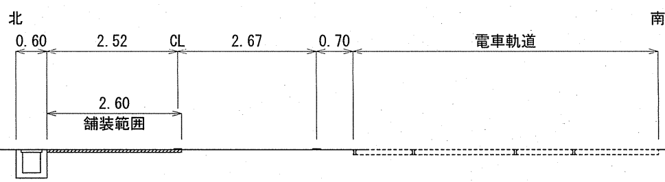
C-C' 横断面 S=1:100
