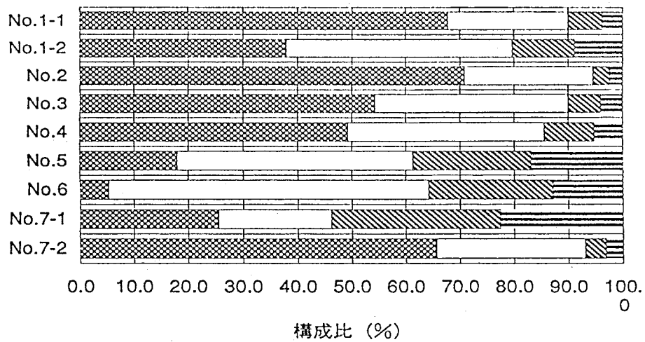
図3-2 粒度組成図
